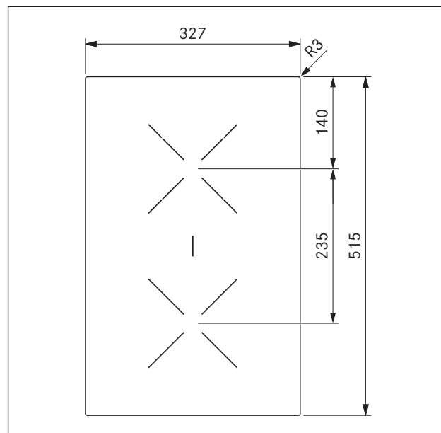
Fig. 3.17 CKCB - enhedens mål set fra oven
