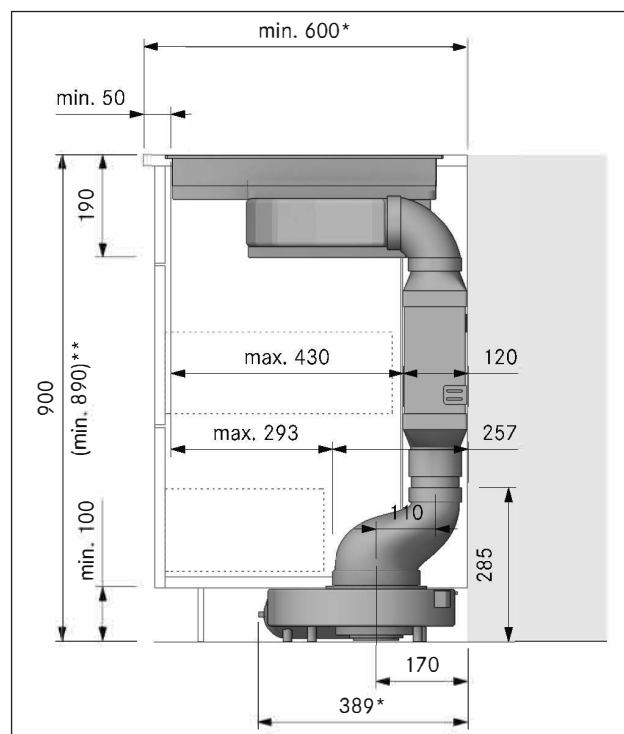
Fig. 4.16 Indbygningsmål mit Flachschalldämpfer USDF, kanalforbindelse flad EFV og overgangsstykke fladt rundt forskydning EFRV110 (køkkenelementer 600)
