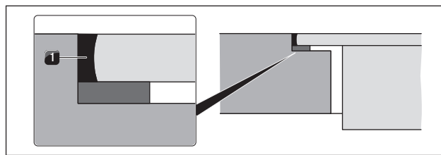
Fig. 4.49 Silikonforseglingsmasse ved planlimet montering
