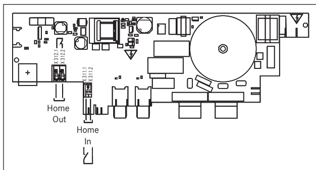
Fig. 4.35 Tilslutningsskema til eksterne afbryderkontakter
