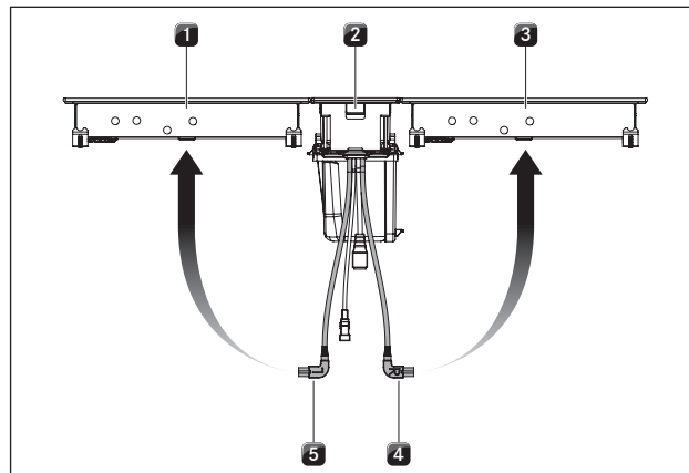
Fig. 4.39 Tilslutning af styrekabler til kogepladen
