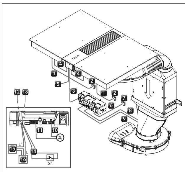
Fig. 4.38 Tilslutningsdiagram for kogepladeemfang CKA2/CKA2AB
