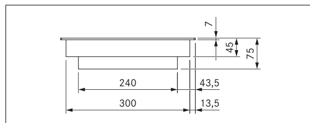
Fig. 3.18 CKCB - enhedens mål set forfra
