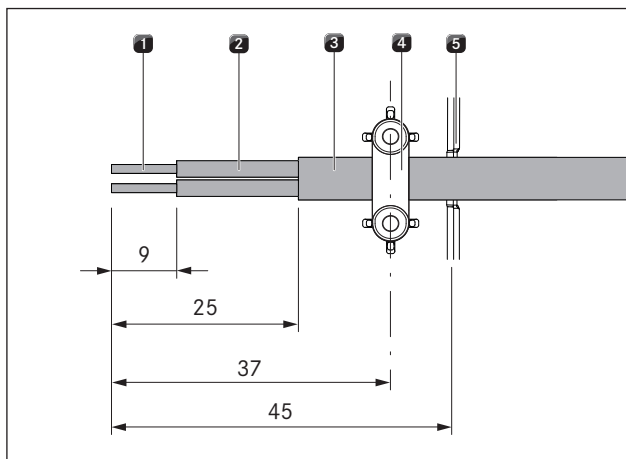
Fig. 4.34 Afisoleringslængder og monteringsposition for tilslutningskablet
