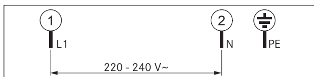
Fig. 4.44 Tilslutningsskema, 1-faset tilslutning kogeplade
