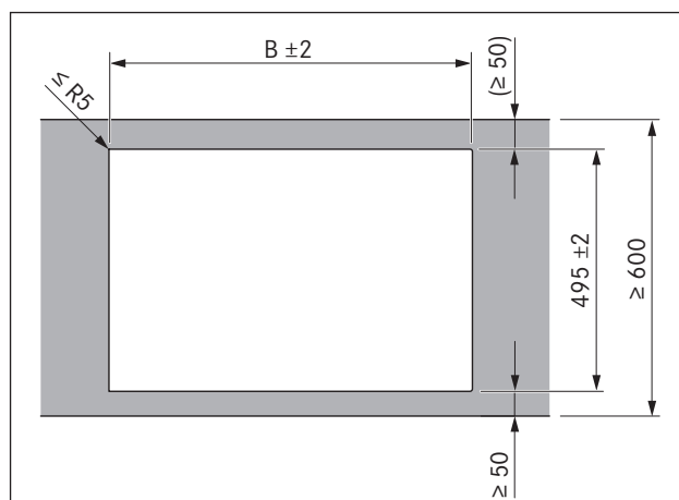
Fig. 4.12 Udkæringsmål til overflademontering
