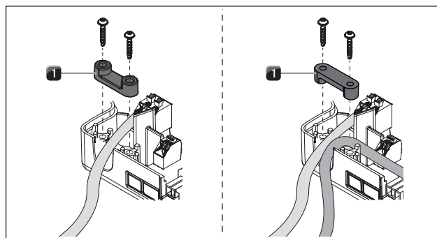
Fig. 4.37 Montering af trækaflastningsklemme
