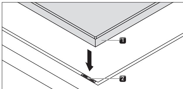
Fig. 4.29 Kogeplade og højdeudligningsplader
