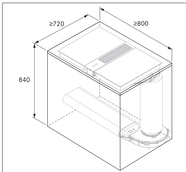
Fig. 4.15 Mindstemål for indbygning med rund lyddæmper USDR50
