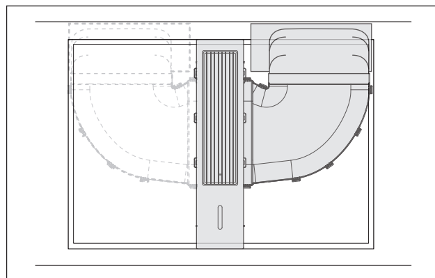
Fig. 4.19 Luftkanal på bagsiden (højre eller venstre)
