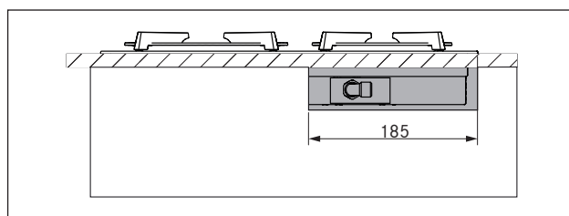
Fig. 4.8 Sideudskæring til gastilslutning
