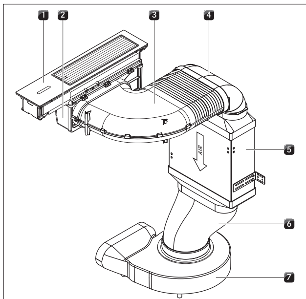
Fig. 4.27 Standardmontering af kogepladeemfang CKA2/CKA2AB
