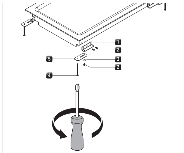
Fig. 4.32 Fastgøring af Tepan-grill i rustfrit stål
