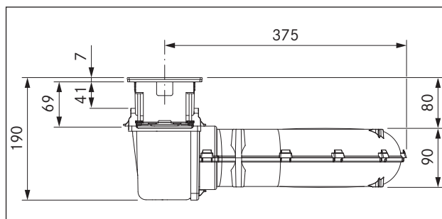
Fig. 3.2 CKA2/CKA2AB - enhedens mål set forfra
