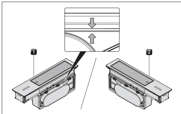
Fig. 4.21 Monteret kogepladeemfang CKA2/CKA2AB
