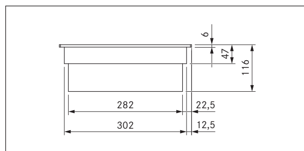
Fig. 3.12 CKIW - enhedens mål set forfra
