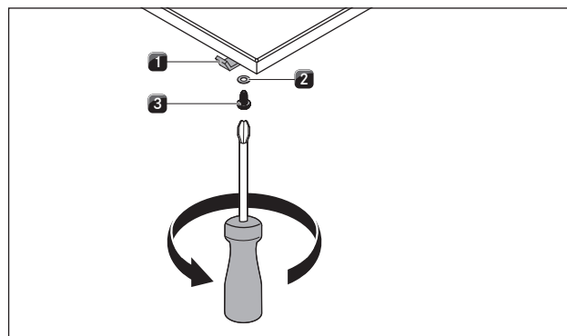
Fig. 4.31 Fastgøring af kogepladen
