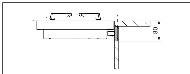
Fig. 4.9 Sideudskæring til gastilslutning (set forfra)
