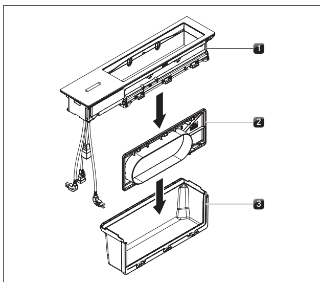
Fig. 4.22 Montering af de enkelte komponenter i kogepladeemfanget CKA2/CKA2AB
