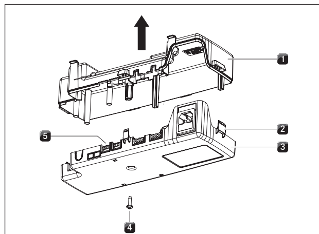
Fig. 4.33 Åbn dækslet på styreenheden
