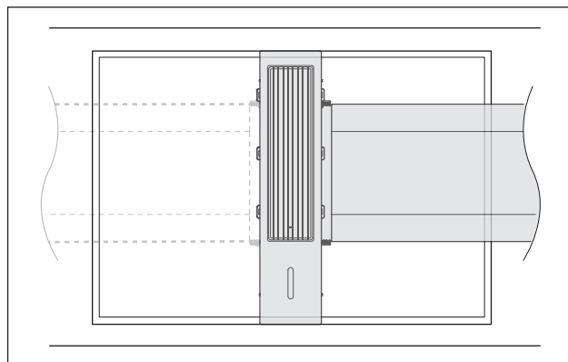
Fig. 4.20 Lige luftkanal på siden (højre eller venstre)
