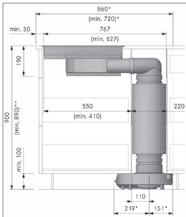
Fig. 4.18 Indbygningsmål med rund lyddæmper USDR50 og kanalforbindelse rund ERV (køkkenøer)
