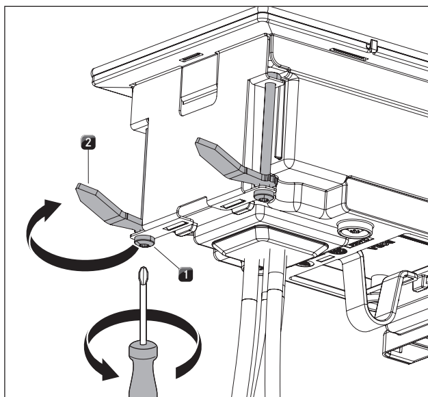
Fig. 4.30 Fastmontering af emfanget
