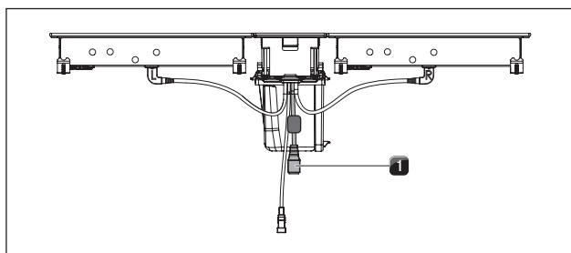
Fig. 4.41 Tilslutningsbøsning til kommunikationskablet CAT 5e på styreenheden
