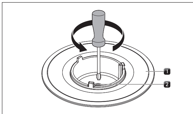
Fig. 4.47 Kogezone-brænder med gas-brænderdyse
