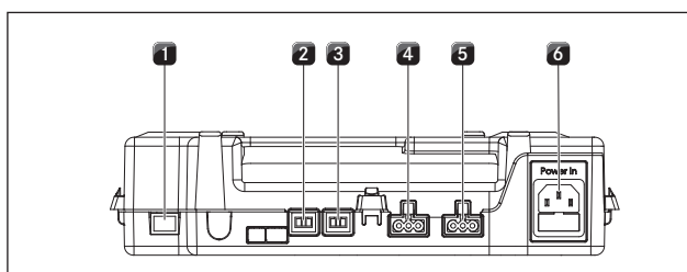
Fig. 4.42 Tilslutninger til styreenheder
