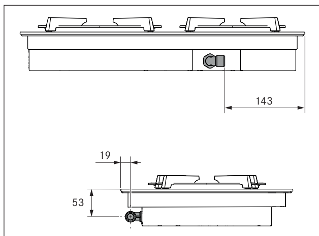
Fig. 4.45 Placering af gastilslutning
