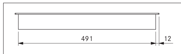
Fig. 3.7 CKFI - enhedens mål set fra siden
