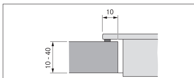
Fig. 4.13 Monteringsmål ved overflademontering
