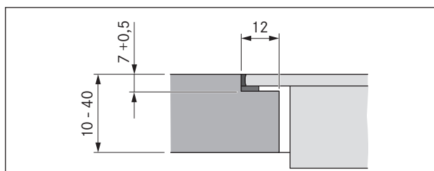
Fig. 4.11 Falsmål til planimet montering
