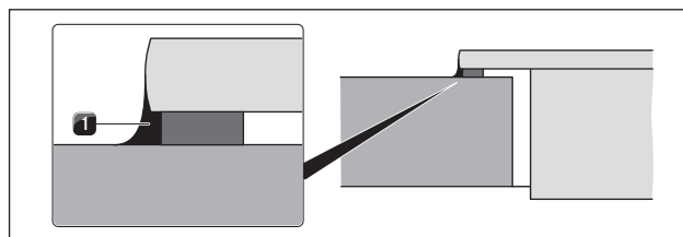
Fig. 4.50 Silikonmasse ved overflademontering
