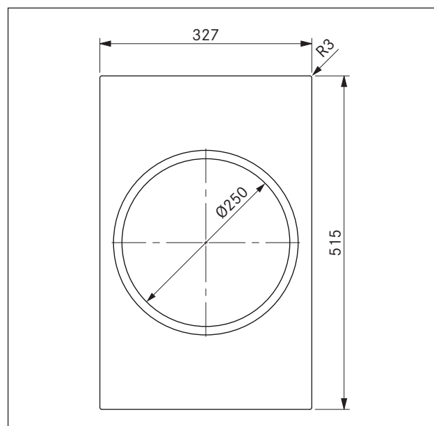
Fig. 3.11 CKIW - enhedens mål set fra oven
