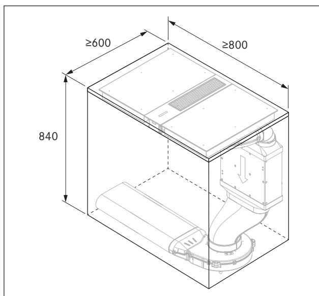
Fig. 4.14 Mindstemål for indbygning med flad lyddæmper USDF
