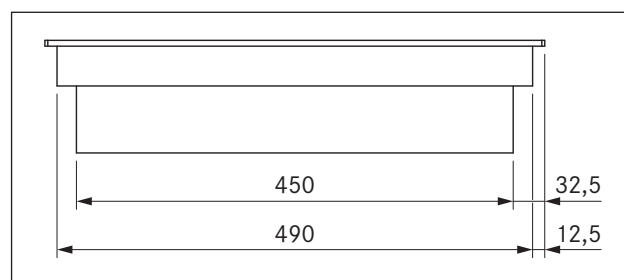
Fig. 3.13 CKIW - enhedens mål set fra siden
