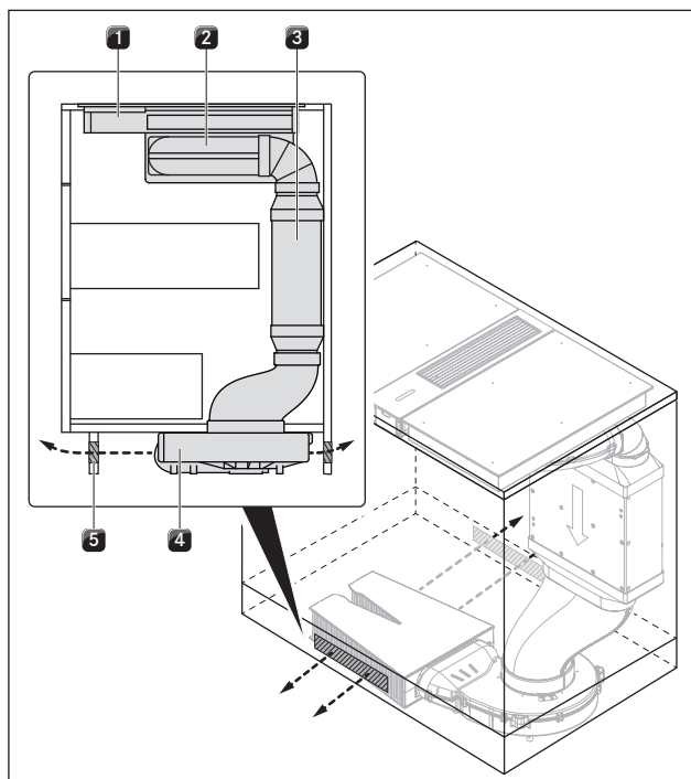
Fig. 4.4 Planlægningseksempel for recirkulationsluft (køkkenø + Kogeplade + CKA2/CKA2AB + luftrensingsenhed)
