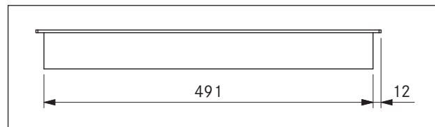
Fig. 3.10 CKI - enhedens mål set fra siden
