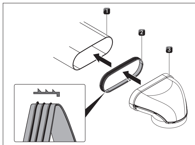
Fig. 4.26 Samling af kanalsystemet
