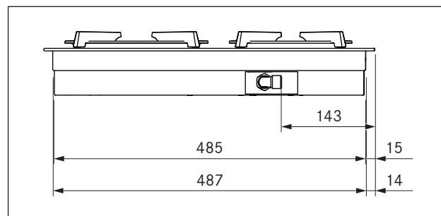
Fig. 3.22 CKG - enhedens mål set fra siden
