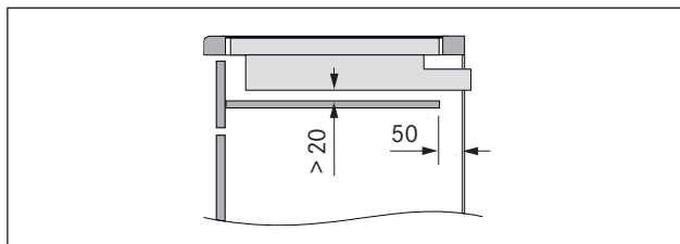
Kuva 5.2 Johdonsuojan ja tuuletuksen sivukuva
