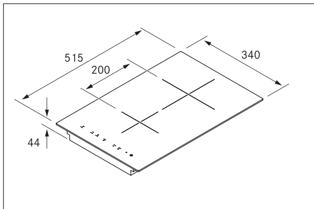
Kuva 3.1 Laitemitat
