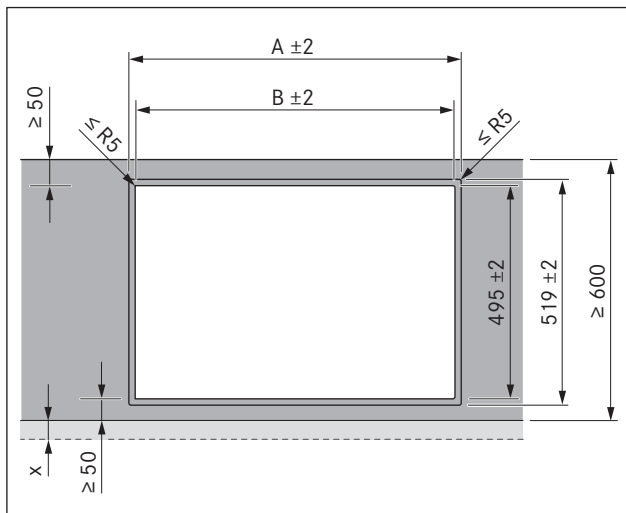
Abb. 5.3 Flächenbündige Montage
