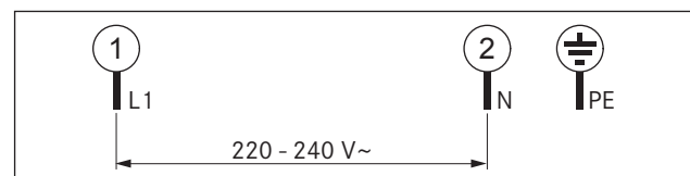
Abb. 5.12 Anschlussschema einphasig
