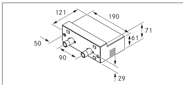
Fig. 3.2 Dimensioni quadro elettrico
