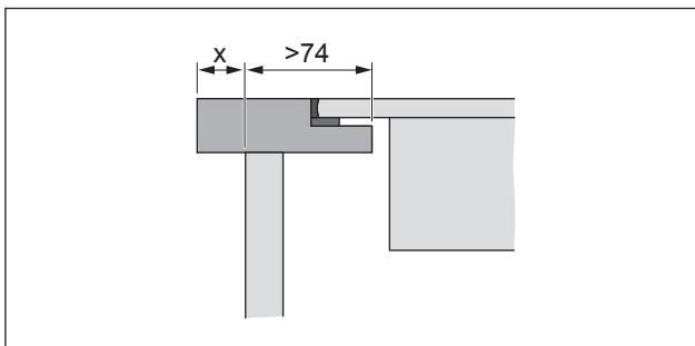
Fig. 5.2 Saliente de la encimera
