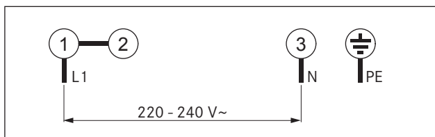
Fig. 5.18 Esquema de conexión monofásica
