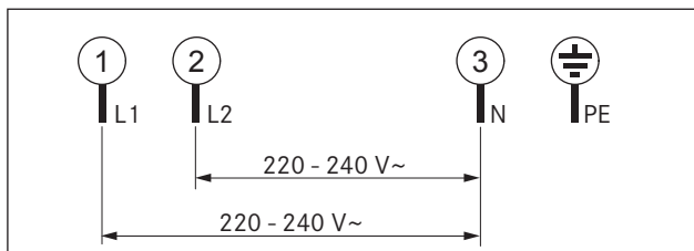
Fig. 5.17 Esquema de conexión bifásica
