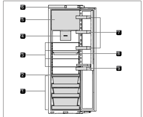
Afb. 5.2 Opbouw C178KGF
