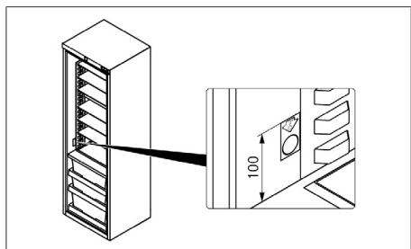
Afb. 8.16 Temperatuurindicator plaatsen
