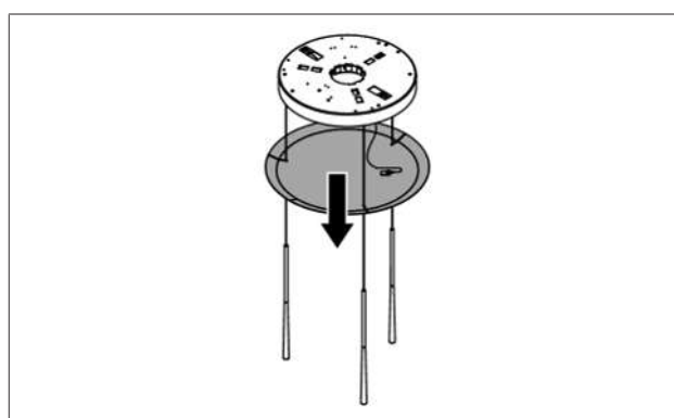
Rys. 5.4 Usuwanie pokrywy
