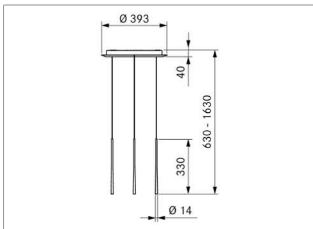
Rys. 3.1 Wymiary urządzenia
