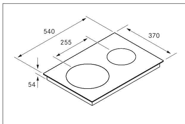
bild 3.1 Apparats mått
