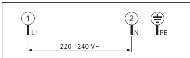
bild 5.17 Anslutningsschema 1-fasigt
