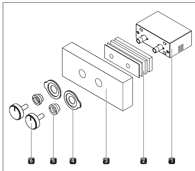
Kuva 5.9 Säätyksikön rakenne
