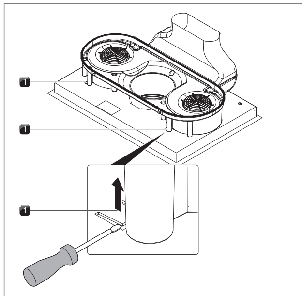
Fig. 6.32 Imobilização da posição
