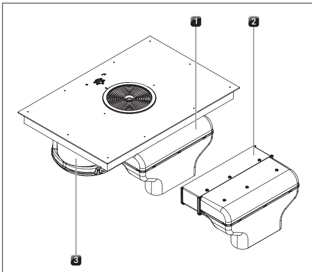
Fig. 5.3 Extrator de superfície com extração de ar (BFIA)
