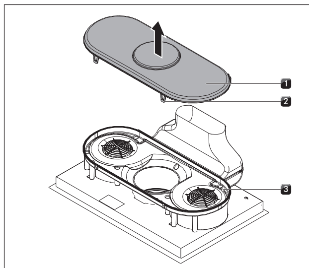
Fig. 6.24 Retirar o fundo da carcaça
