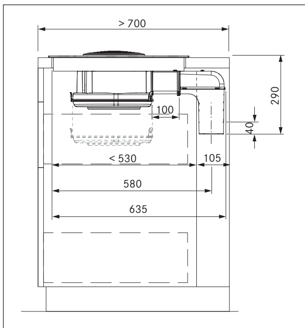
Fig. 6.23 Medidas de montagem com extração de ar, profundidade da bancada a partir de 700 mm
