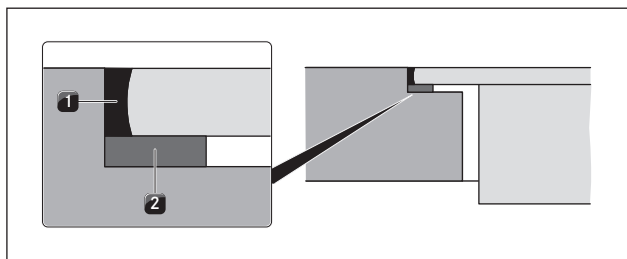
Fig. 6.8 Cinta vedante na montagem à face
