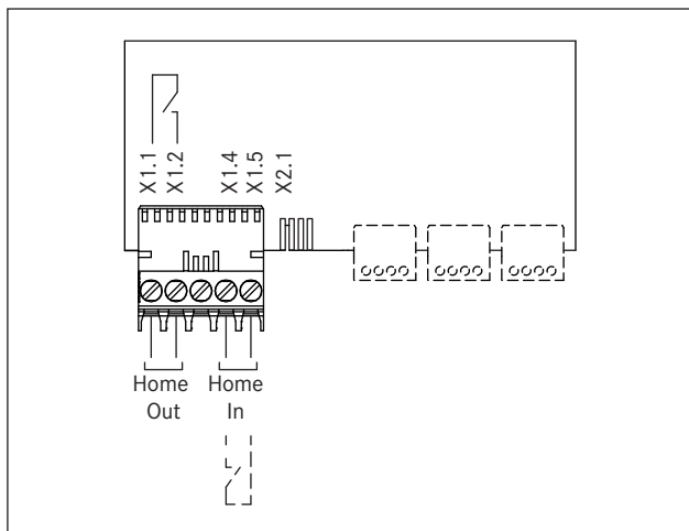
Fig. 6.42 Esquema de ligações dos contactos de corte externos
