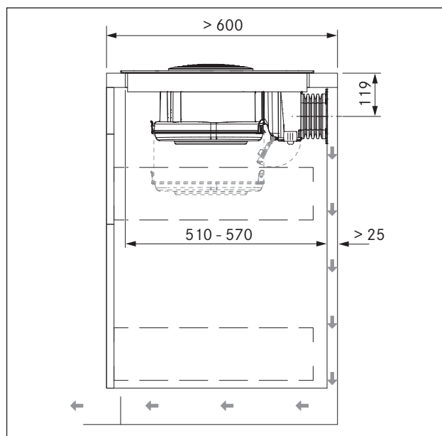
Fig. 6.10 Medidas de montagem com sistema de circulação de ar, profundidade da bancada 600 mm
