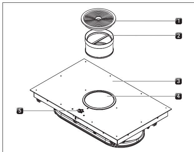
Fig. 5.1 Placa de cozinhar
