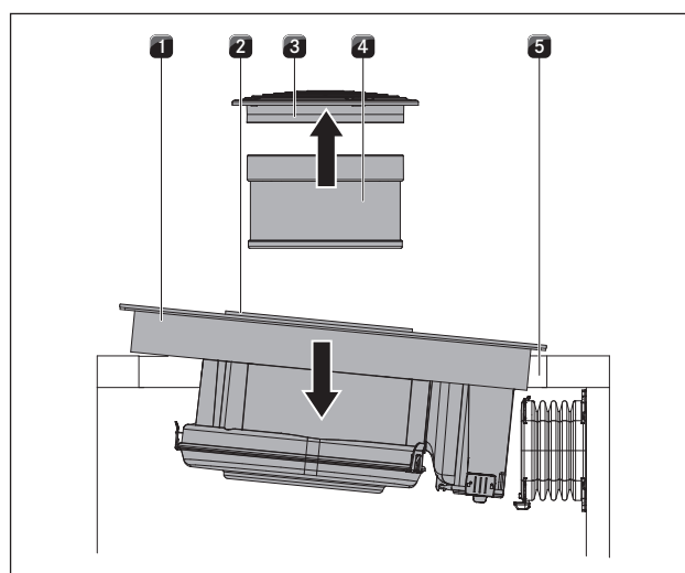
Fig. 6.13 Colocar a placa de cozinhar inclinada
