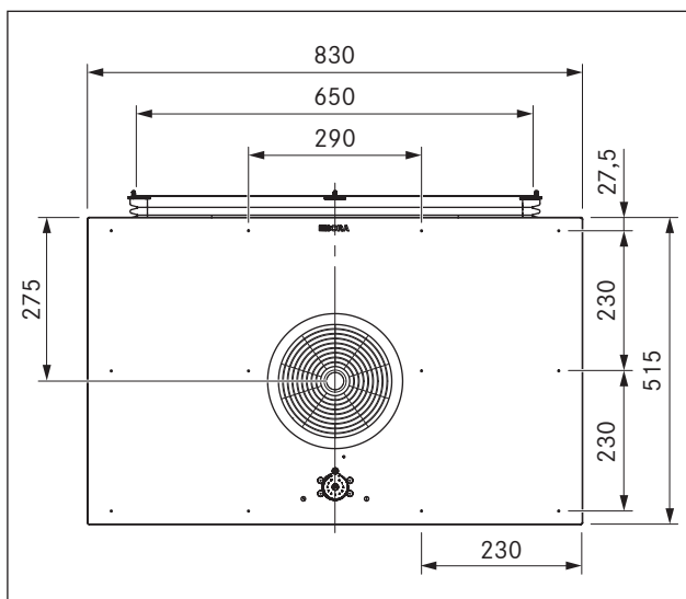
Fig. 3.5 BFIU dimensões do aparelho vista de cima
