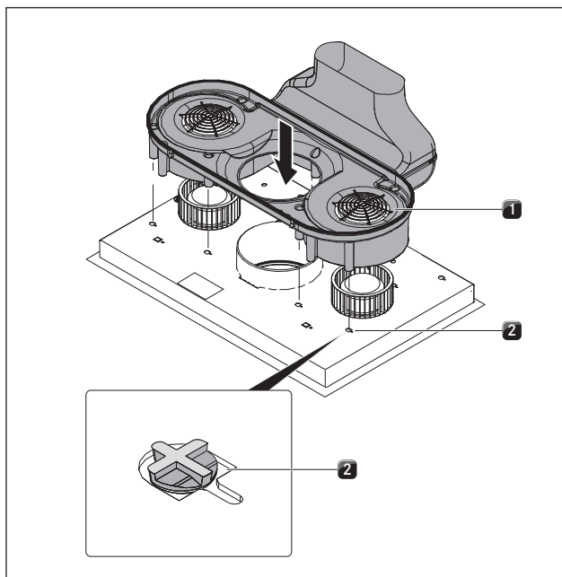
Fig. 6.30 Colocar o módulo de condução de ar na base da placa de cozinhar
