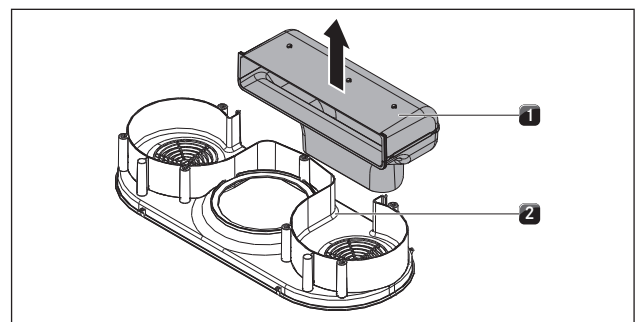
Fig. 6.28 Remover o cotovelo de extração de ar
