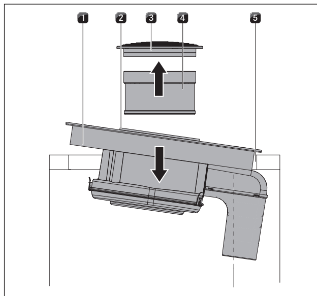
Fig. 6.33 Colocar a placa de cozinhar
