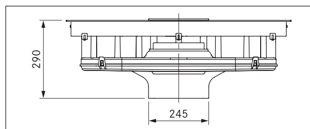
Fig. 3.2 BFIA dimensões do aparelho vista frontal
