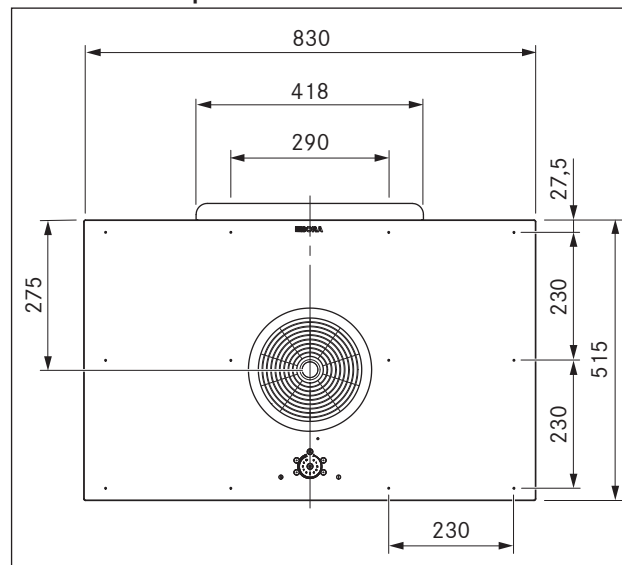
Fig. 3.1 BFIA dimensões do aparelho vista de cima
