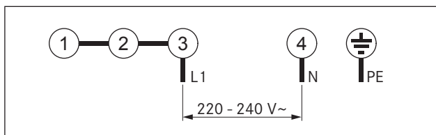
Fig. 6.38 Esquema de ligações ligação monofásica
