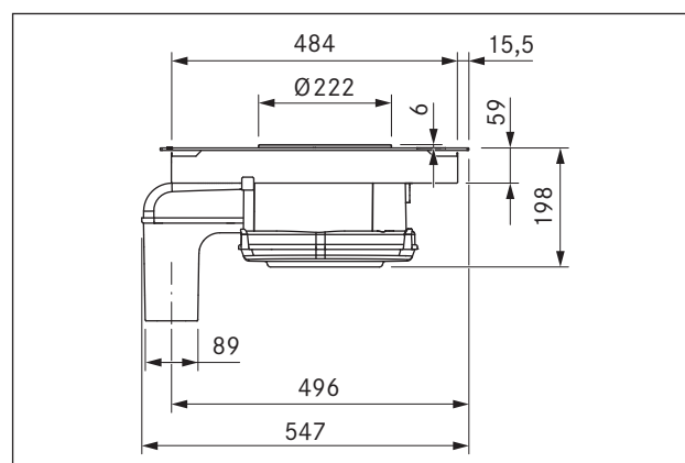
Fig. 3.3 BFIA dimensões do aparelho vista lateral
