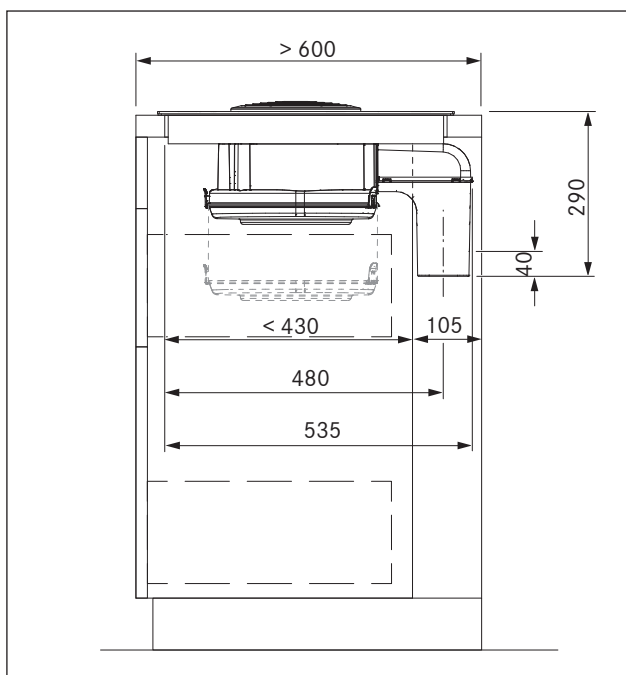
Fig. 6.22 Medidas de montagem com extração de ar, profundidade da bancada 600 mm
