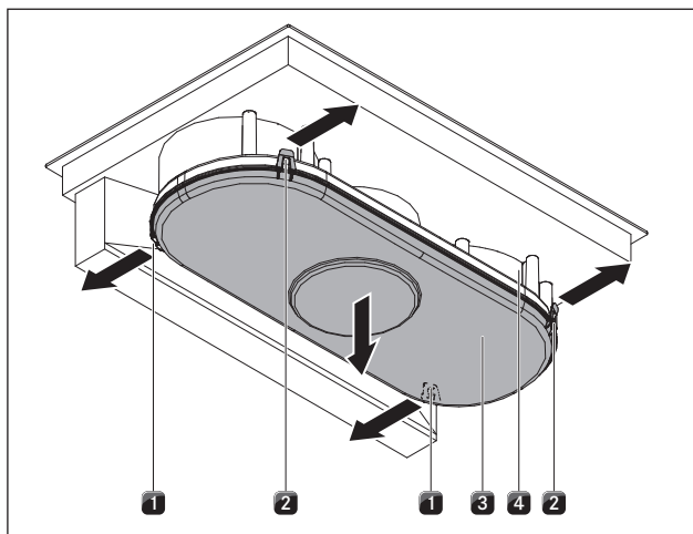
Fig. 8.3 Abrir a carcaça de condução do ar
