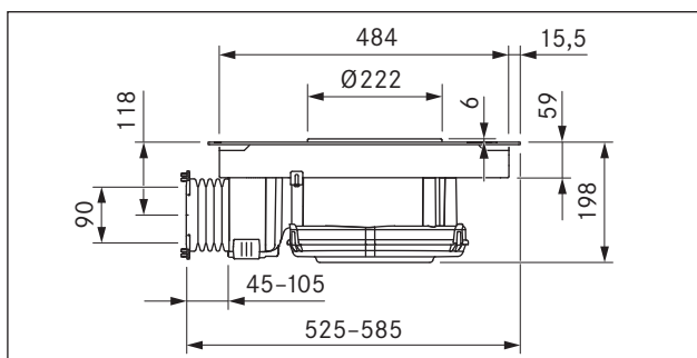
Fig. 3.7 BFIU dimensões do aparelho vista lateral
