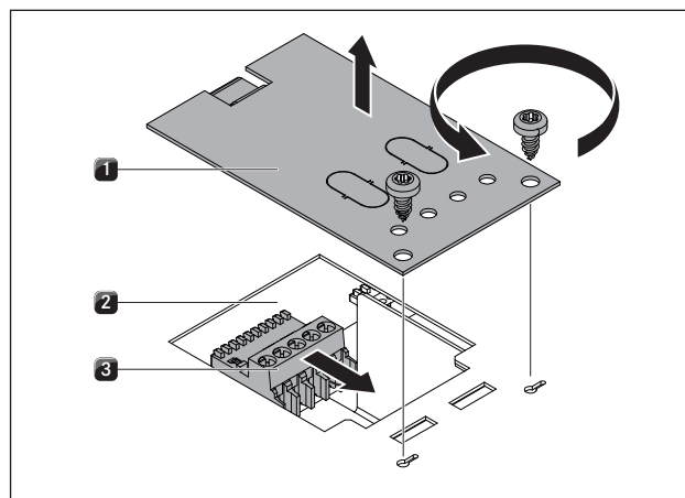
Fig. 6.41 Abrir a tampa e remover a ficha de contactos
