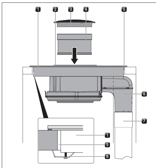
Fig. 6.35 Ligar a conduta de extração de ar + fixação
