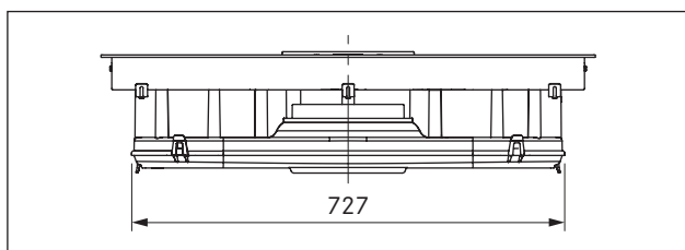
Fig. 3.6 BFIU dimensões do aparelho vista frontal
