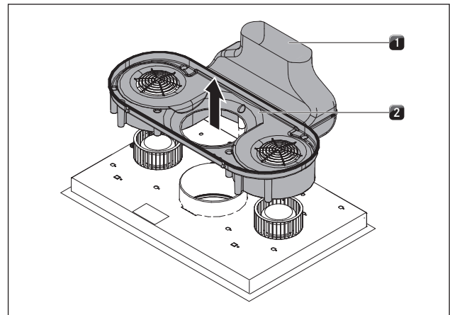
Fig. 6.27 Remover a carcaça de condução do ar
