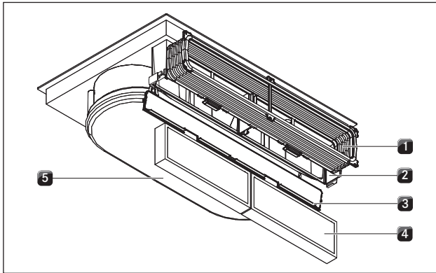
Fig. 5.2 Extrator de superfície com circulação de ar (BFIU)
