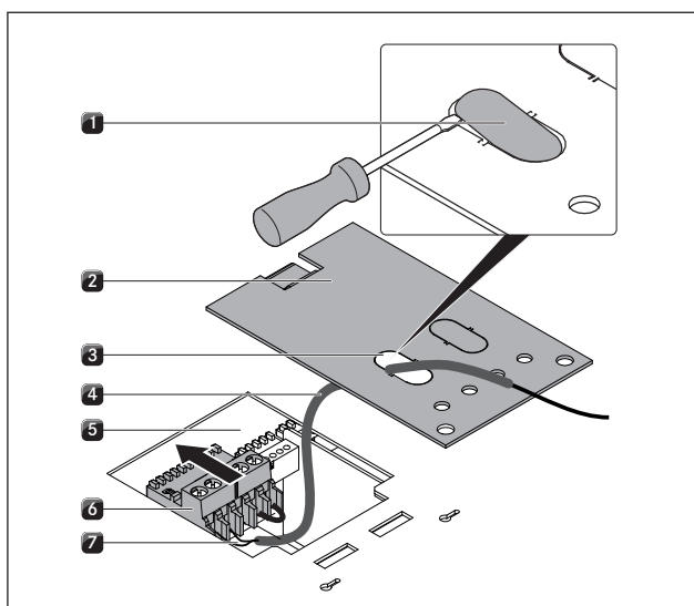
Fig. 6.43 Ligar o cabo
