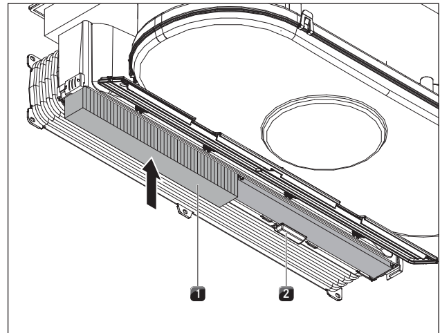
Fig. 8.9 Sette inn det aktive kullfilteret
