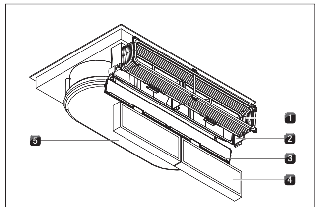
Fig. 5.2 Avtrekk resirkulering (BFU)
