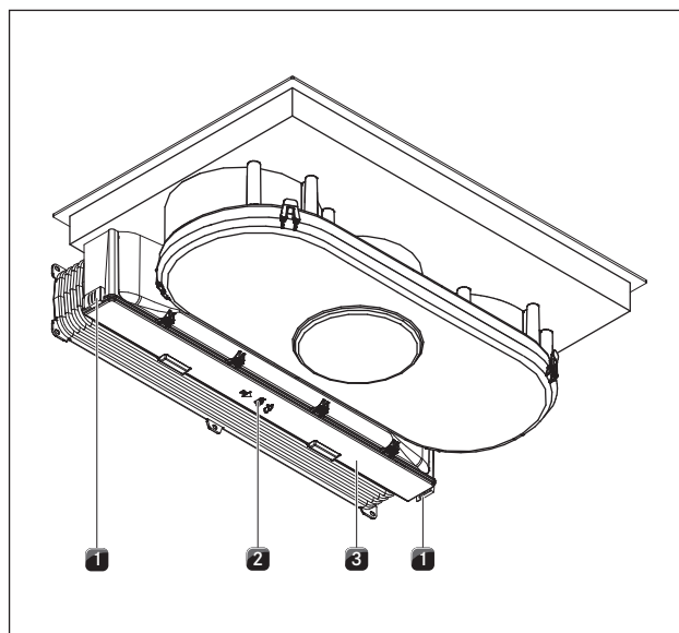
Fig. 8.5 Låse opp dekkelet aktivt kullfilterhus
