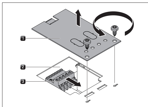
Fig. 6.41 Åpne dekelet og trekk ut kontaktstøpselet
