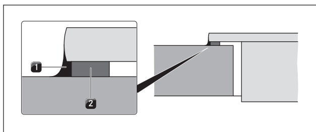
Fig. 6.7 Tettingsbånd ved overflatemontering
