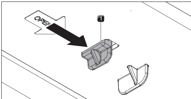
Fig. 8.7 Åpne den midtre låsen
