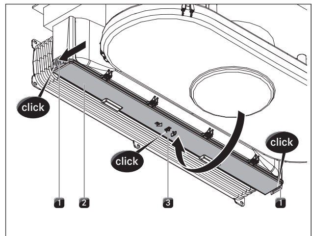
Fig. 8.10 Lukk apparatdekslet til det aktive kullfilteret
