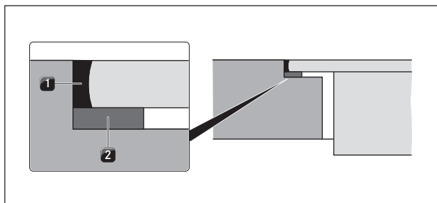
Fig. 6.8 Tettingsbånd ved planlimt montering
