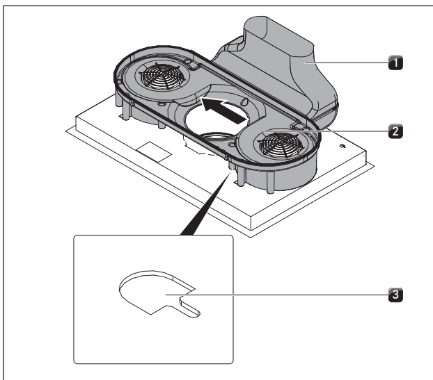
Fig. 6.26 Forskyve luftføringshuset
