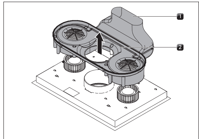
Fig. 6.27 Ta av luftføringshuset
