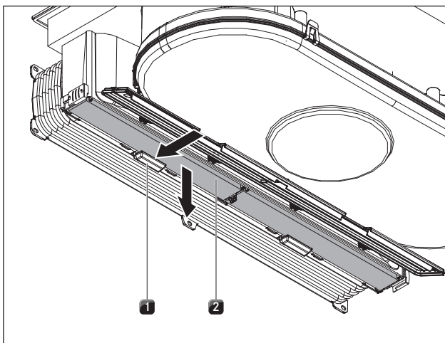
Fig. 8.8 Ta ut det aktive kullfilteret
