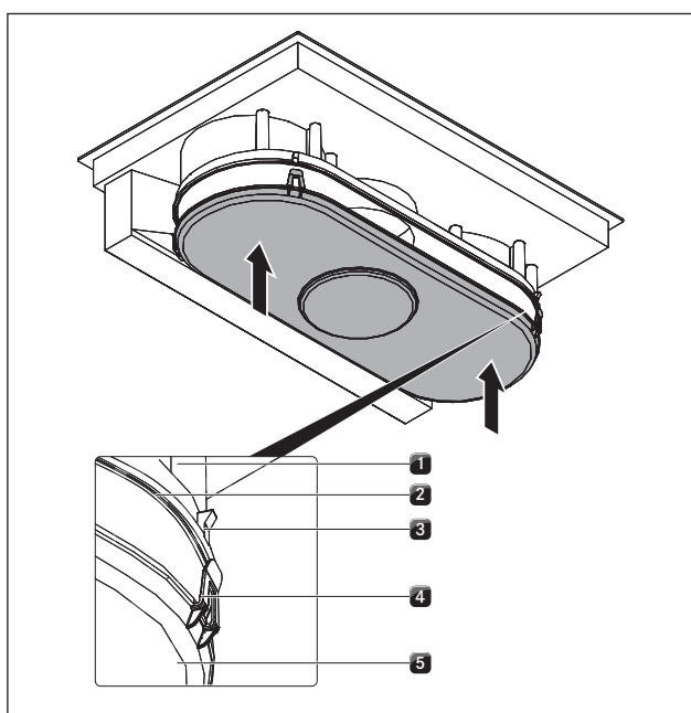
Fig. 8.4 Lukke luftføringshuset
