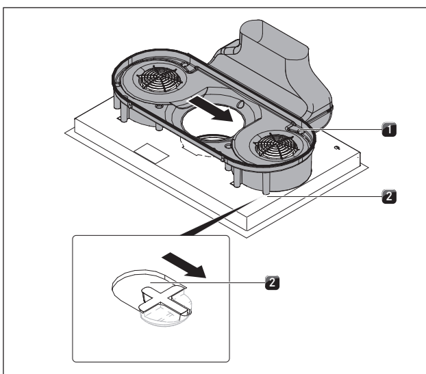
Afb. 6.31 Luchtgeleidingsmodule vastklikken
