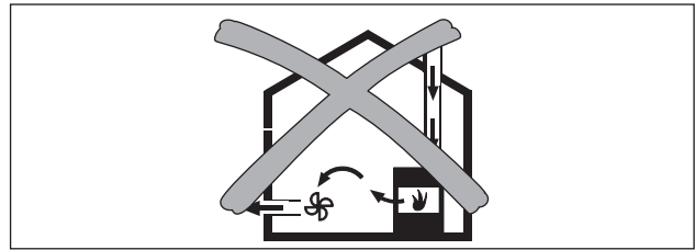
Afb. 6.19 Montage met luchtafvoer - niet toegestaan
