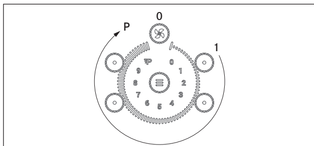
Afb. 7.2 Pauzefunctie inschakelen
