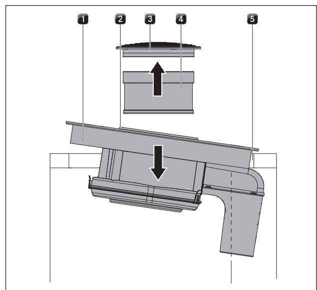
Afb. 6.33 Plaats het kookveld
