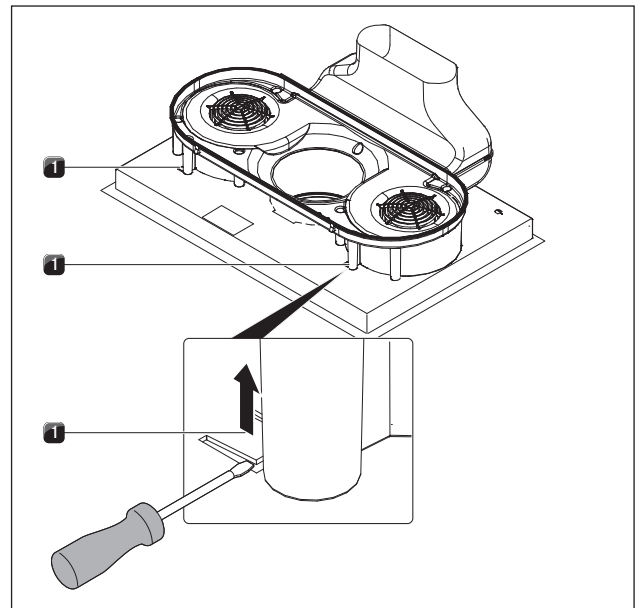
Afb. 6.32 Positiebeveiliging
