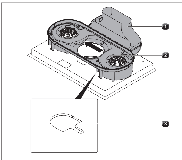
Afb. 6.26 Luchtgeleidingsbehuizing verschuiven
