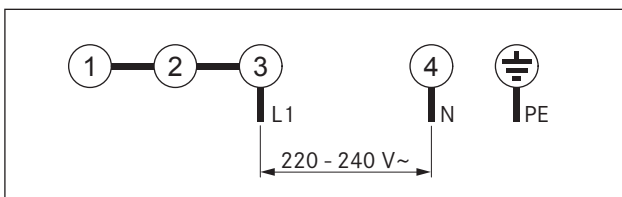
Afb. 6.38 Aansluitschema 1-fasen-aansluiting
