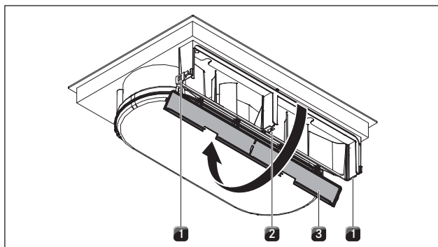
Afb. 6.14 Behuizingsdeksel openen
