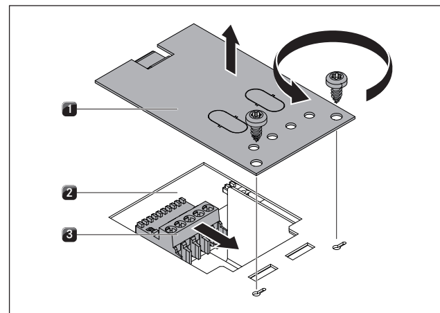
Afb. 6.41 Deksel openen en de contactstekker eruit halen
