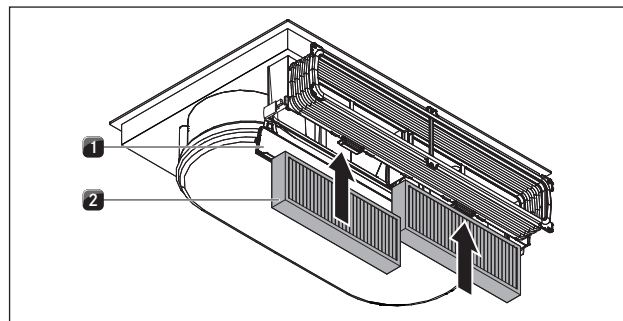
Afb. 6.16 Actieve-koolfilter plaatsen
