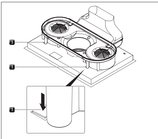
Afb. 6.25 Positiebeveiliging ontgrendelen
