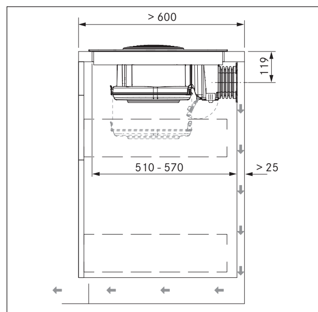
Afb. 6.10 Inbouwmaten bij recirculatie, werkbladhoogte 600 mm
