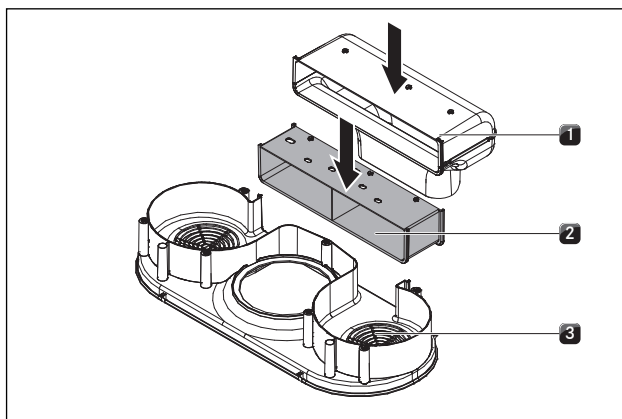
Afb. 6.29 Luchtafvoerkanaalverlenging plaatsen
