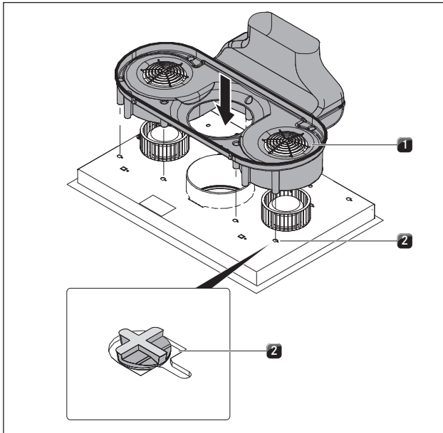
Afb. 6.30 Luchtgeleidingsmodule op de kookveldbodem monteren
