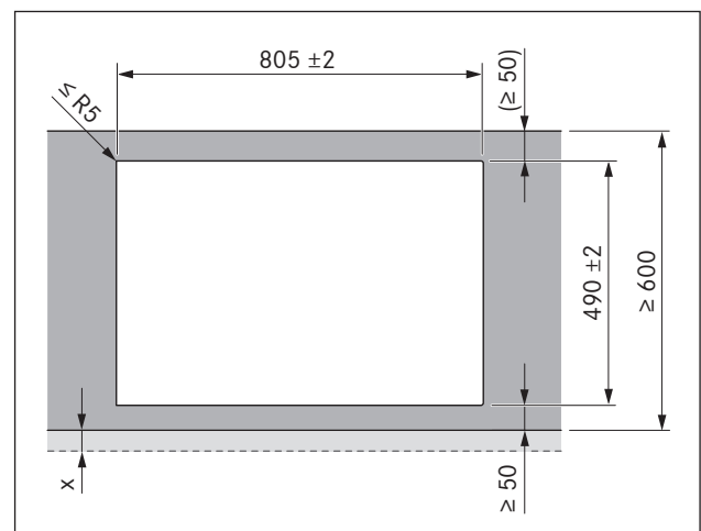
Afb. 6.5 De maten van de uitsparingen voor opbouwmontage
