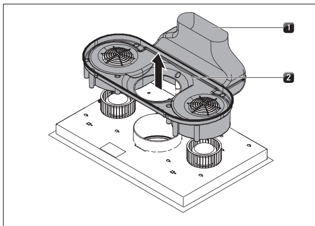
Afb. 6.27 Luchtgeleidingsbehuizing verwijderen
