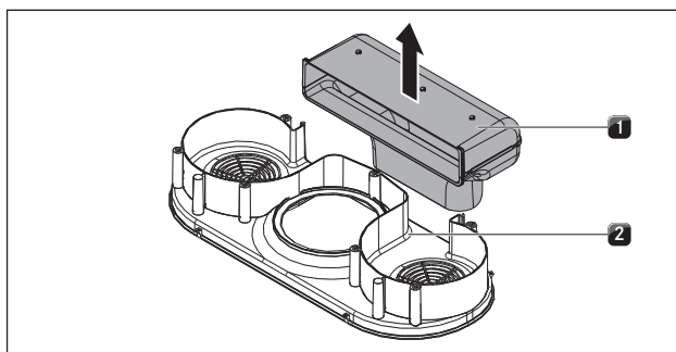
Afb. 6.28 Luchtafvoerboog verwijderen
