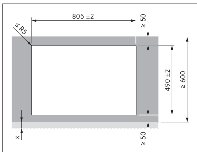
Fig. 6.5 Dimensioni intaglio per montaggio in battuta
