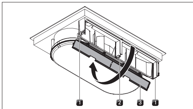
Fig. 6.14 Aprire il coperchio dell'alloggiamento
