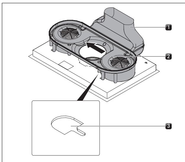
Fig. 6.26 Spostare l'alloggiamento della conduttura dell'aria
