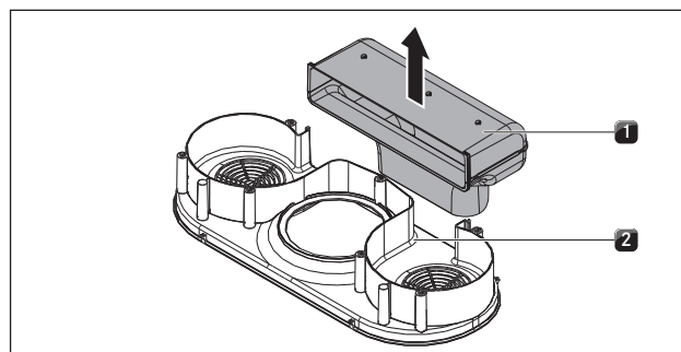
Fig. 6.28 Togliere la curva di scarico aria
