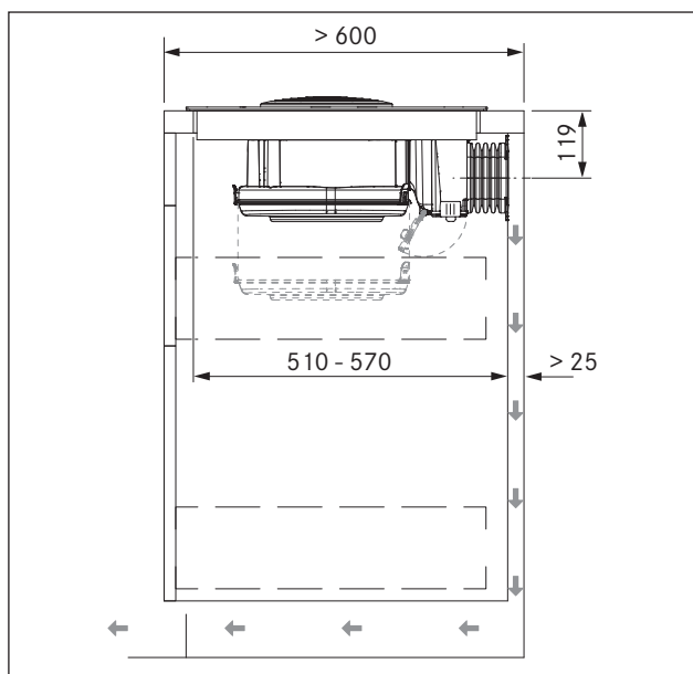
Fig. 6.10 Dimensioni di montaggio con sistema filtrante, profondità piano di lavoro 600 mm
