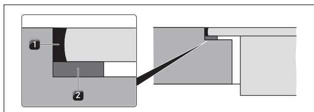
Fig. 6.8 Nastro a tenuta per montaggio a filo
