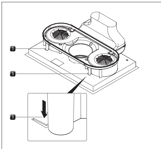
Fig. 6.25 Sbloccare la protezione di posizionamento
