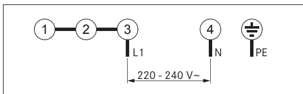
Kuva 6.38 Liitäntäkaavio - 1-vaiheiliitäntä
