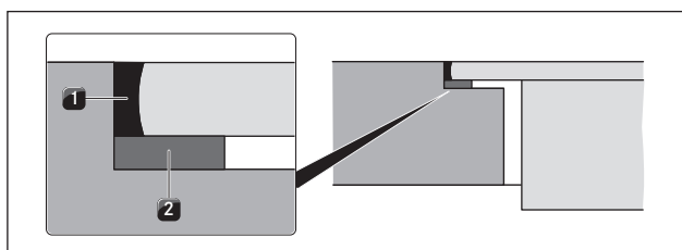
Kuva 6.8 Tiivistenauha uppoasennuksessa
