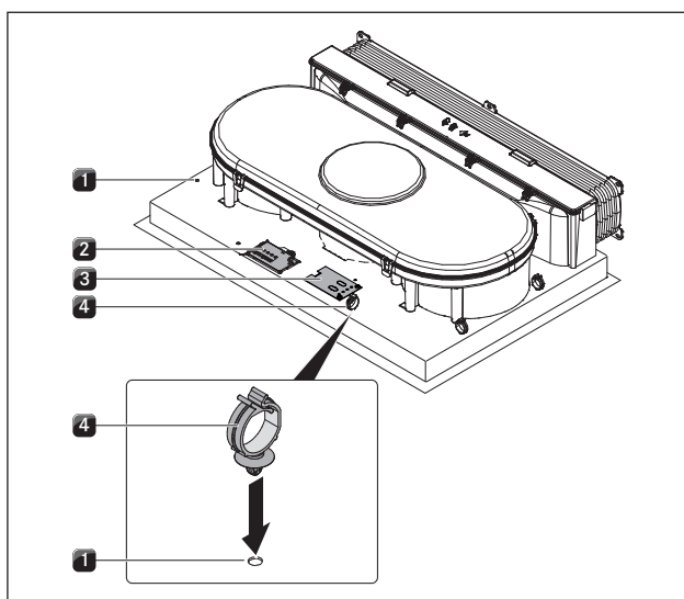
Kuva 6.39 Keittotason sähköliitännät
