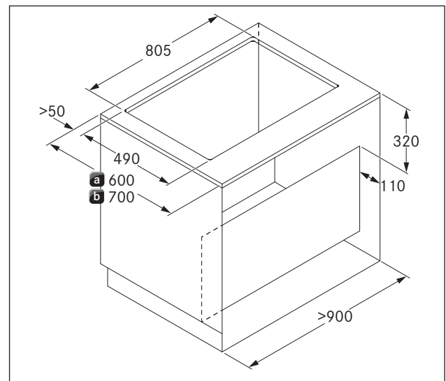
Kuva 6.21 Kalustemitat poistoilmakäytössä
