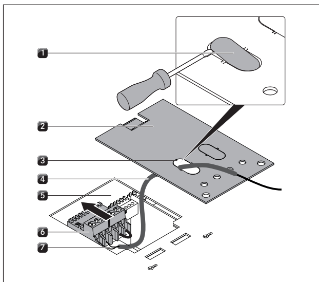
Kuva 6.43 Johdon liittäminen
