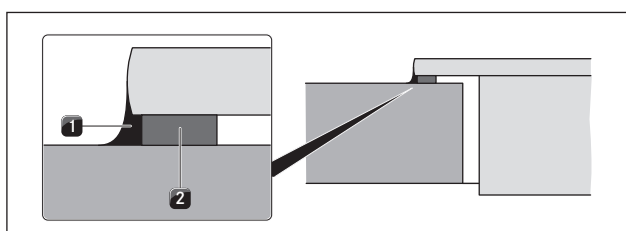
Kuva 6.7 Tiivistenauha pinta-asennuksessa
