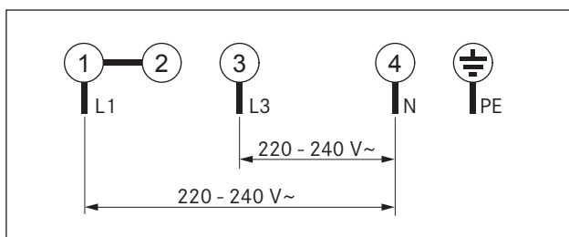
Kuva 6.37 Liitäntäkaavio - 2-vaiheiliitäntä
