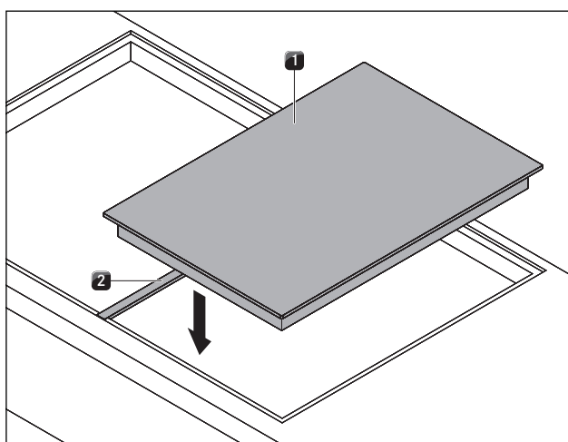
bild 5.14 Lägg i monteringskenan och spishällen
