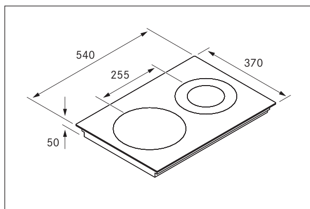
bild 3.1 Apparatsens mått
