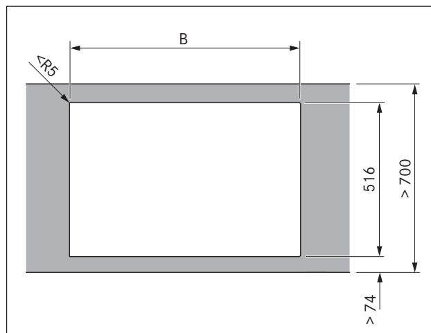
bild 5.5 Ytmontering
