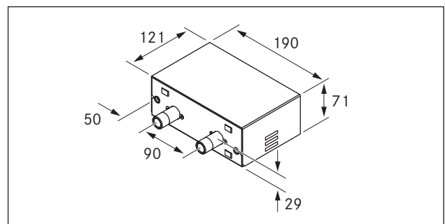
איור 3.2 מידות תיבת מתגים
