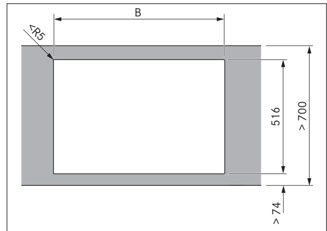
Fig. 5.5 Superposición
