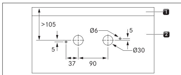
Fig. 5.10 Plantilla de perforación
