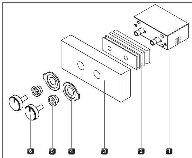
Fig. 5.9 Estructura de la caja de distribución
