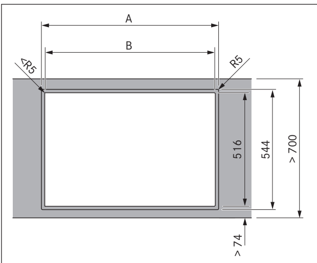
Fig. 5.3 Montaje enrasado
