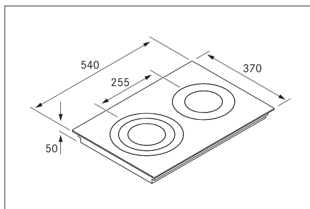
Fig. 3.1 Apparatmål PC32
