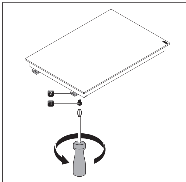
Fig. 5.16 Monteringsbøjler
