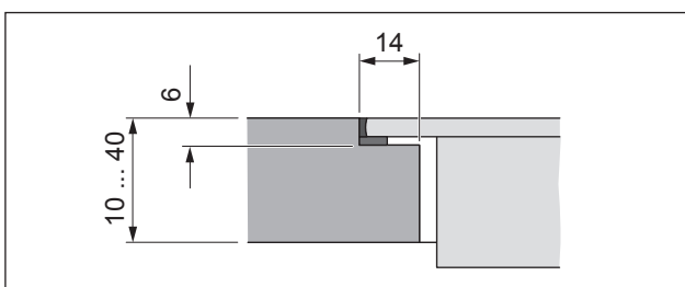
Fig. 5.4 Falsmålt til planlimet montering
