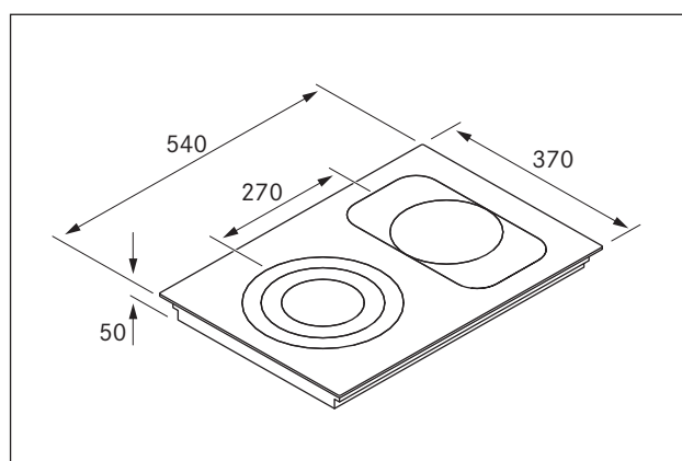
Fig. 3.2 Apparatmål PC3B
