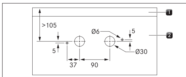
Fig. 5.10 Boreskabelon
