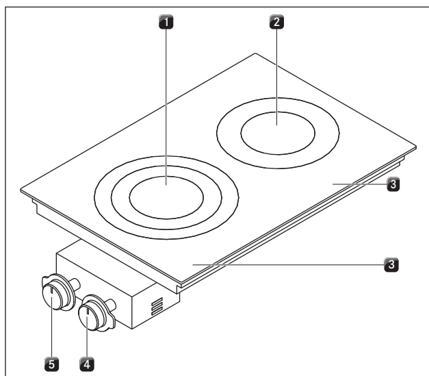
Fig. 4.1 Kogeplade PC32
