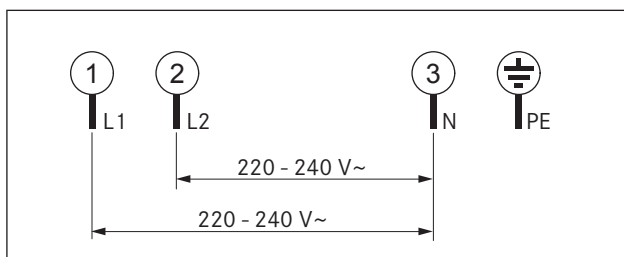
Fig. 5.17 Tilslutningsskema, 2-faset
