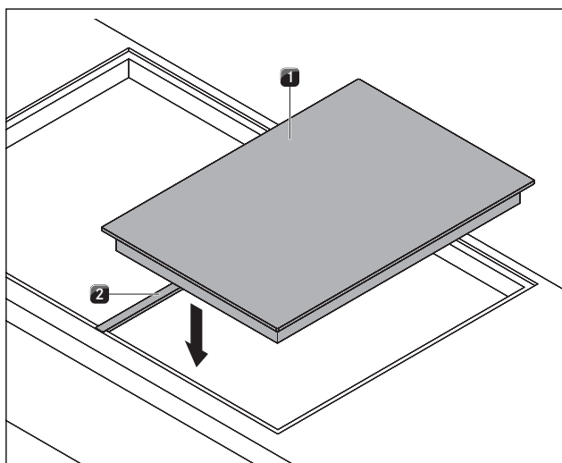
Fig. 5.14 Læg monteringskinnen og kogepladen ind
