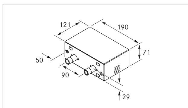
Fig. 3.3 Mål på styreboks PC32/PC3B
