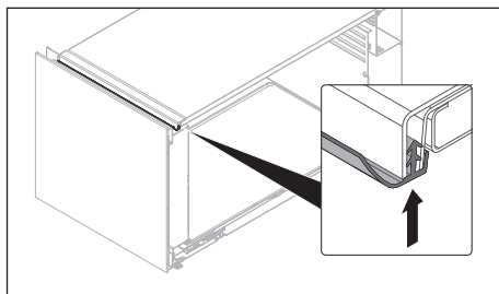
Fig. 9.18 Pose du joint profilé
