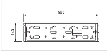
Fig. 3.8 Dimensions MS140 - Vue de devant
