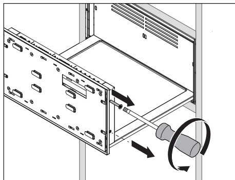
Fig. 9.16 Retrait du support de façade
