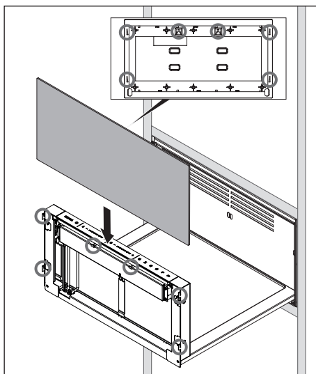
Fig. 9.13 Montage du support de façade
