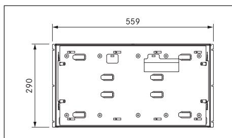
Fig. 3.2 Dimensions MS290 - Vue de devant
