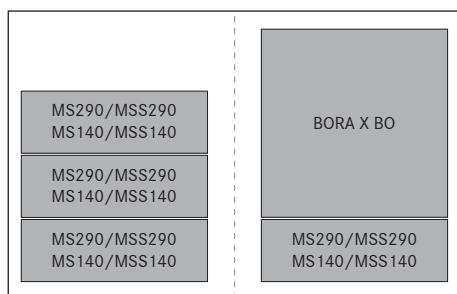
Fig. 9.1 Combinaisons d'appareils maximales
