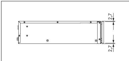
Fig. 3.9 Dimensions MS140 - Vue latérale
