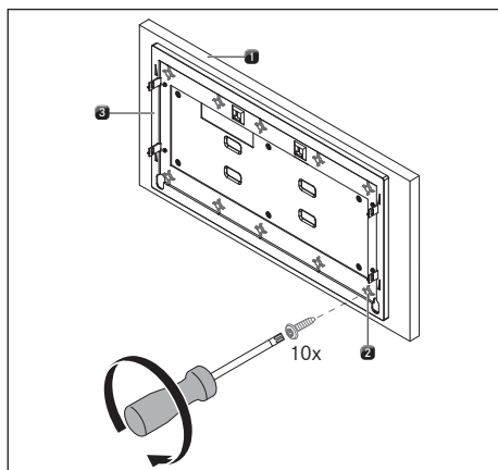
Fig. 9.12 Fixation de la façade de meuble
