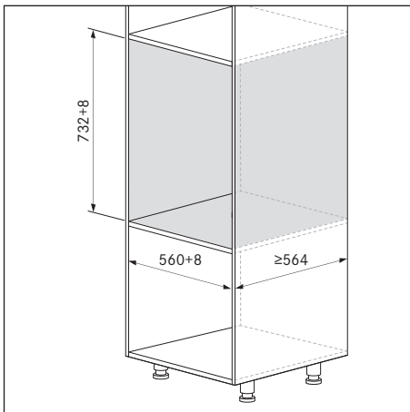
Fig. 9.5 Cotes de montage MS140/MSS140 + BORA X BO
