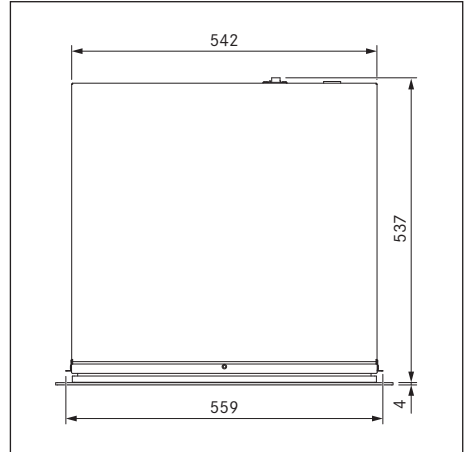
Fig. 3.10 Dimensions MSS140 - Vue de dessus
