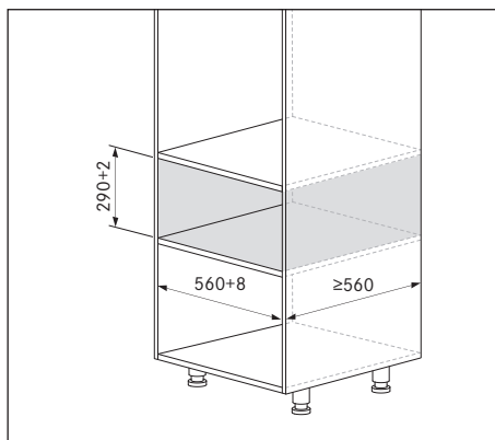
Fig. 9.2 Cotes de montage MS290/MSS290
