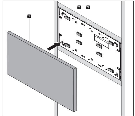
Fig. 9.10 Patins adhésifs sur le support de façade
