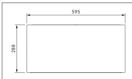
Fig. 3.5 Dimensions MSS290 - Vue de devant
