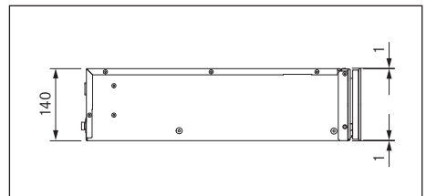
Fig. 3.12 Dimensions MSS140 - Vue latérale
