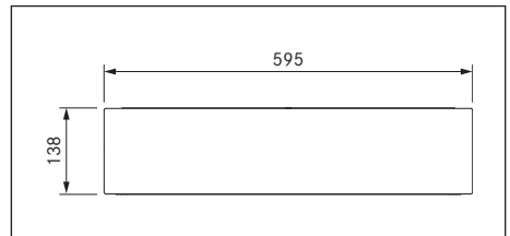
Fig. 3.11 Dimensions MSS140 - Vue de devant
