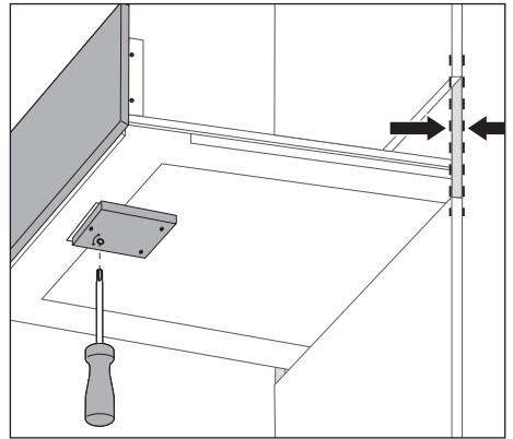
Fig. 9.15 Ajustement de la façade en profondeur
