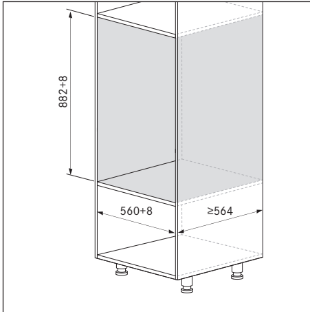
Fig. 9.4 Cotes de montage MS290/MSS290 + BORA X BO
