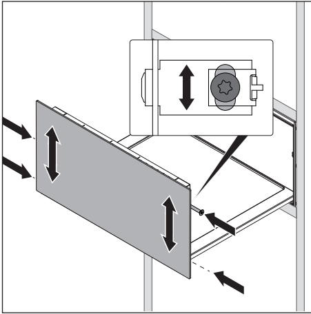
Fig. 9.14 Ajustement horizontal
