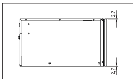
Fig. 3.3 Dimensions MS290 - Vue latérale
