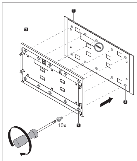
Fig. 9.17 Fixation de la façade en verre
