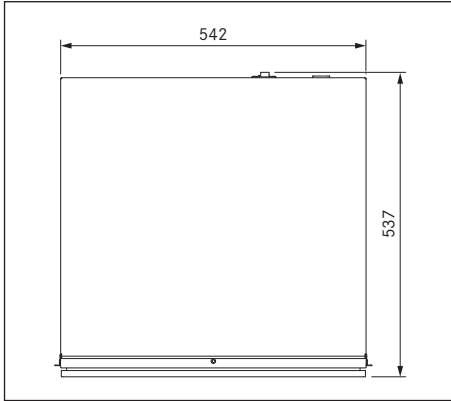
Fig. 3.7 Dimensions MS140 - Vue de dessus
