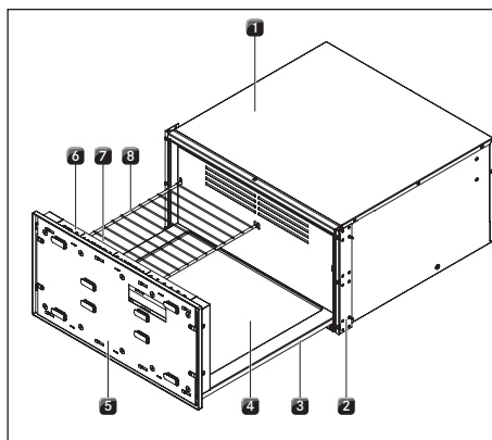
Fig. 4.1 Composition du tiroir multifonction
