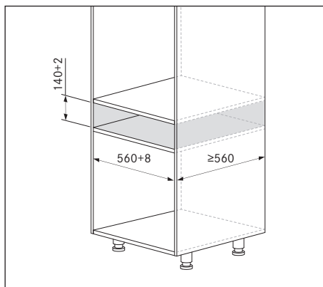
Fig. 9.3 Cotes de montage MS140/MSS140
