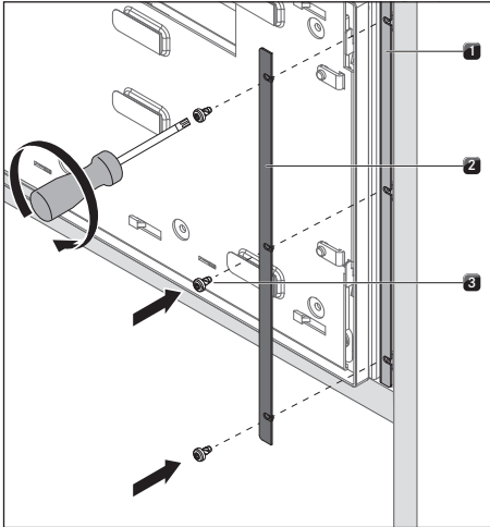
Fig. 9.9 Fixer l'appareil
