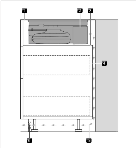
Fig. 9.21 Variante di montaggio con piano intermedio
