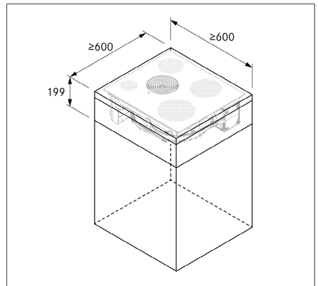
Fig. 9.4 Dimensioni minime mobili S Pure
