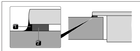
Fig. 9.12 Nastro a tenuta per montaggio in battuta
