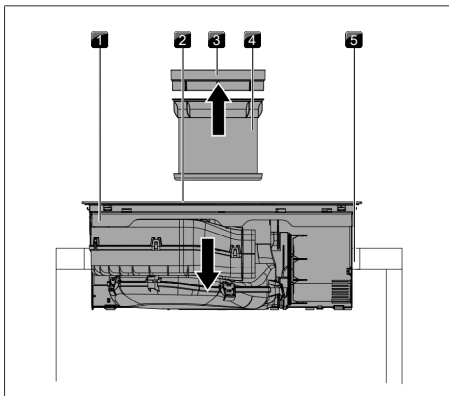
Fig. 9.14 Inserire il piano cottura
