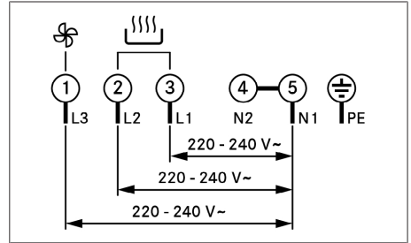
Fig. 9.35 Schema di collegamento connessione a trifase
