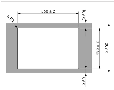
Fig. 9.7 Dimensioni intaglio per montaggio in battuta
