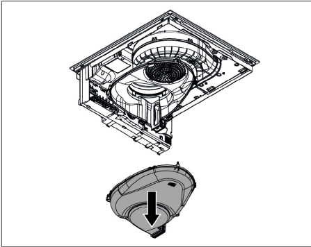
Fig. 9.34 Smontare la parte inferiore del sistema di aspirazione
