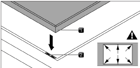
Fig. 9.16 Posizionamento dei pannelli di compensazione altezza
