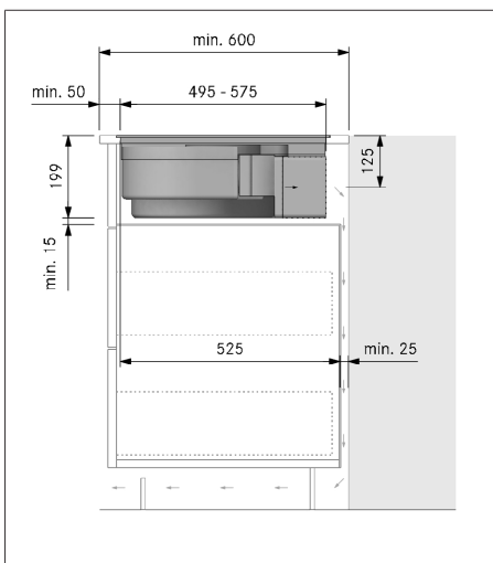
Fig. 9.25 Dimensioni di montaggio con sistema filtrante variante di montaggio B, profondità piano di lavoro 600 mm
