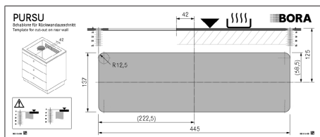
Fig. 9.24 Maschera per intaglio parete posteriore
