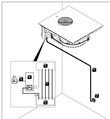
Fig. 9.39 Schema di collegamento con contatti di commutazione esterni
