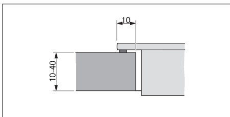
Fig. 9.8 Misura d'appoggio per montaggio in battuta
