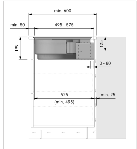
Fig. 9.22 Dimensioni di montaggio con sistema filtrante, variante di montaggio A
