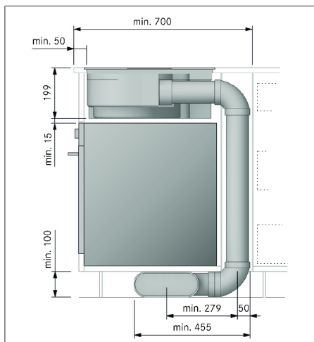
Fig. 9.6 PURSA sopra il forno con la canalina nell'area di base
