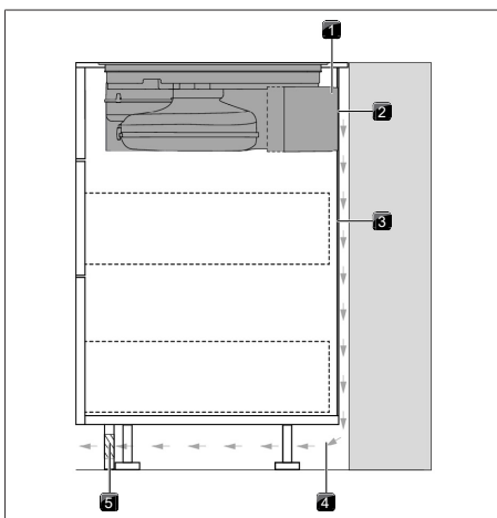
Fig. 9.20 Variante di montaggio con parete posteriore passante
