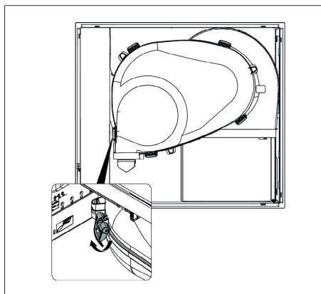
Fig. 9.33 Chiusure del sistema di aspirazione
