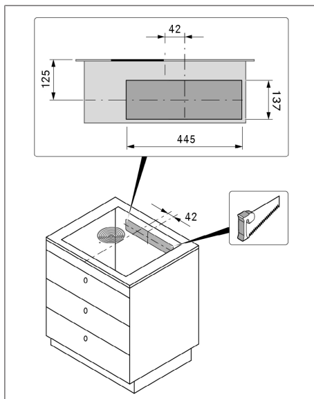
Fig. 9.23 Sezione parete posteriore
