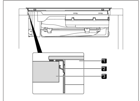
Fig. 9.29 Fissare il piano cottura
