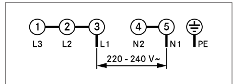
Fig. 9.37 Schema di collegamento connessione monofase
