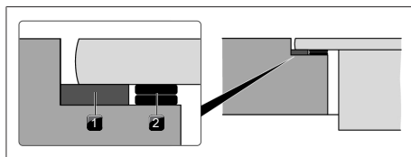
Fig. 9.31 Pannelli di compensazione altezza
