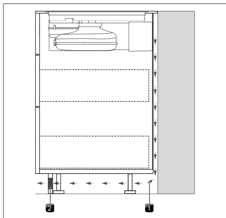
Fig. 9.19 Apertura di sfogo nell'area dello zoccolo
