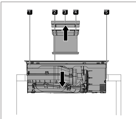
Fig. 9.28 Inserire il piano cottura
