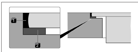
Fig. 9.13 Nastro a tenuta per montaggio a filo piano
