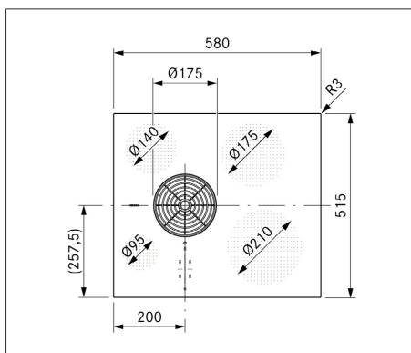
Fig. 3.1 Vista dall'alto PURSA
