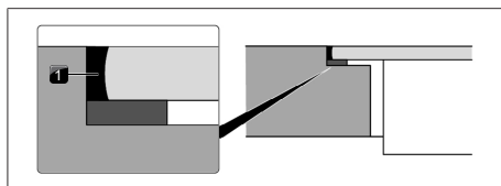
Fig. 9.45 Pasta sigillante al silicone per montaggio a filo piano
