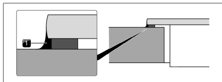
Fig. 9.44 Pasta sigillante al silicone per montaggio in battuta
