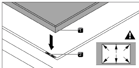
Fig. 9.30 Applicare i pannelli di compensazione altezza
