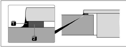
Fig. 9.26 Nastro a tenuta per montaggio in battuta
