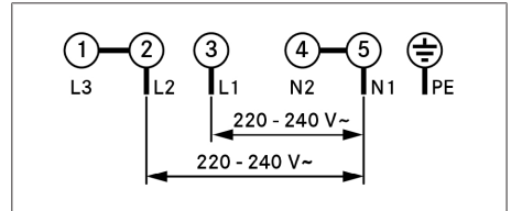
Fig. 9.36 Schema di collegamento connessione bifase
