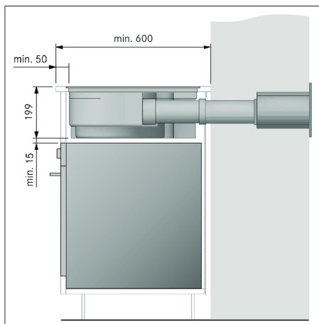
Fig. 9.5 PURSA sopra il forno con la guida dell'aria diretta verso la parte posteriore in una scatola a parete
