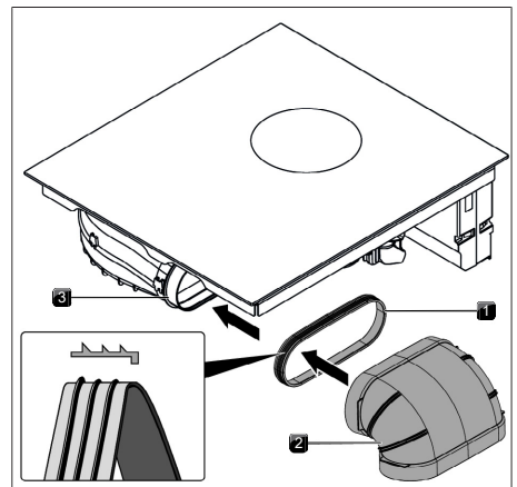
Fig. 9.18 Connessione al sistema di canali
