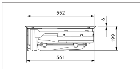
Fig. 3.2 Vista frontale PURSA
