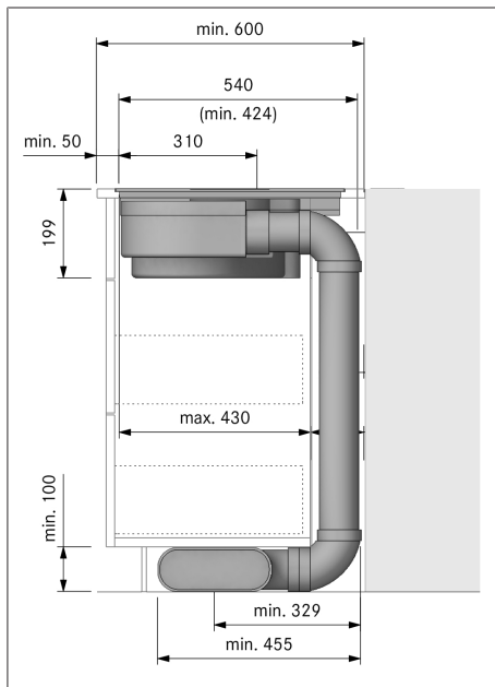
Fig. 9.11 Dimensioni di montaggio con sistema aspirante, profondità piano di lavoro 600 mm
