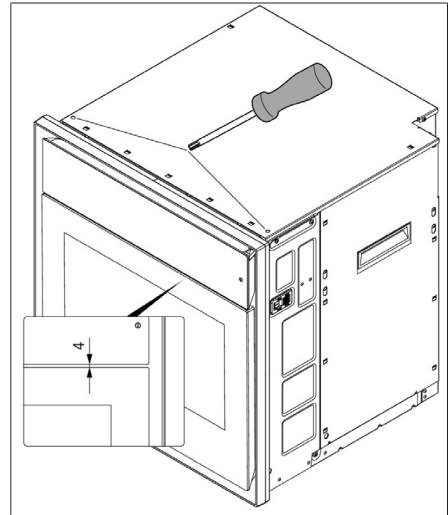
Fig. 8.14 Ajustar a distância entre a unidade de comando e a porta
