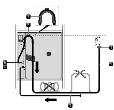
Fig. 8.12 Drenagem da água através do suporte da mangueira
