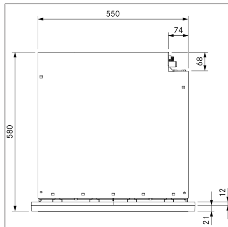
Fig. 3.2 Vista de cima do XBO
