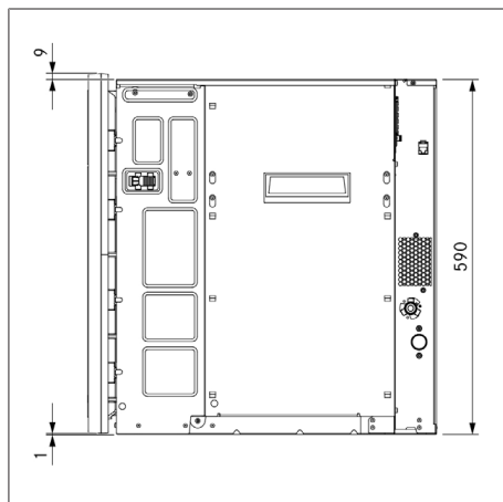
Fig. 3.3 Vista lateral do XBO
