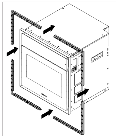
Fig. 8.6 Desmontar a estrutura de espaçamento
