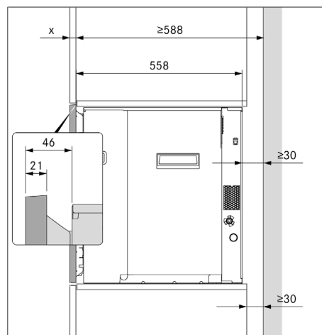
Fig. 8.3 Dimensões de instalação sem estrutura de espaçamento
