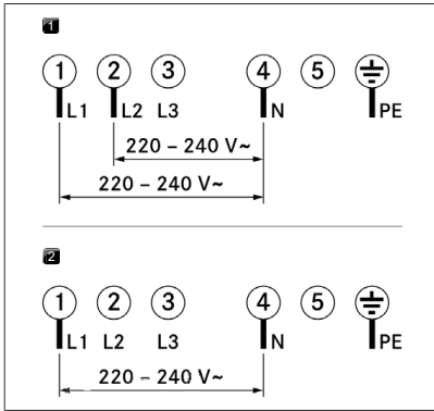
Fig. 8.13 Esquemas de ligação
