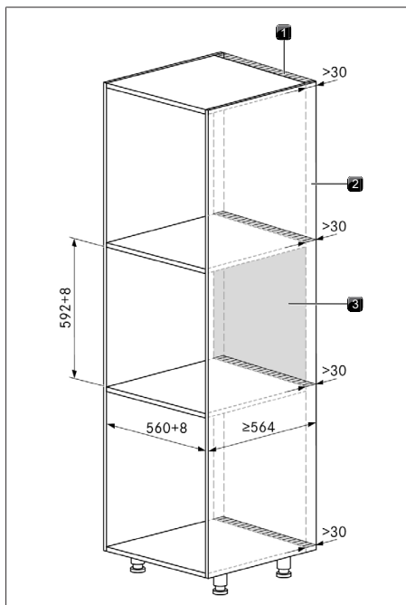
Fig. 8.1 Armário embutido
