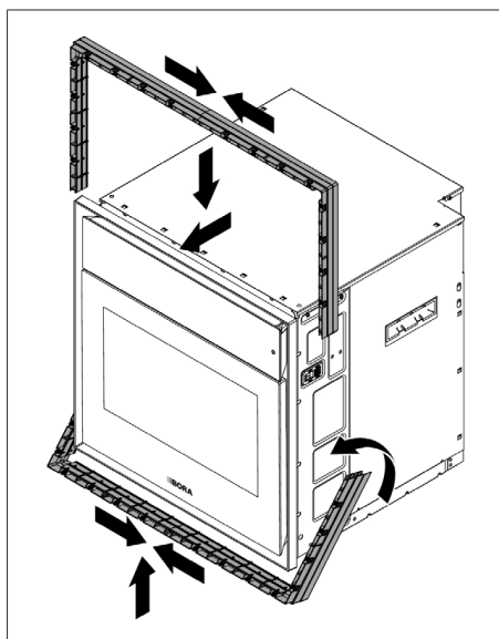
Fig. 8.8 Montagem de 2 estruturas de espaçamento
