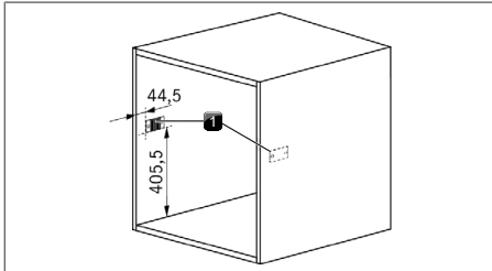
Fig. 8.9 Nicho embutido com placas de retenção do armário
