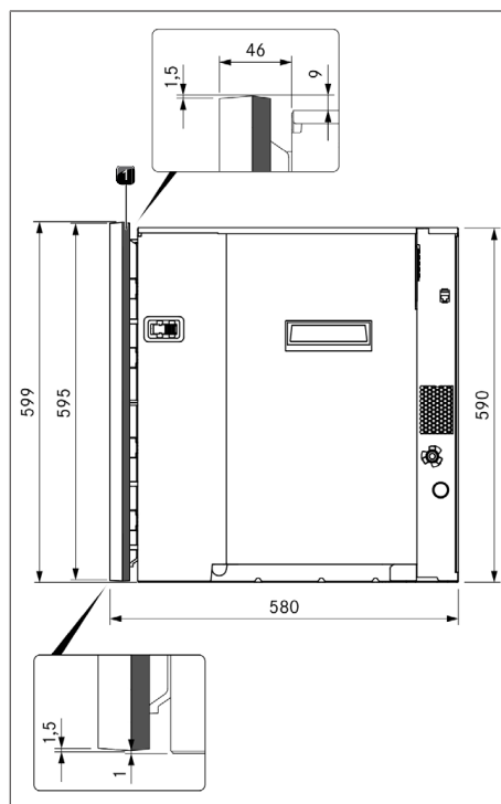
Fig. 8.2 Dimensões do aparelho
