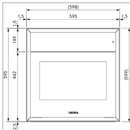
Fig. 3.1 Vista frontal do XBO
