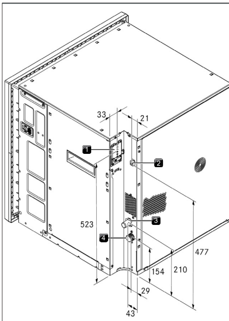
Fig. 8.10 Ligações do aparelho
