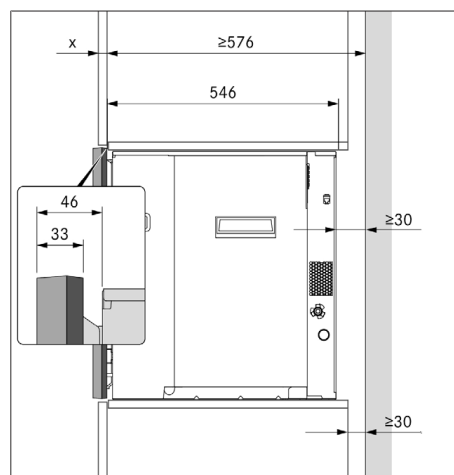
Fig. 8.4 Dimensões de instalação com 1 estrutura de espaçamento
