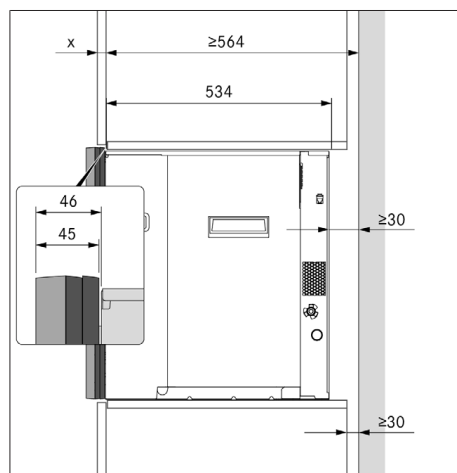
Fig. 8.5 Dimensões de instalação com 2 estruturas de espaçamento
