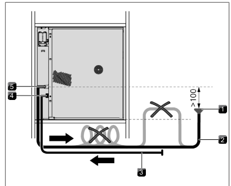
Fig. 8.11 Drenagem da água
