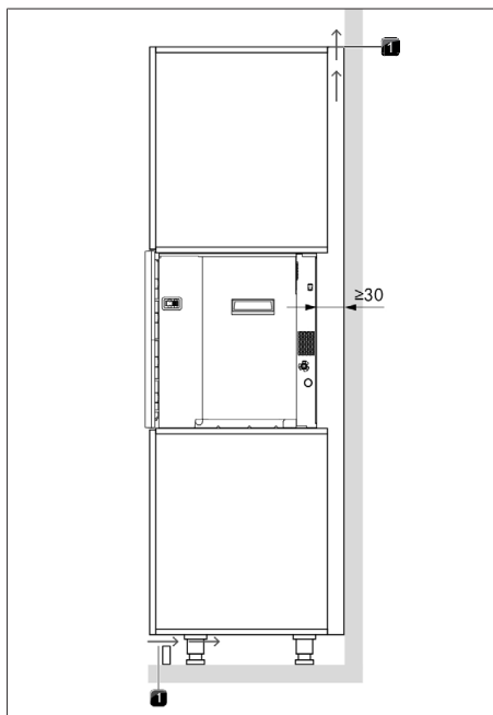
Fig. 8.16 Ventilação
