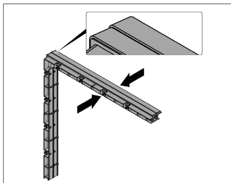
Fig. 8.7 2 elementos da estrutura de espaçamento
