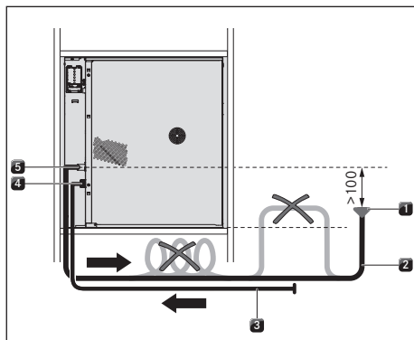
Fig. 9.11 Scarico dell'acqua
