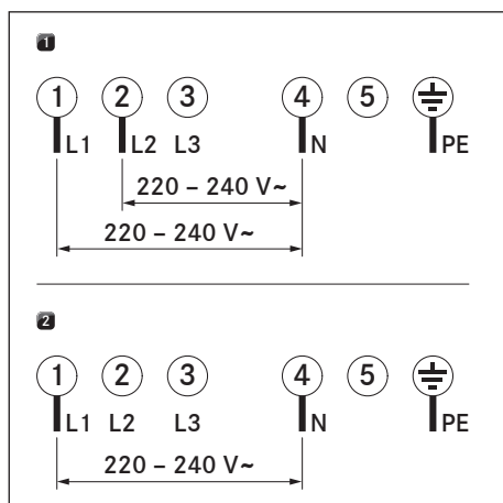
Fig. 9.13 Schéma de raccordement
