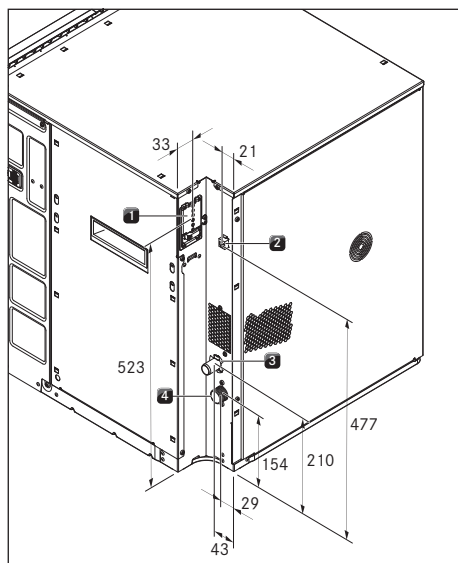
Fig. 9.10 Raccordement de l'appareil
