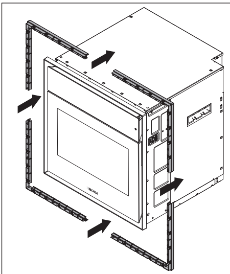
Fig. 9.6 Démontez le cadre d'écartement
