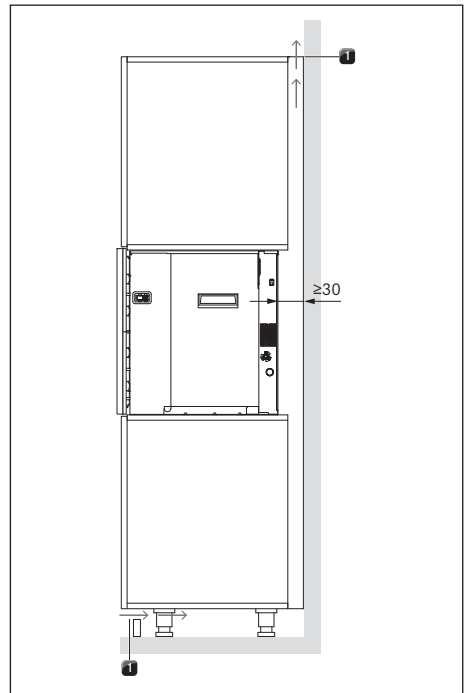
Fig. 9.16 Aération
