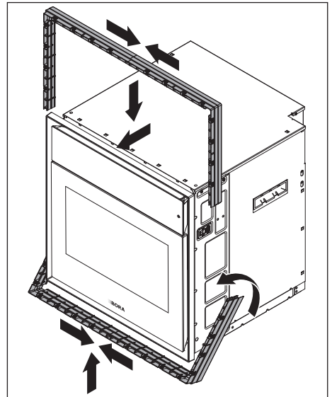
Fig. 9.8 Monter 2 cadres d'écartement
