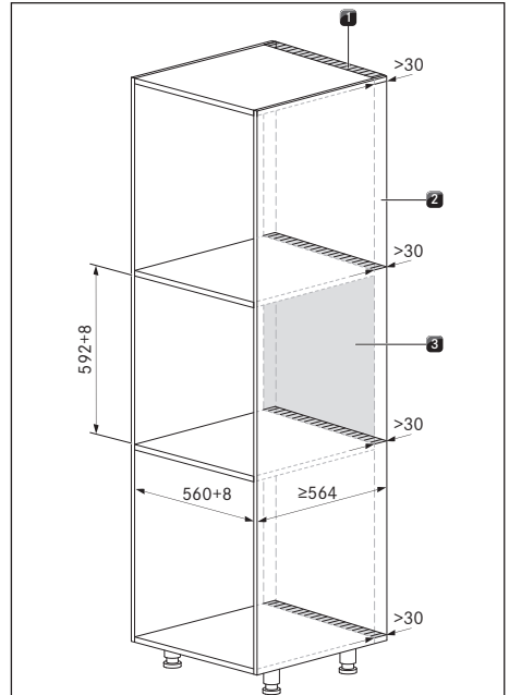
Fig. 9.1 Armoire d'encastrement
