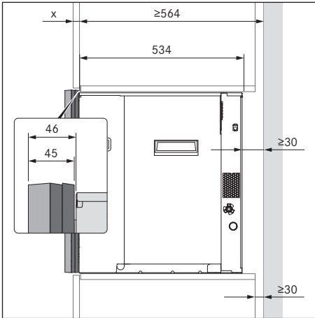
Fig. 9.5 Cotes de montage avec deux cadres d'écartement
