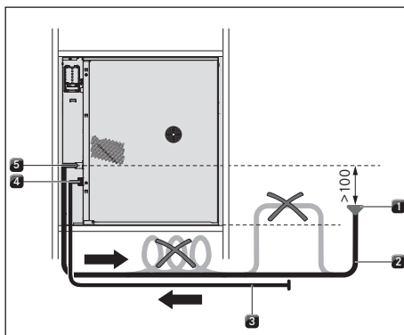
Fig. 9.11 Évacuation d'eau
