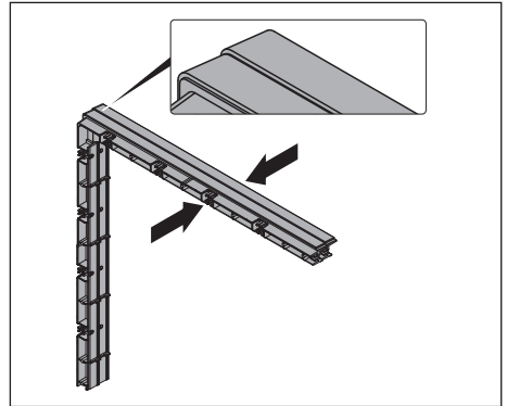
Fig. 9.7 Éléments de 2 cadres d'écartement
