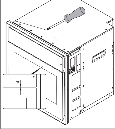
Kuva 9.14 Käyttöyksikön ja luukun välisen etäisyyden säätö
