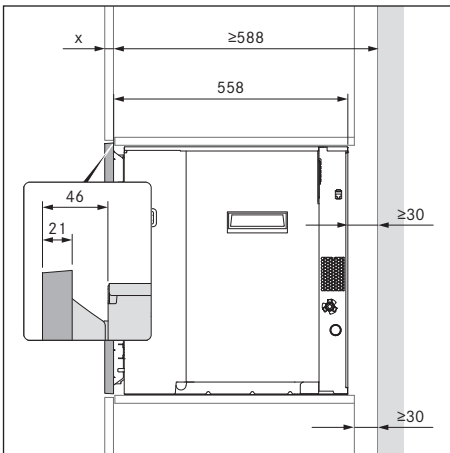
Kuva 9.3 Asennusmitat ilman kehysvälikettä
