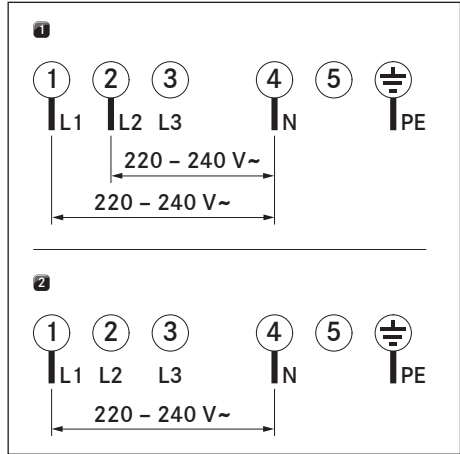
Kuva 9.13 Liitäntäkaaviot
