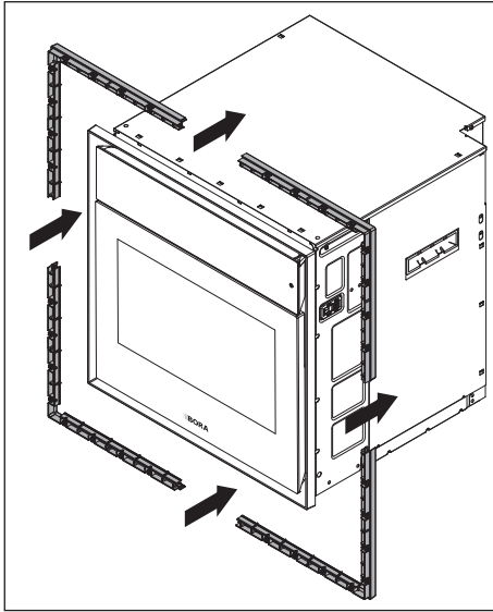
Kuva 9.6 Kehysvälikkeen irrottaminen
