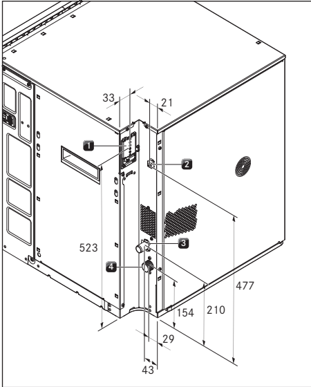
Kuva 9.10 Laitteen liitännät
