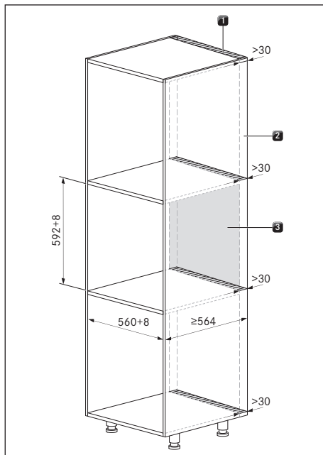
Kuva 9.1 Kalustekaappi
