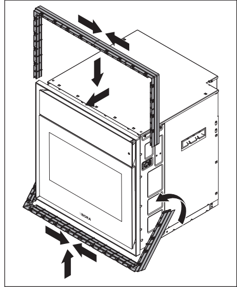
Kuva 9.8 2 kehysovien asennus
