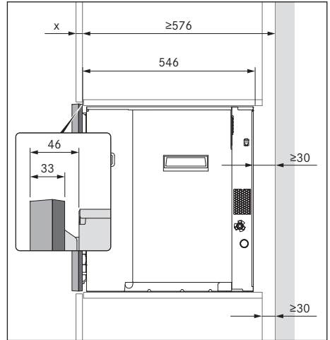
Kuva 9.4 Asennusmitat, 1 kehysvälike
