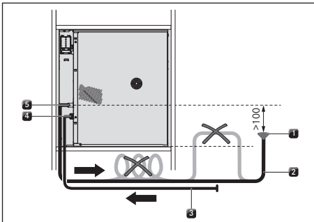
Kuva 9.11 Vedenpoisto
