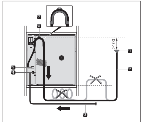
Kuva 9.12 Vedenpoisto kannakekaaren kautta
