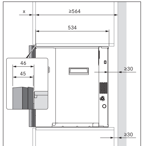
Kuva 9.5 Asennusmitat, 2 kehysvälikettä
