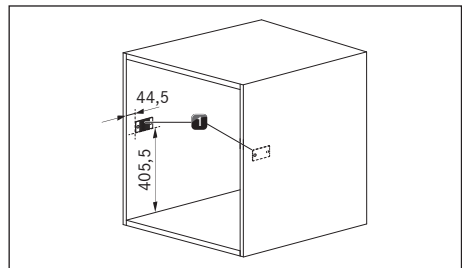
Kuva 9.9 Asennusaukko ja kalusteen kiinnityslevyt
