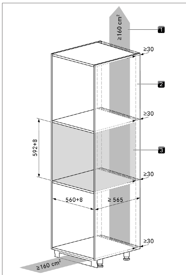
obr. 9.1 Vestavná skříňka
