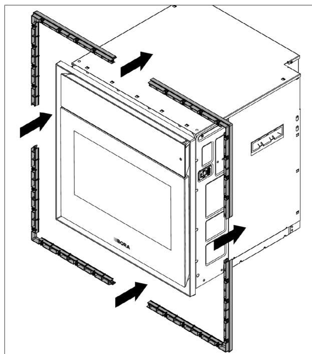
obr. 9.6 Demontáž distančního rámu
