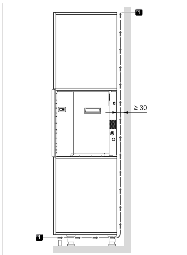
obr. 9.16 Větrání
