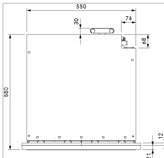
obr. 3.2 Pohled shora na spotřebič XBO
