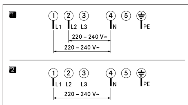
obr. 9.13 Schémata zapojení
