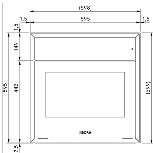
obr. 3.1 Pohled zepředu na spotřebič XBO
