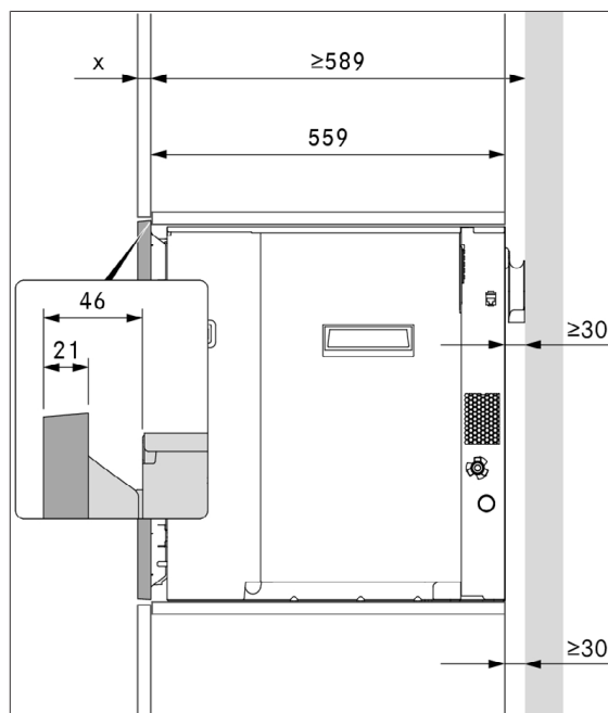
obr. 9.3 Montážní rozměry bez distančního rámu
