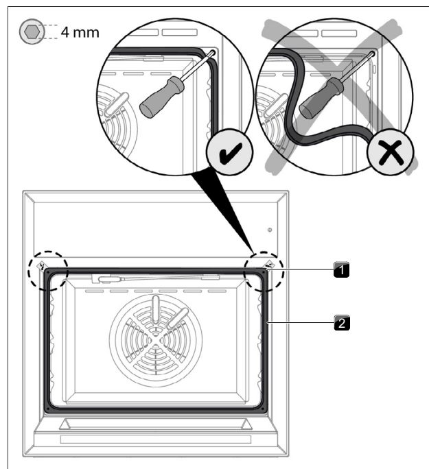
obr. 9.15 Připevnění spotřebiče
