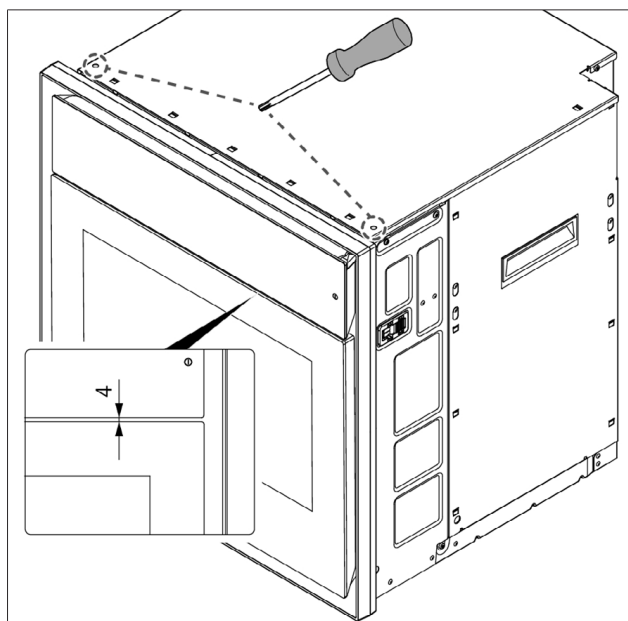
obr. 9.14 Nastavení vzdálenosti ovládací jednotky a dvířek
