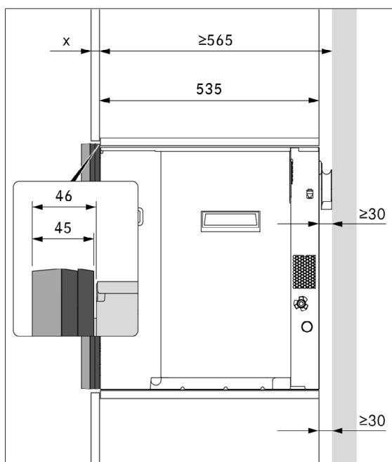
obr. 9.5 Montážní rozměry se 2 distančními rámy
