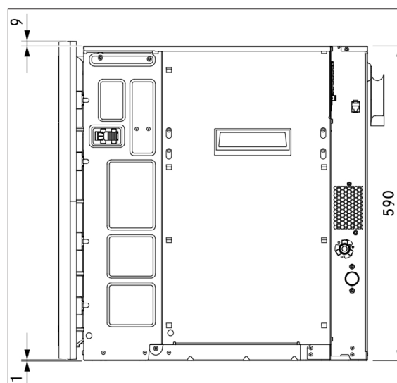
obr. 3.3 Pohled z boku na spotřebič XBO
