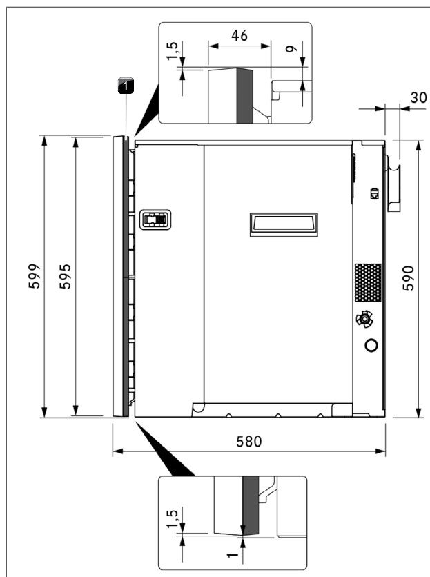
obr. 9.2 Rozměry
