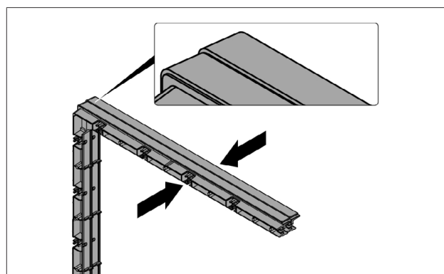
obr. 9.7 2 prvky distančního rámu
