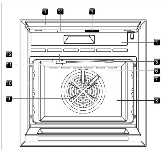
obr. 4.1 Uspořádání – část 1
