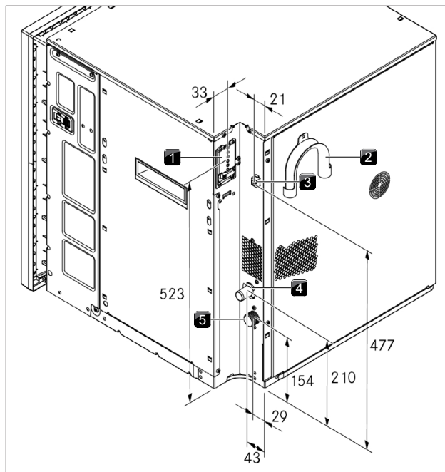
obr. 9.10 Připojky zařízení
