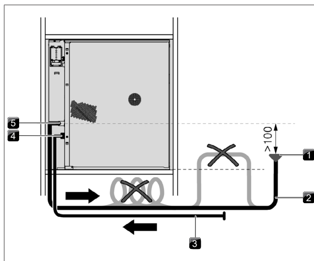
obr. 9.11 Odvod vody
