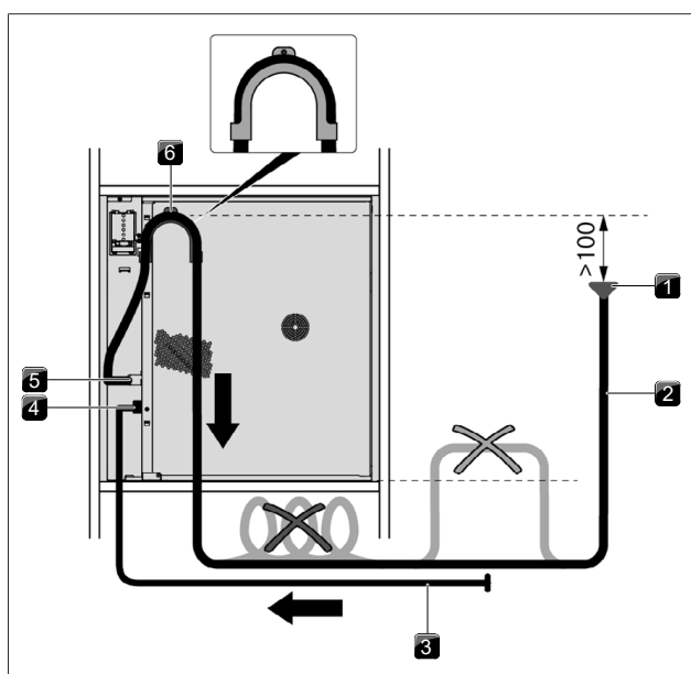
obr. 9.12 Odvod vody přes přídržné kolínko
