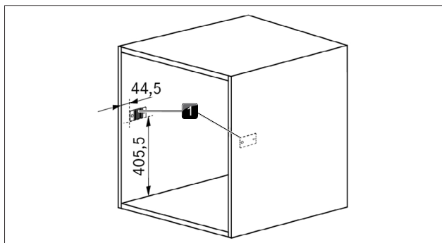
obr. 9.9 Montážní výklenek s aretační deskou korpusu
