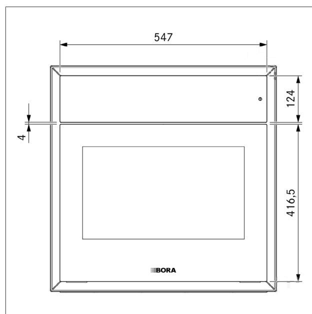
obr. 3.4 Pohled zepředu na sklo spotřebič XBO
