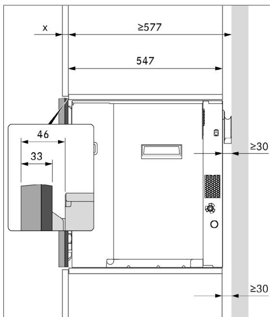
obr. 9.4 Montážní rozměry s 1 distančním rámem
