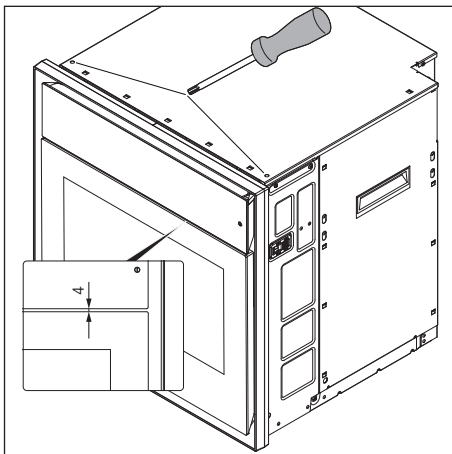
Obr. 9.14 Nastavení vzdálenosti ovládací jednotky a dvířek
