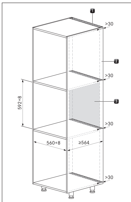
Obr. 9.1 Vestavná skříňka
