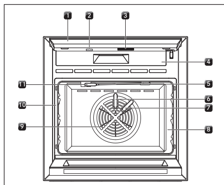
Obr. 5.1 Ovládací jednotka a otevírání dveří
