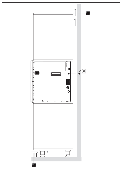
Obr. 9.16 Větrání
