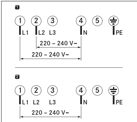
Obr. 9.13 Schéma připojení
