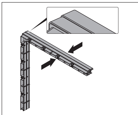
Obr. 9.7 2 prvky distančního rámu
