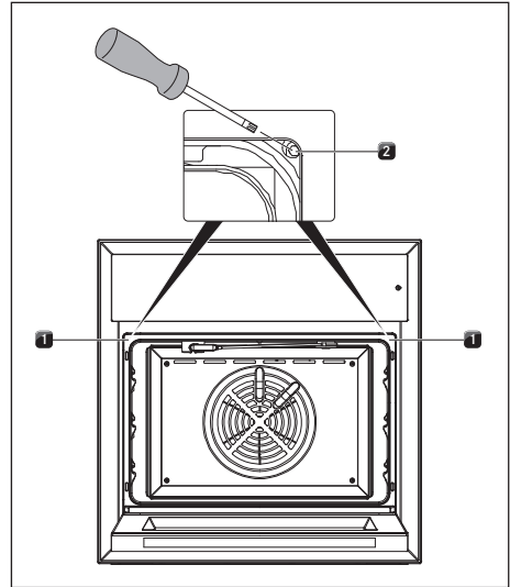
Obr. 9.15 Připevnění spotřebiče
