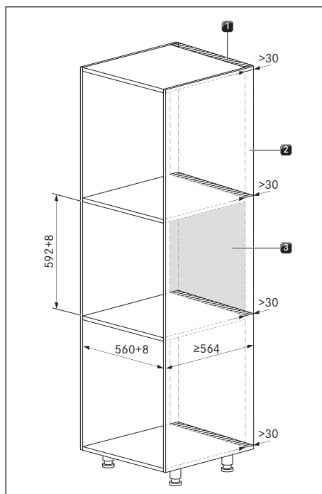
Obr. 9.1 Vestavná skříňka
