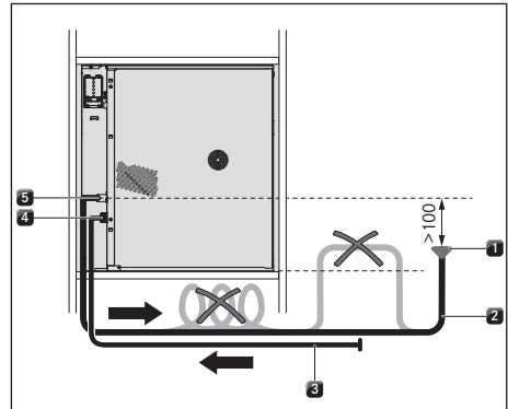
Obr. 9.11 Odvod vody
