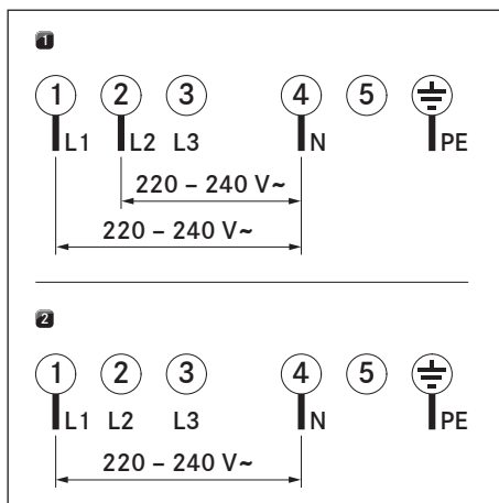
Obr. 9.13 Schéma připojení
