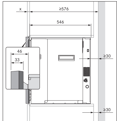
Obr. 9.4 Montážní rozměry s 1 distančním rámem
