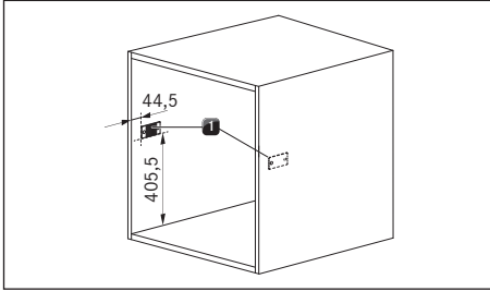
Obr. 9.9 Montážní výklenek s aretační deskou korpusu
