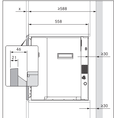
Obr. 9.3 Montážní rozměry bez distančního rámu
