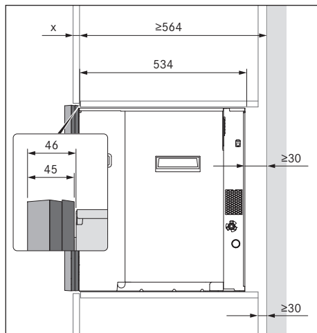
Obr. 9.5 Montážní rozměry se 2 distančními rámy
