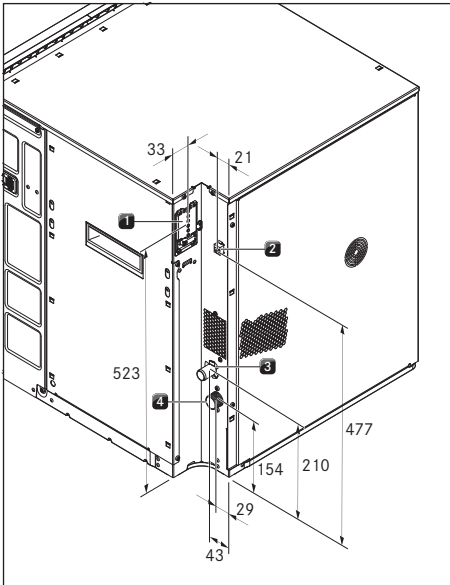
Obr. 9.10 Přípojky zařízení
