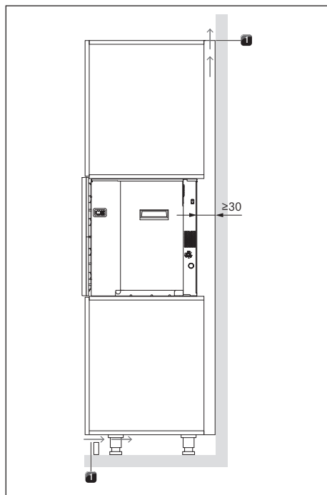
Obr. 9.16 Větrání
