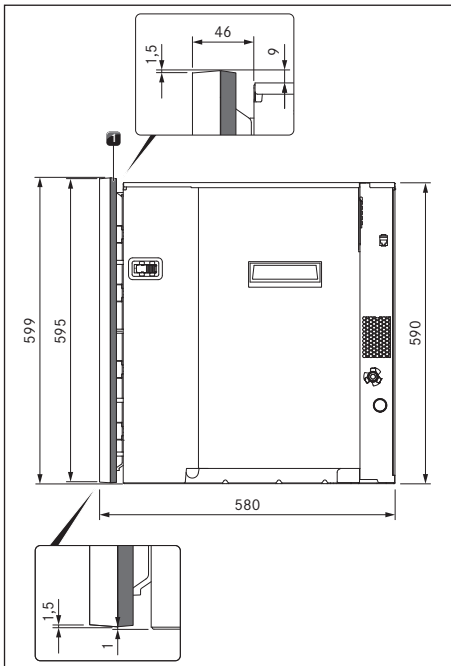
Obr. 9.2 Rozměry
