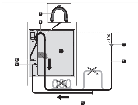
Obr. 9.12 Odvod vody přes přídržné kolínko
