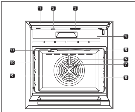
Obr. 5.1 Ovládací jednotka a otevírání dveří
