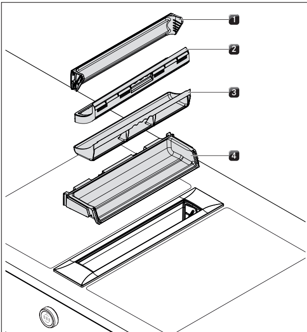
Afb. 4.7 Vetfiltercomponenten
