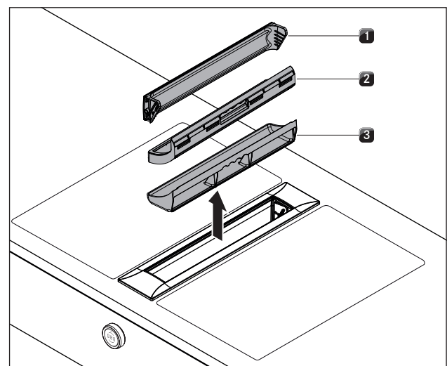
Afb. 8.1 Demontage van de vetfilteronderdelen
