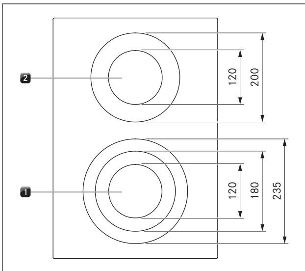
Afb. 4.11 Opbouw kookveld PKC3 en grootte van de kookzones
