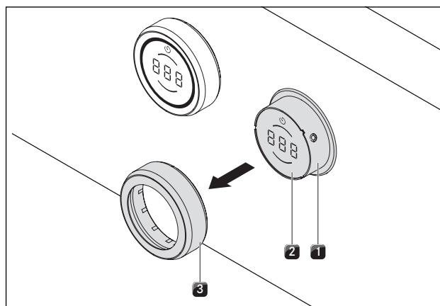
Afb. 8.6 Knopring verwijderen
