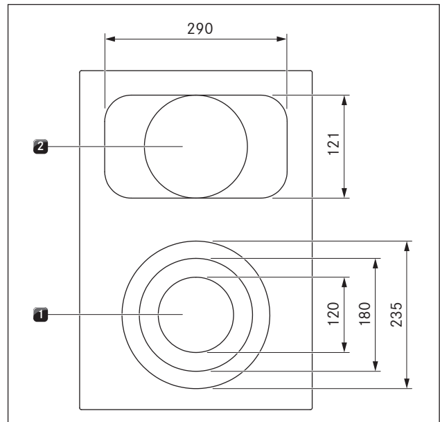
Afb. 4.12 Opbouw kookveld PKCB3 en grootte van de kookzones
