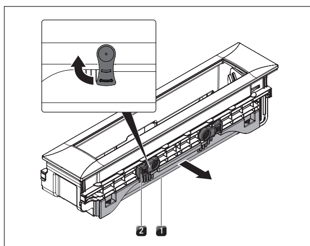
Afb. 8.4 Demontage van de onderhoudstank
