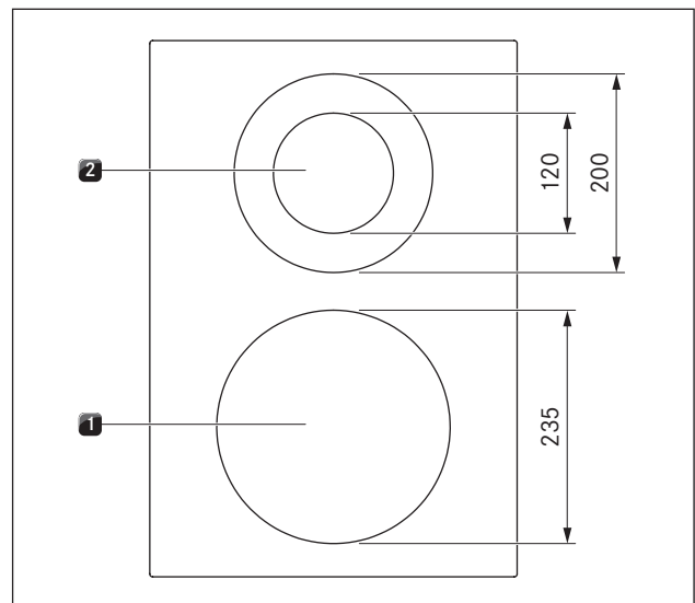
Afb. 4.13 Opbouw kookveld PKCH3 en grootte van de kookzones
