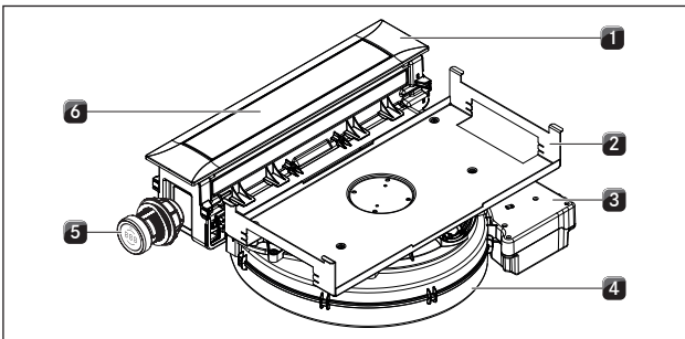
Afb. 4.6 Kookveldafzuigstelsysteem PKAS3/PKAS3AB
