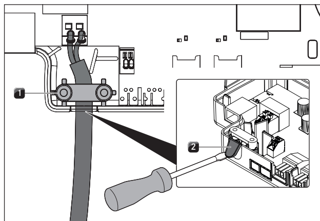
Afb. 4.47 Contact Home Out met trekcontlasting
