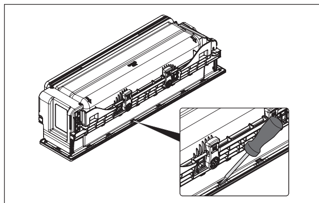
Afb. 4.23 Afdekframe demonteren
