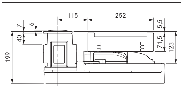
Afb. 3.6 PKAS3/PKAS3AB toestelafmetingen vooraanzicht
