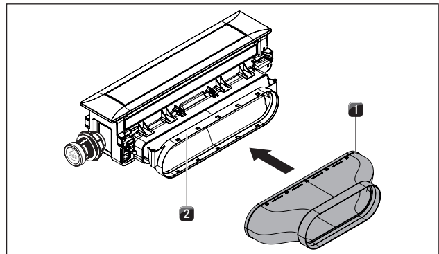
Afb. 4.20 Rechte kanaalstuk monteren
