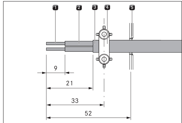
Afb. 4.42 Striplengtes en montagepositie van de aansluitkabel PKAS3/PKAS3AB - Home In
