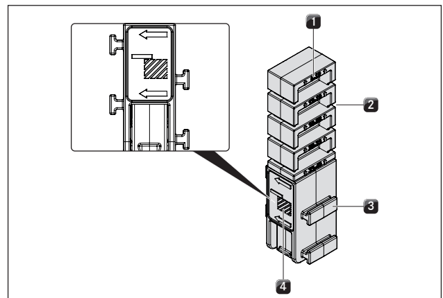
Afb. 4.29 Montageklem linkerzijde (opbouwmontage)
