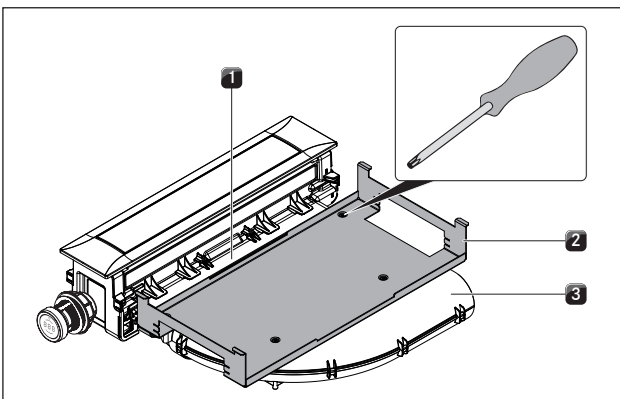
Afb. 4.18 Bevestigingsplaat verwijderen
