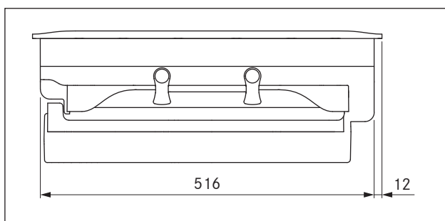
Afb. 3.7 PKAS3/PKAS3AB toestelafmetingen zijaanzicht
