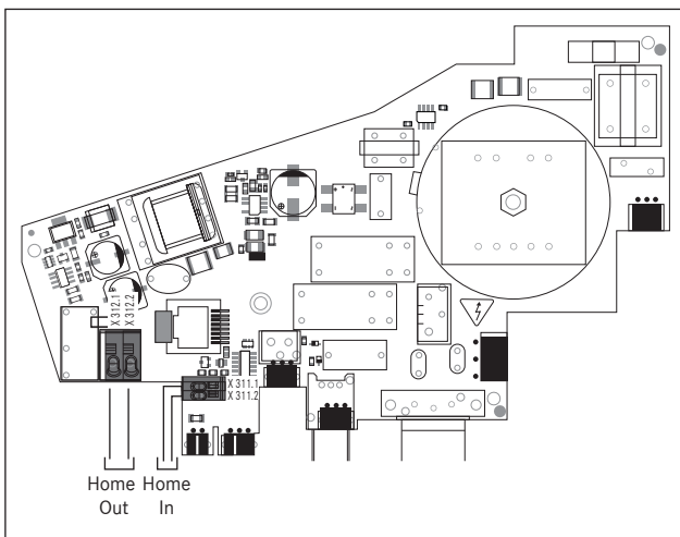
Afb. 4.45 Aansluitschema voor externe schakelcontacten PKAS3/PKAS3AB
