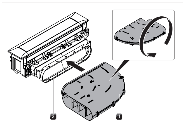
Afb. 4.21 Kanaalboogstuk draaien
