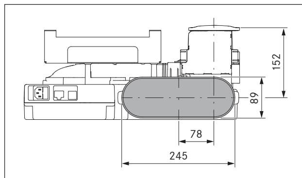
Afb. 4.35 Kanaalaansluitmaten PKAS3, PKAS3AB
