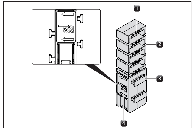
Afb. 4.28 Klem rechterzijde (vlakbouw)
