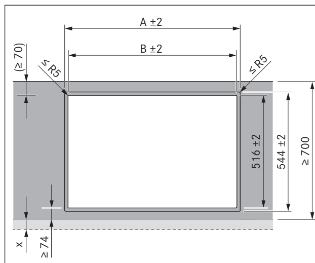
Afb. 4.7 Uitsparingsafmetingen in geval van vlinbouw
