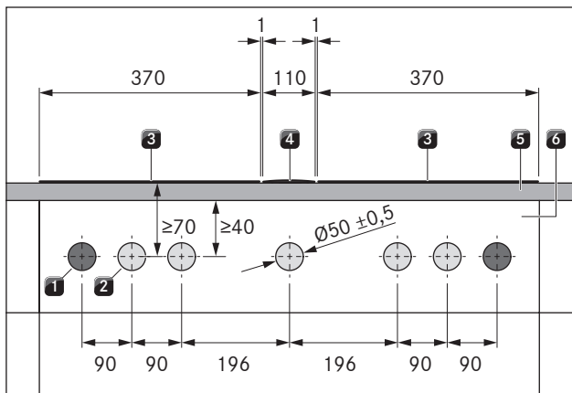
Afb. 4.13 Boorschema voor boorgaten in het paneel voor 2 kookvelden, 1 kookveldafzuiging en 2 stopcontacten
