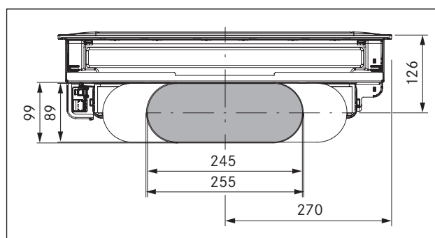
Afb. 4.33 Kanaalaansluitmaten PKA3/PKA3AB met het rechte kanaalstuk
