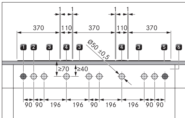
Afb. 4.14 Boorschema voor boorgaten in het paneel voor 3 kookvelden, 2 kookveldafzuigingen en 2 stopcontacten
