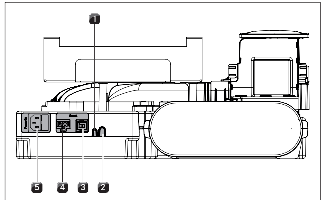
Afb. 4.51 Aansluitingen aan de achterzijde PKAS3 en PKAS3AB
