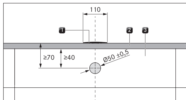
Afb. 4.12 Boorschema voor boorgaten in het paneel voor de kookveldaafzuiging
