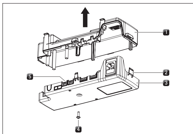
Afb. 4.40 Behuizingsdeksel van de besturingseenheid openen
