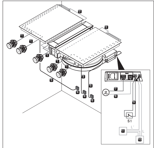
Afb. 4.57 Aansluitschema PKAS3/PKAS3AB
