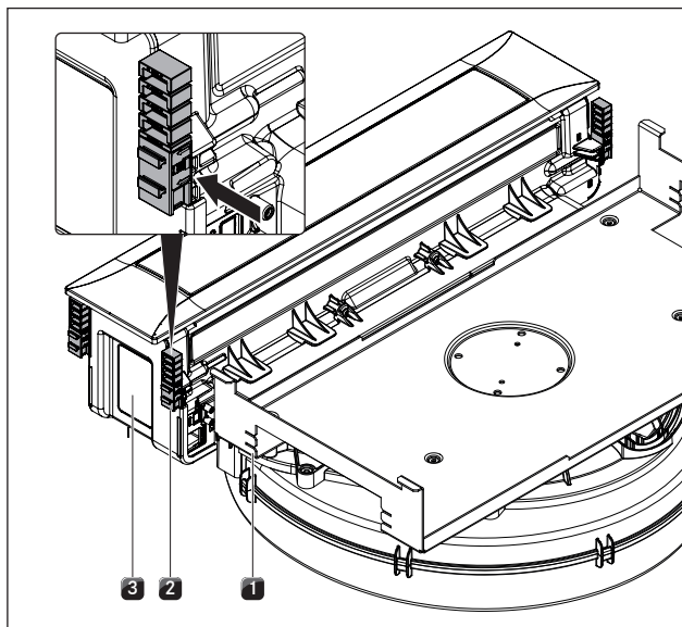
Afb. 4.30 De klemmen eroverheen schuiven
