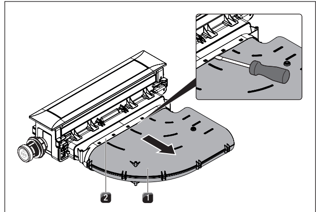
Afb. 4.19 Demonteer het kanaalboogstuk.
