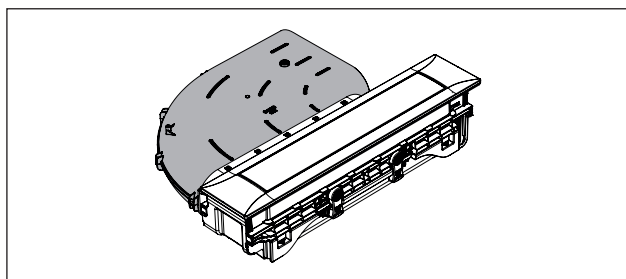
Afb. 4.22 Luchtgeleiding naar links met kanaalboogstuk
