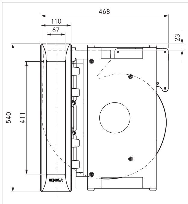
Afb. 3.5 PKAS3/PKAS3AB toestelafmetingen bovenaanzicht
