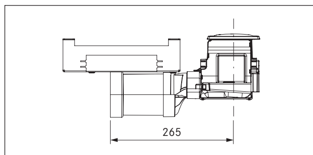
Afb. 4.34 Kanaalaansluitmaten PKA3/PKA3AB met het rechte kanaalstuk
