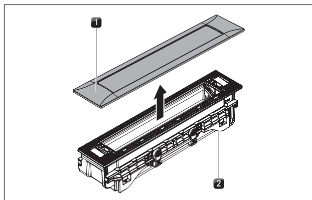
Afb. 4.24 Afdekframe demonteren
