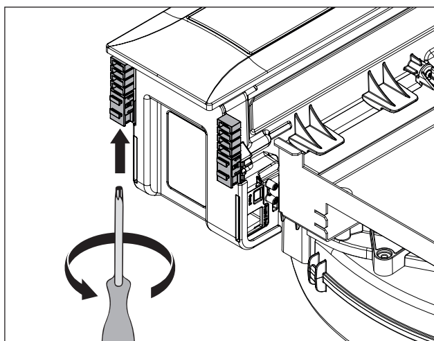
Afb. 4.31 De klemmen aandraaien
