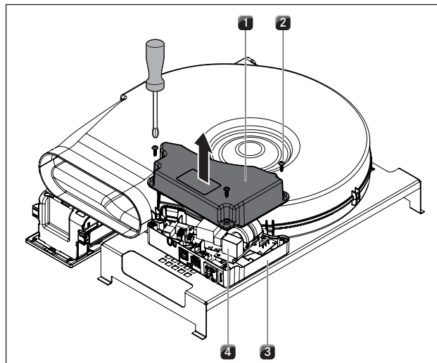
Afb. 4.39 Behuizingsdeksel van de besturingseenheid openen
