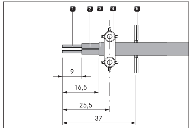
Afb. 4.43 Striplengtes en montagepositie van de aansluitkabel PKAS3/PKAS3AB - Home Out
