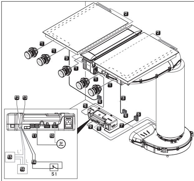
Afb. 4.56 Aansluitschema PKA3/PKA3AB
