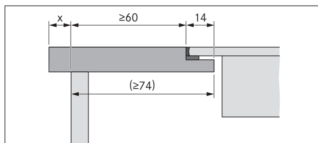
Afb. 4.6 Uitstekend deel van het werkblad
