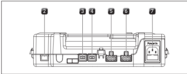
Afb. 4.53 Aansluitingen van de besturingseenheid
