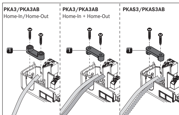
Afb. 4.48 Montage van de trekcontlastingsklem
