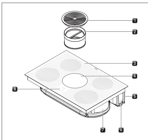
Ilustracja 4.1 Płyta grzewcza
