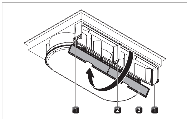
Ilustracja 5.12 Otwieranie pokrywy obudowy
