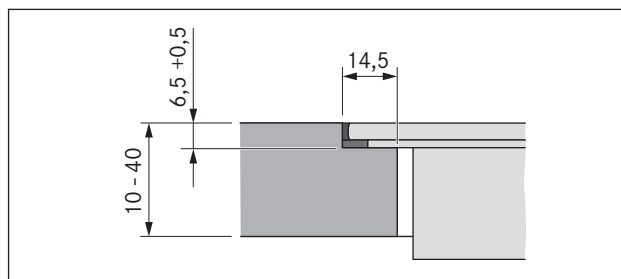
Ilustracja 5.7 Wielkość zakładki przy montażu z zachowaniem równej powierzchni
