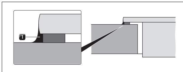
Ilustracja 5.24 Masa silikonowa przy montażu elementu z uskokiem
