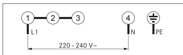
Ilustracja 5.22 Schemat podłączenia, przyłącze 1-fazowe
