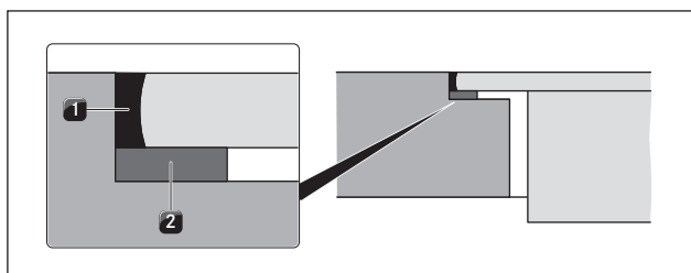
Ilustracja 5.11 Taśma uszczelniająca przy montażu z zachowaniem równej powierzchni
