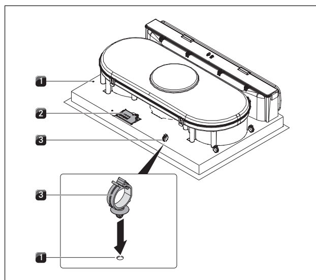
Ilustracja 5.23 Przyłącza elektryczne płyty grzewczej
