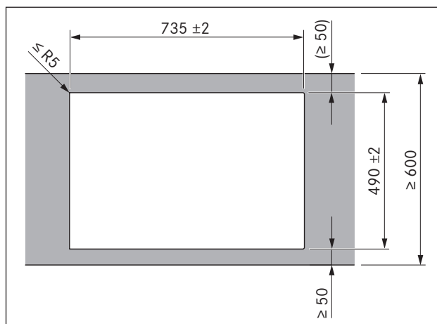
Ilustracja 5.8 Wymiary wycięcia dla montażu elementu z uskokiem
