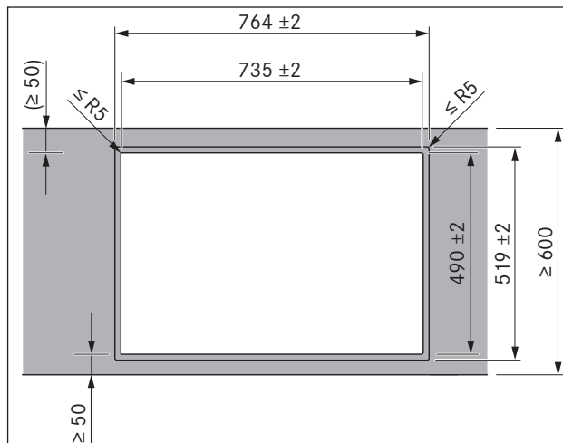
Ilustracja 5.6 Wymiary wycięcia dla montażu z zachowaniem równej powierzchni
