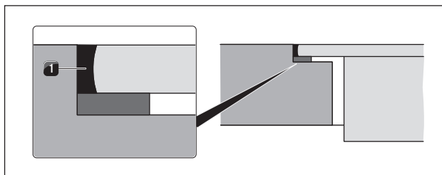
Ilustracja 5.25 Masa silikonowa przy montażu z zachowaniem równej powierzchni
