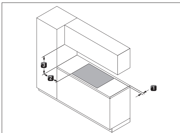
Ilustracja 5.1 Minimalne odstępów
