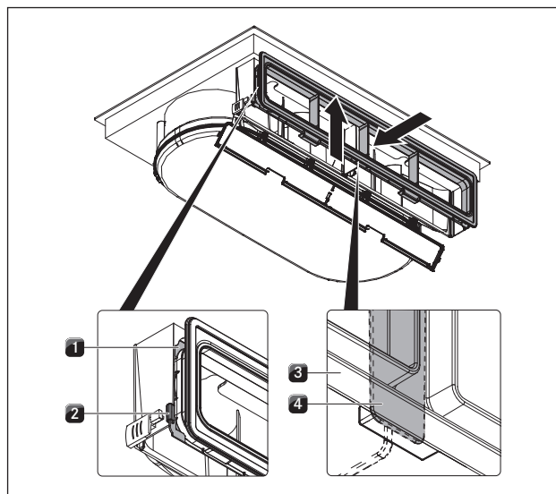
Ilustracja 5.13 Zawieszanie ramy kanału elastycznego
