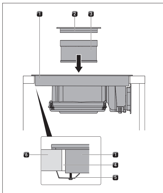
Ilustracja 5.18 Centralne mocowanie płyty grzewczej
