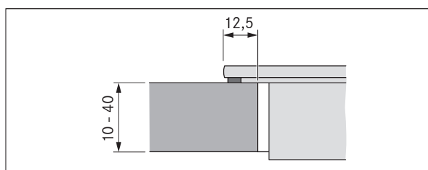
Ilustracja 5.9 Wymiary podparcia dla montażu elementu z uskokiem
