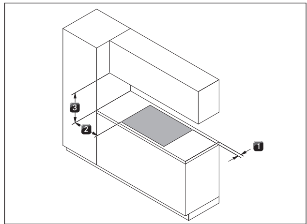
Abb. 5.1 Mindestabstände
