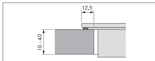
SI. 5.9 Dimenzije prirobnice za nasadno montažo
