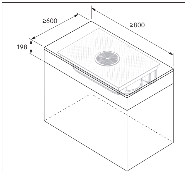
SI. 5.2 Najmanjše dimenzije povišča GP4U
