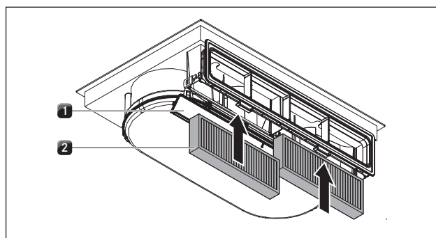
Sl. 5.14 Vstavljanje filtra z aktivnim ogljem
