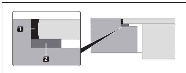
Sl. 5.11 Trak za tesnjenje pri montaži v isti ravnini s površino
