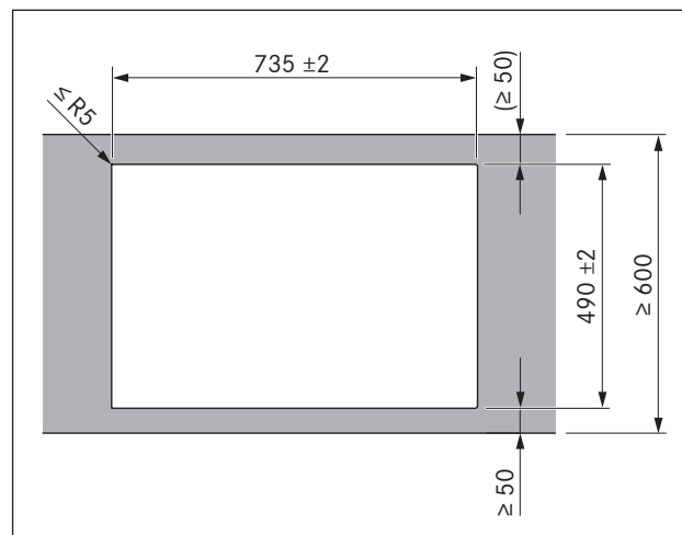
SI. 5.8 Dimenzije izreza za nasadno montažo
