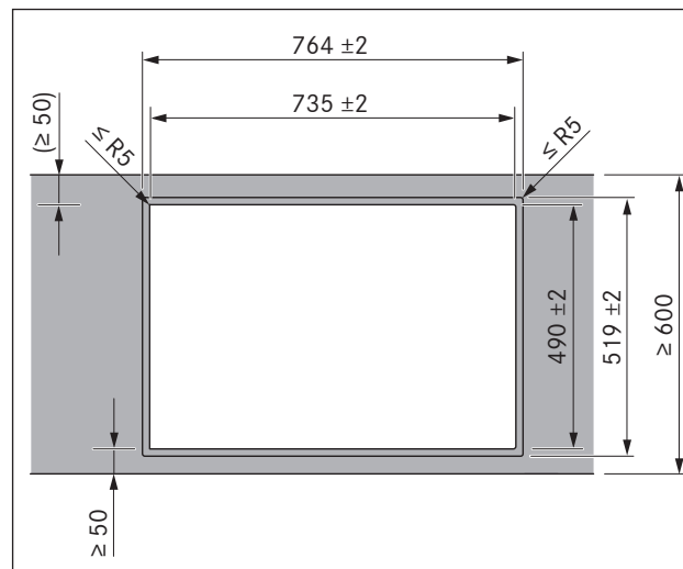
SI. 5.6 Dimenzije izreza za montažo v isti ravnini s površino
