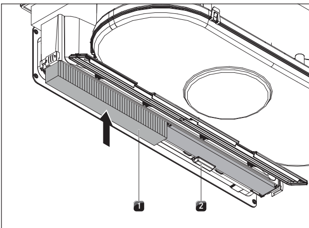
SI. 7.9 Vstavljanje filtra z aktivnim ogljem
