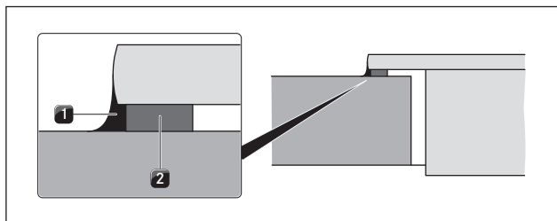
Sl. 5.10 Trak za tesnjenje pri nasadni montaži
