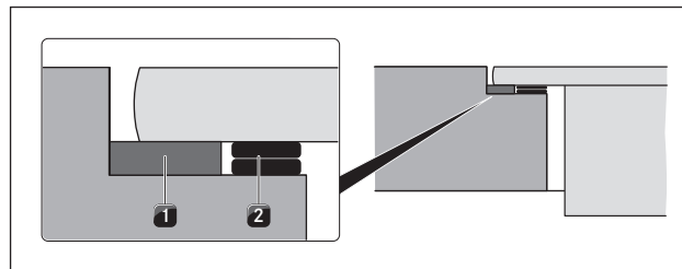
SI. 5.17 Plošče za izravnavo višine
