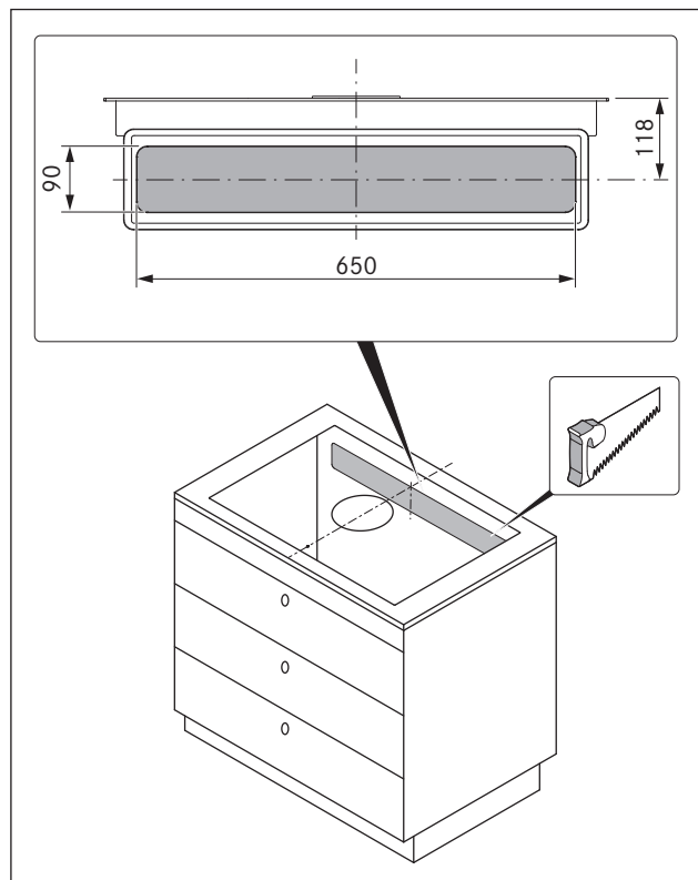
SI. 5.5 Izrez zadnje strani
