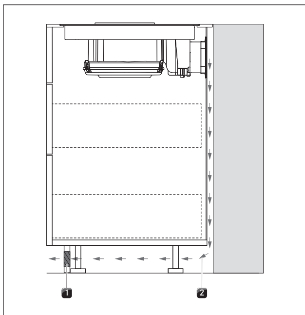
SI. 5.3 Odprtina za povratni tok v območju vtiča
