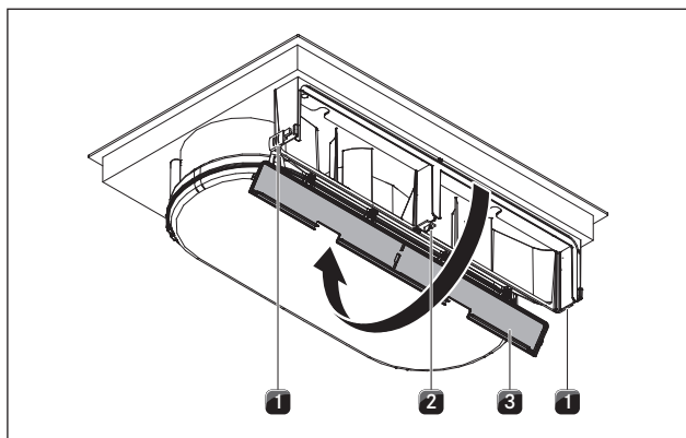
Sl. 5.12 Odpiranje pokrova ohišja
