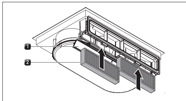
Prikaz 5.14 Umetanje filtra s aktivnim ugljenom
