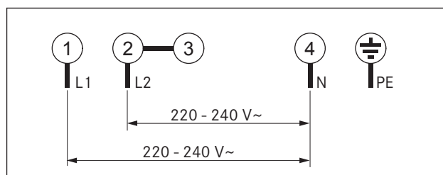
Prikaz 5.21 Priključna shema za dvofazni priključak
