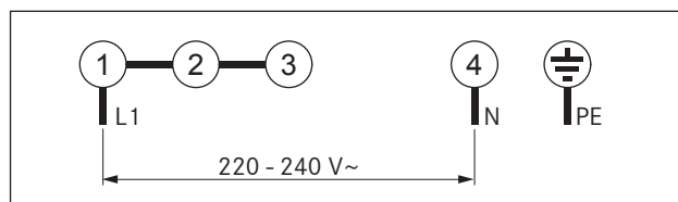
Prikaz 5.22 Priključna shema za jednofazni priključak
