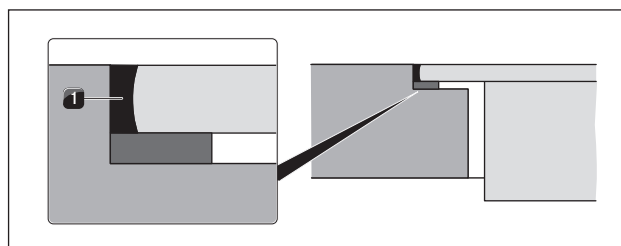
Prikaz 5.25 Silikonska masa za brtvljenje kod montaže u ravni s površinom
