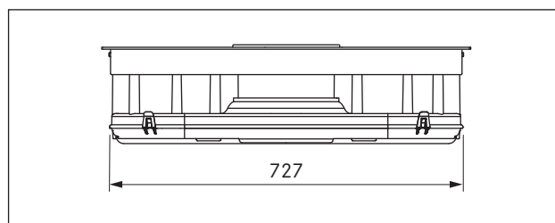
Prikaz 3.2 GP4U dimenzije uređaja, prikaz srijeda
