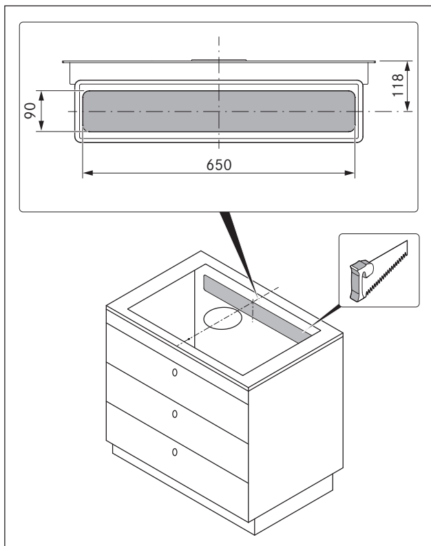
Prikaz 5.5 Izrez u stražnjoj stranici
