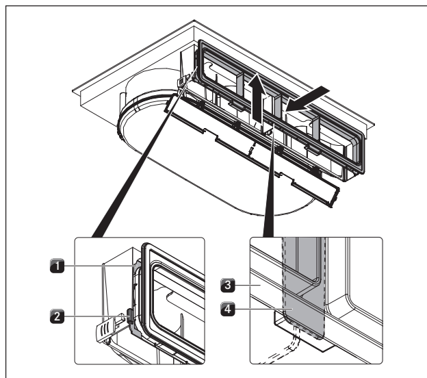
Prikaz 5.13 Vješanje okvira fleksibilnog kanala
