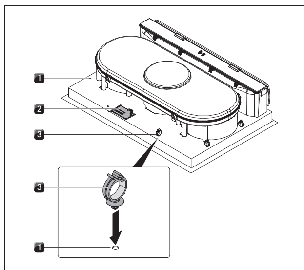
Prikaz 5.23 Električni priključci ploče za kuhanje
