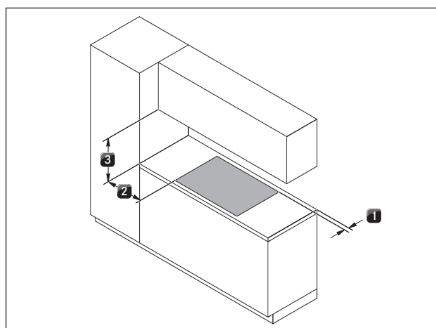
Prikaz 5.1 Minimalne udaljenosti
