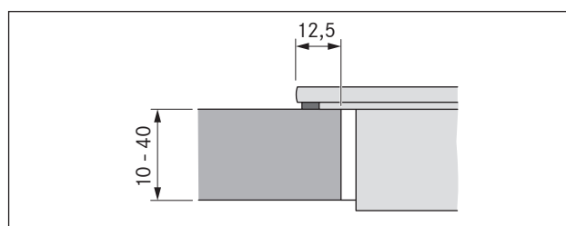
Prikaz 5.9 Dimenzija polaganja za montažu na površinu
