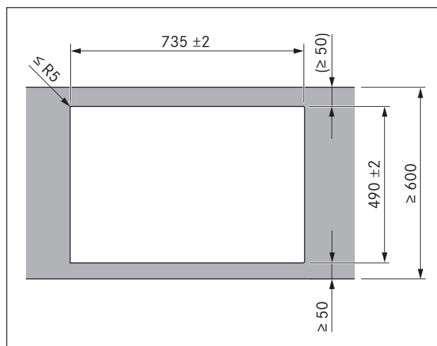
Prikaz 5.8 Dimenzije izreza za montažu na površinu
