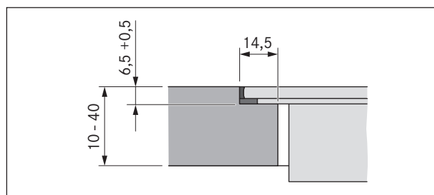
Prikaz 5.7 Dimenzije pregiba za montažu u ravnini s površinom
