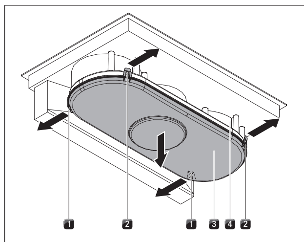
Fig. 12.3 Ouverture du boîtier de circulation de l'air
