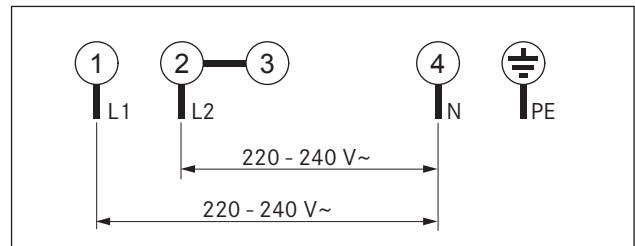
Fig. 5.22 Schéma de raccordement biphasé
