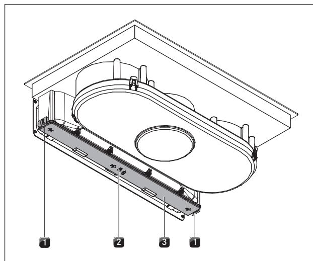
Fig. 12.5 Déverrouillage du couvercle du boîtier des filtres à charbon actif
