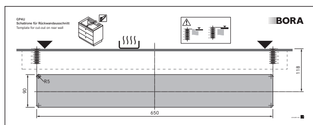
Fig. 5.6 Gabarit de découpe dans la paroi arrière
