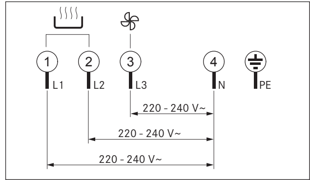
Fig. 5.21 Schéma de raccordement triphasé
