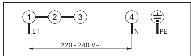
Fig. 5.23 Schéma de raccordement monophasé
