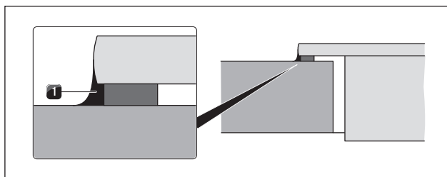
Fig. 5.25 Joint en silicone en montage en saillie
