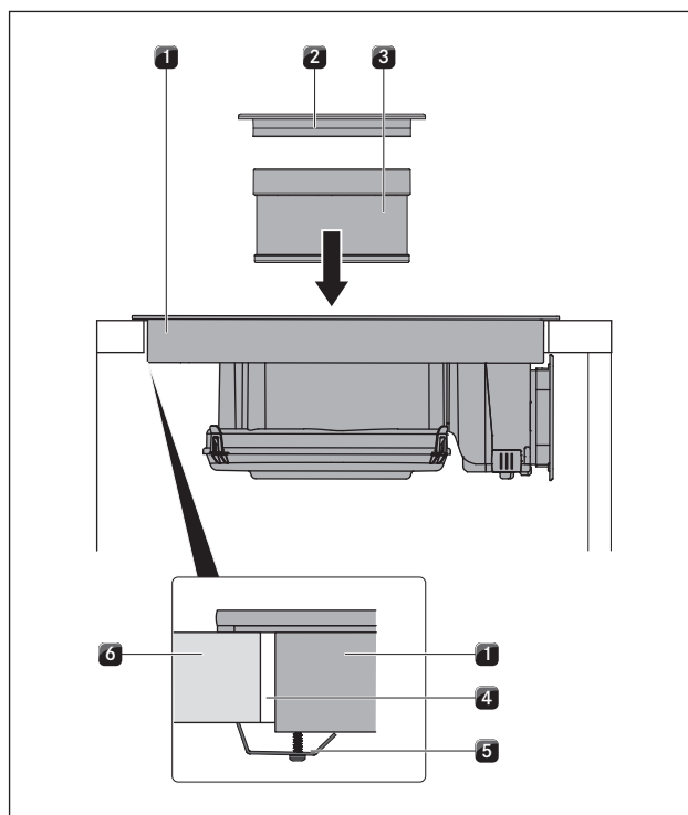
Fig. 5.19 Centrage et fixation de la table de cuisson
