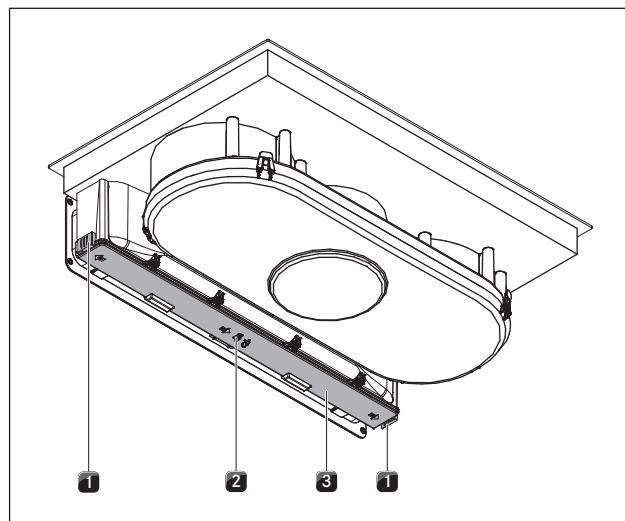
Fig. 7.5 Desbloquear la tapa de la carcasa del filtro de carbón activo
