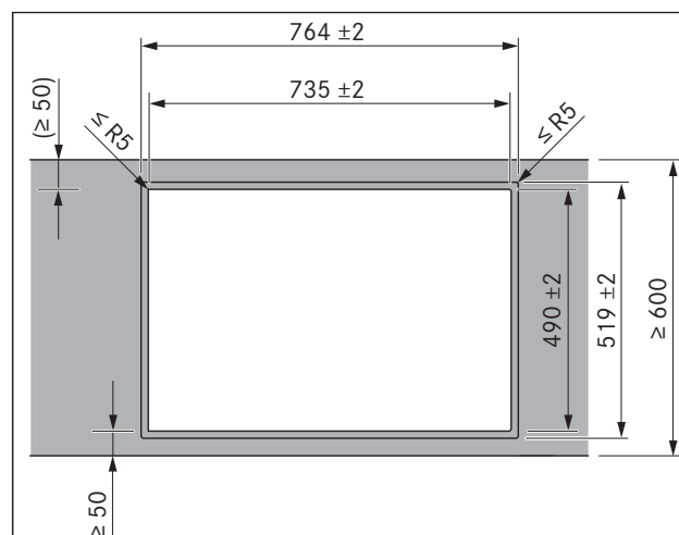
Fig. 5.6 Medidas del recorte para montaje enrasado
