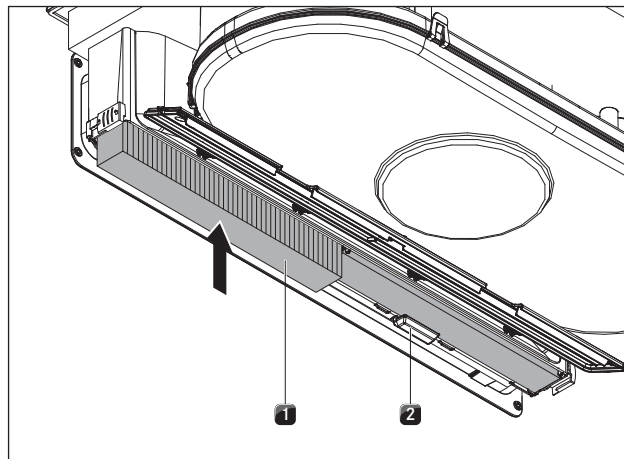
Fig. 7.9 Colocación de los filtros de carbón activo
