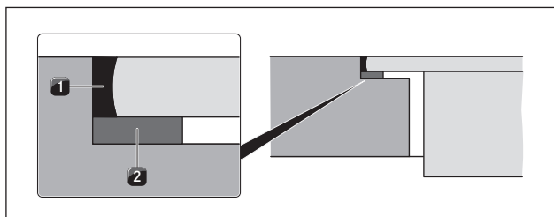
Fig. 5.11 Cinta selladora para montaje enrasado
