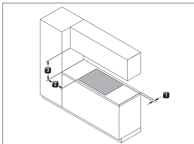
Fig. 5.1 Distancias mínimas
