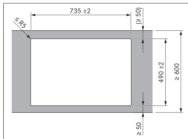
Fig. 5.8 Medidas del recorte para montaje superpuesto
