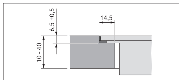
Fig. 5.7 Medida del pliegue para un montaje enrasado
