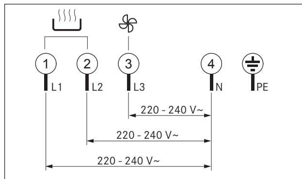
Fig. 5.20 Esquema de conexiones, conexión trifásica
