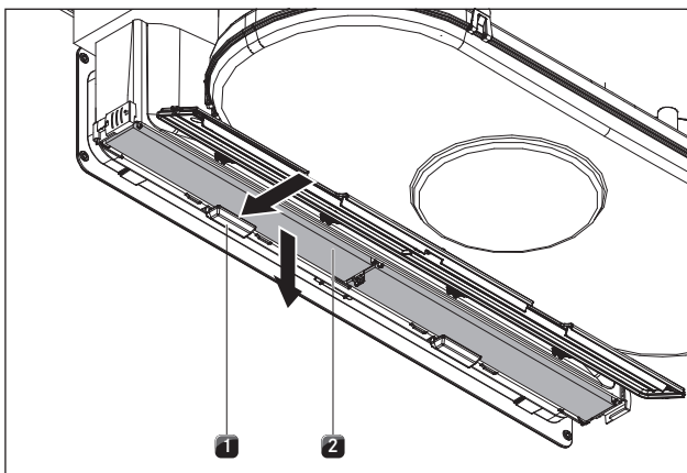
Fig. 7.8 Desmontar el filtro de carbón activo
