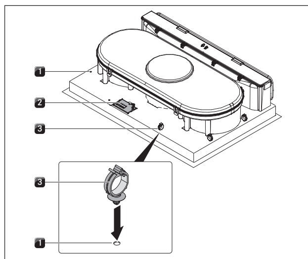
Fig. 5.23 Conexiones eléctricas de la placa de cocción
