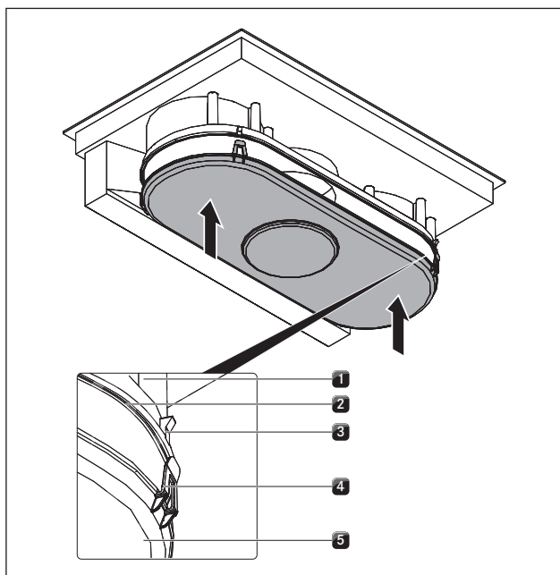
Fig. 7.4 Cierre de la carcasa de conducción del aire
