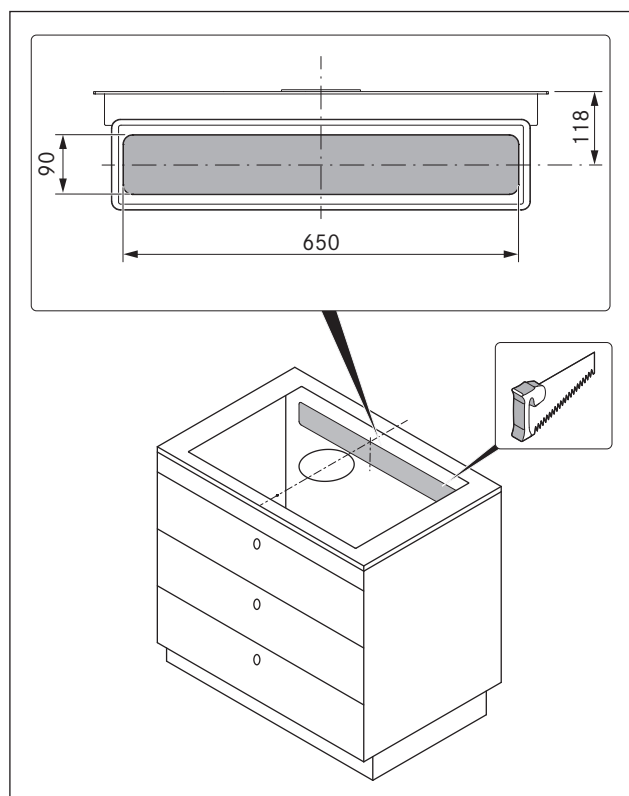
Fig. 5.5 Recorte del panel trasero
