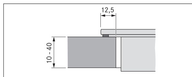
Fig. 5.9 Dimensiones para montaje superpuesto
