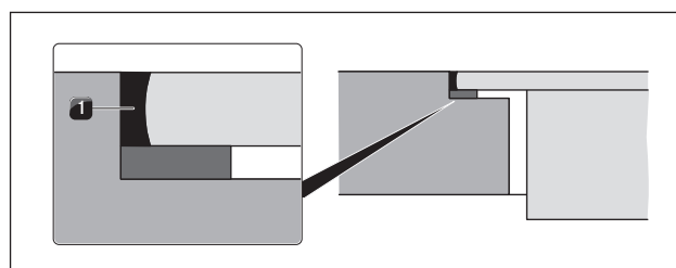
Fig. 5.25 Silicona de sellado para montaje enrasado
