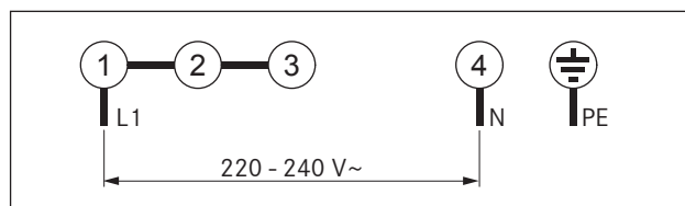
Fig. 5.22 Esquema de conexiones, conexión monofásica
