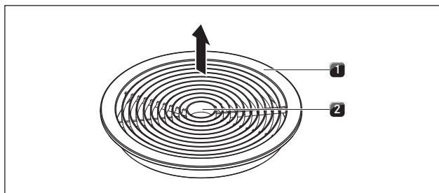
Fig. 7.1 Desmontaje de la tobera de entrada
