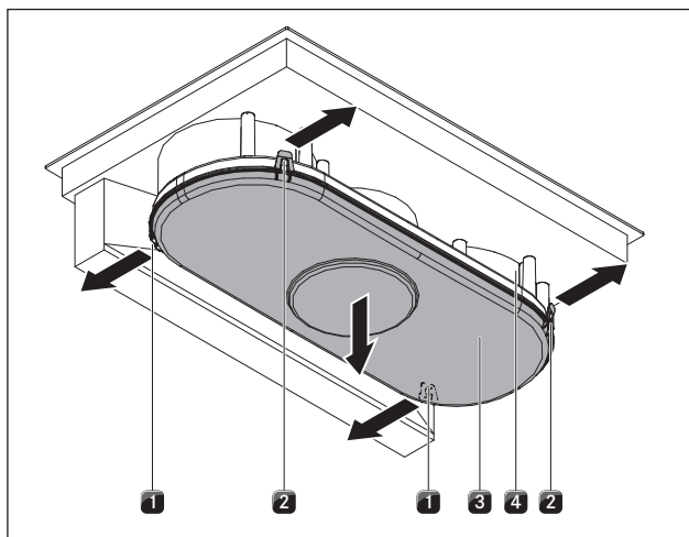
Fig. 7.3 Apertura de la carcasa de conducción del aire
