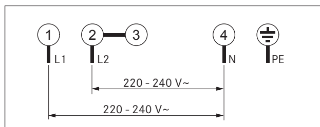
Fig. 5.21 Esquema de conexiones, conexión bifásica
