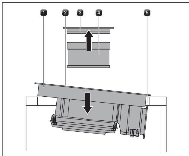
Fig. 5.15 Colocación de la placa de cocción
