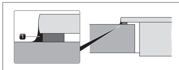
Fig. 5.24 Silicona de sellado para montaje superpuesto
