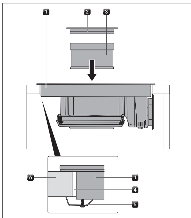
Fig. 5.18 Fijación de la placa de cocción en posición centrada
