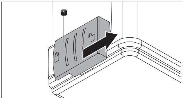
Fig. 7.6 Abrir los bloqueos exteriores
