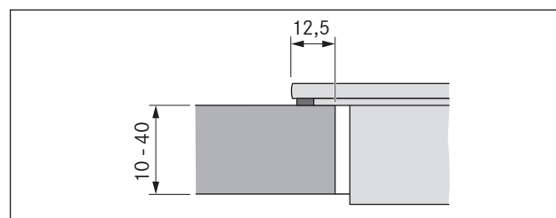
Obr. 5.10 Rozměry podkladu pro montáž na povrch
