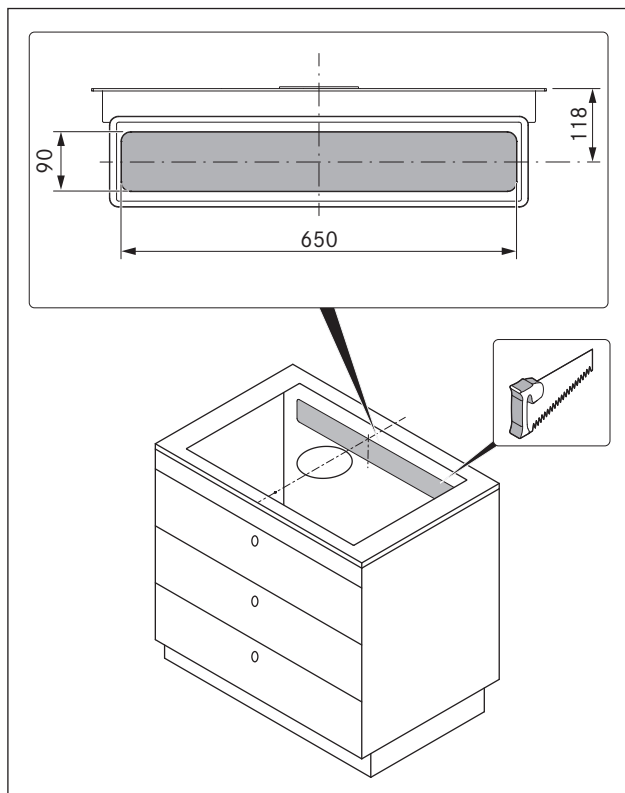
Obr. 5.5 Výřez v zadní stěně
