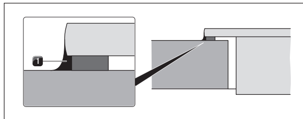
Obr. 5.25 Silikonová těsnicí hmota při montáži na povrch
