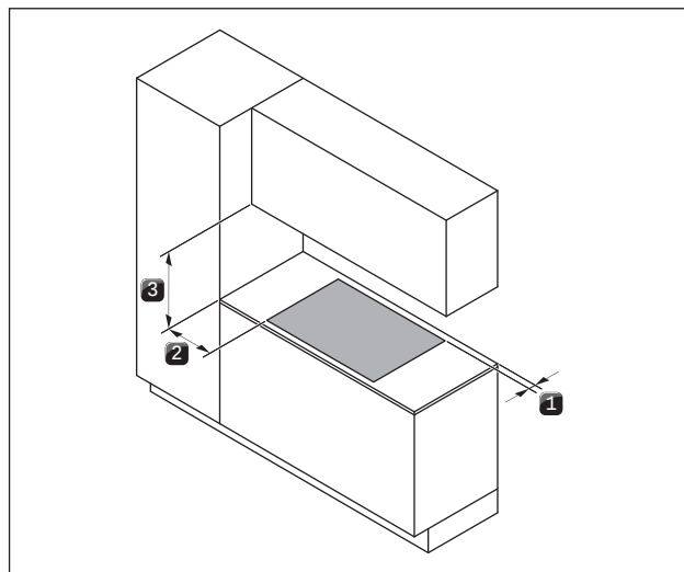
Obr. 5.1 Minimální vzdálenosti
