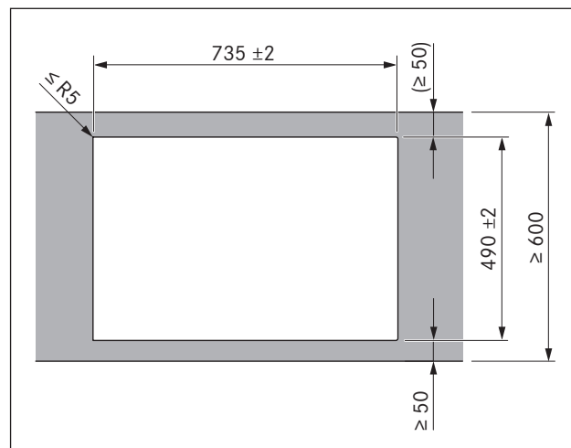
Obr. 5.9 Rozměry výřezu pro montáž na povrch
