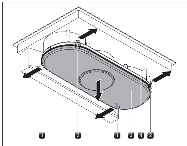
Obr. 7.3 Otevření skříně ventilace
