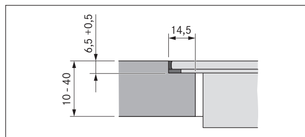
Obr. 5.8 Rozměr drážky pro plošně zarovnanou montáž
