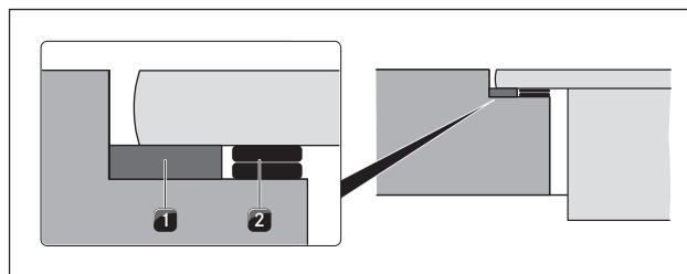
Obr. 5.18 Podložky k nastavení výšky
