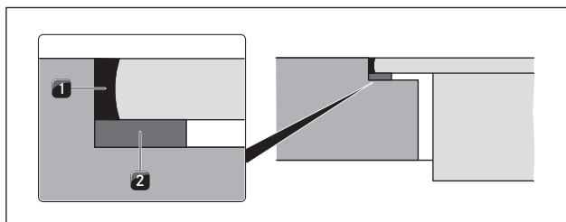
Obr. 5.12 Těsnící páska při plošně zarovnané montáži
