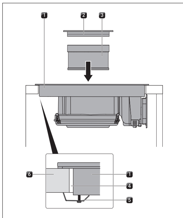
Obr. 5.19 Upevnění varné desky do středu
