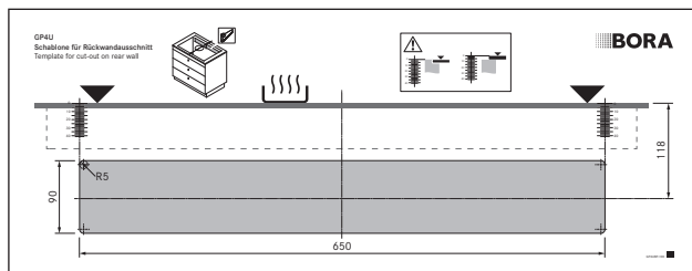
Obr. 5.6 Šablona pro výřez zadní stěny
