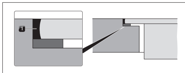
Obr. 5.26 Silikonová těsnicí hmota při plošně zarovnané montáži
