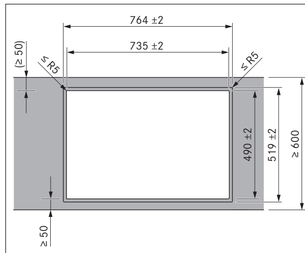
Obr. 5.7 Rozměry výřezu pro plošně zarovnanou montáž
