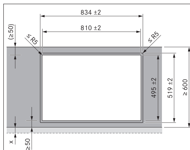
Sl. 8.7 Dimenzije izreza za montažo v isti ravnini s površino
