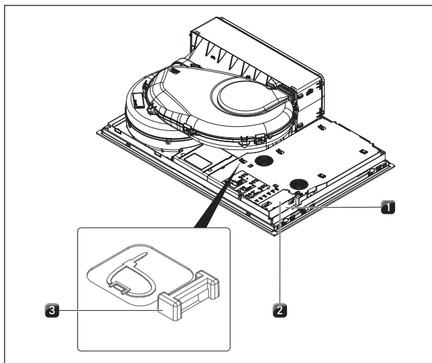
Sl. 8.50 Električni priključki kuhalne plošče
