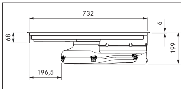
SI. 5.11 Dimenzije naprave PURU, pogled od spredaj
