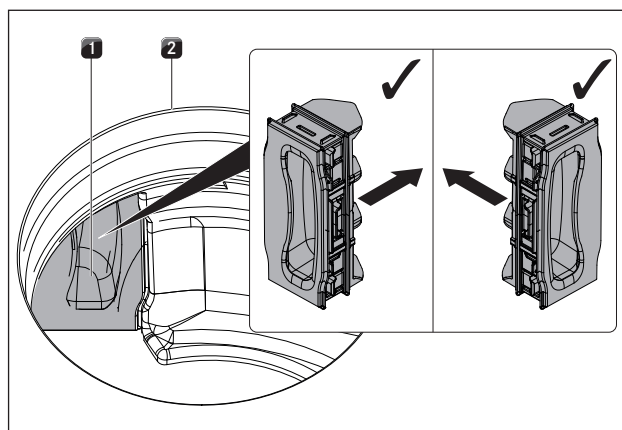
SI. 8.45 Vstavljanje lopute za zamenjavo filtra
