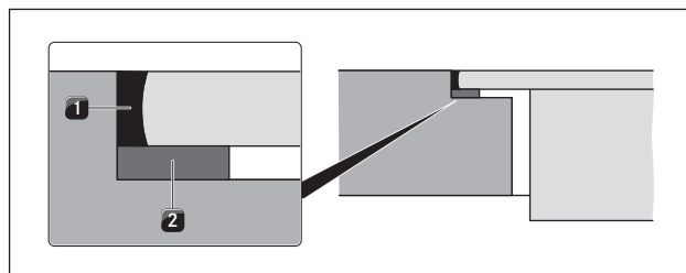
SI. 8.32 Trak za tesnjenje pri montaži v isti ravnini s površino
