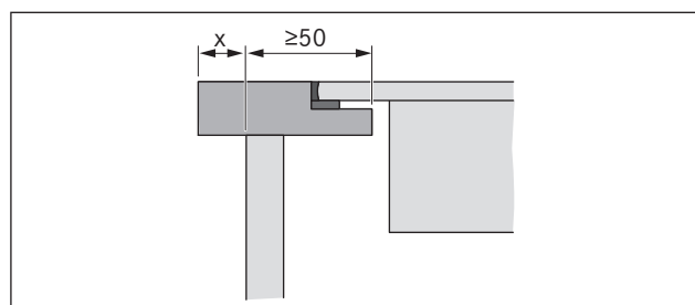
Sl. 8.6 Previs delovne plošče
