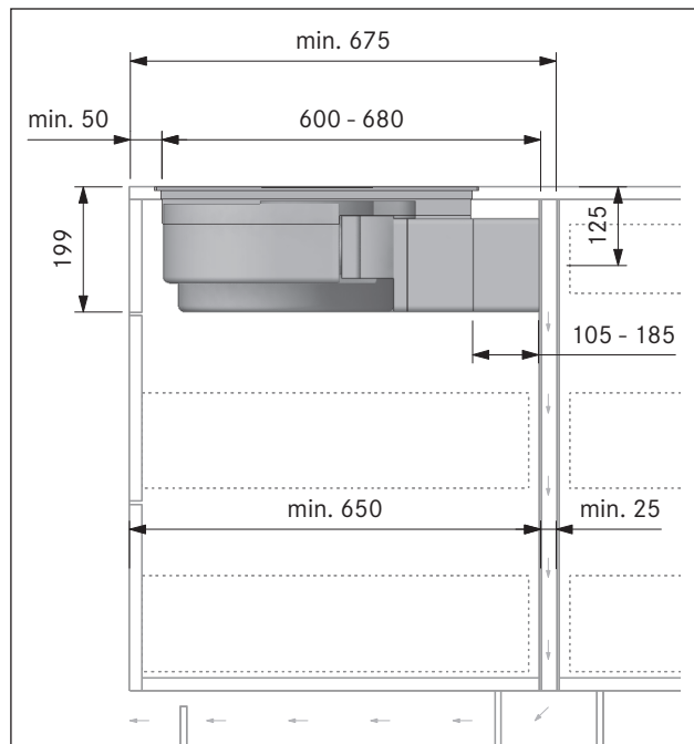
SI. 8.34 Dimenzije vgradnje pri različici montaže A z obtočnim zrakom, globina delovne plošče od 675 mm
