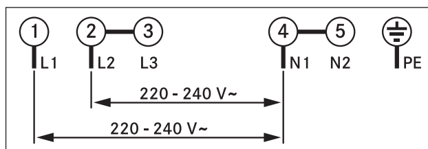
Sl. 8.48 Priključna shema dvofaznega priključka
