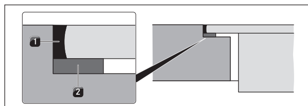
Sl. 8.17 Trak za tesnjenje pri montaži v isti ravnini s površino
