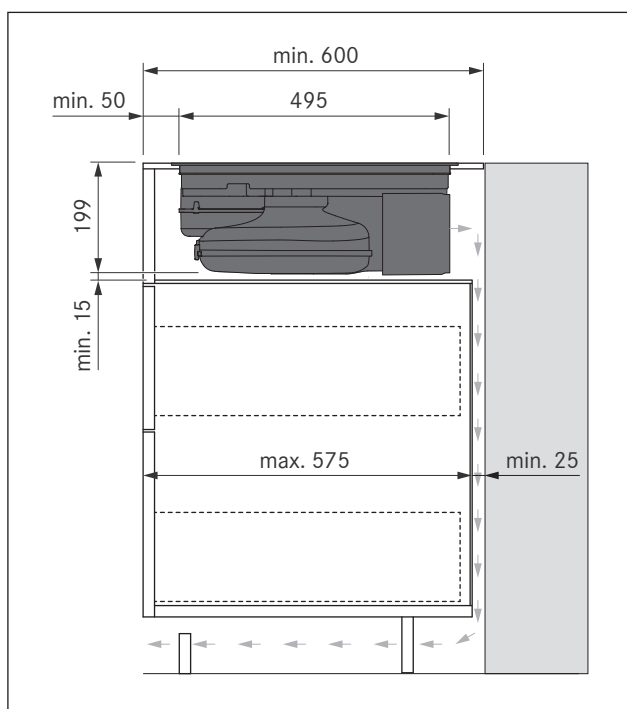
SI. 8.30 Dimenzije vgradnje pri različici montaže B z obtočnim zrakom, globina delovne plošče 600 mm
