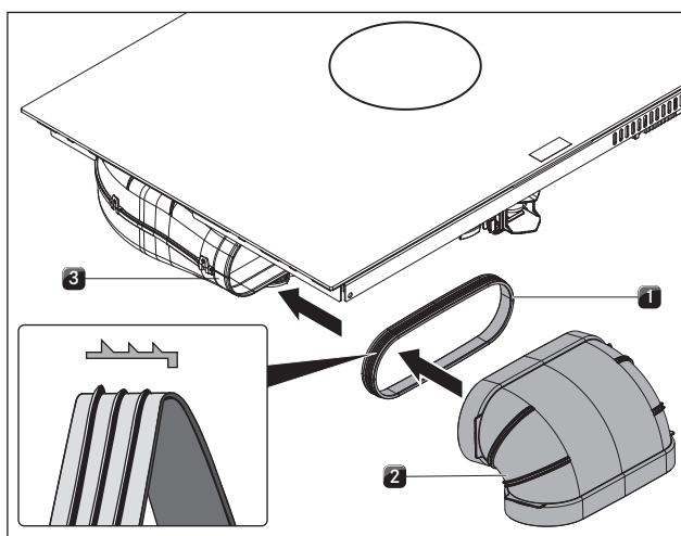
SI. 8.23 Priključitev na sistem kanala
