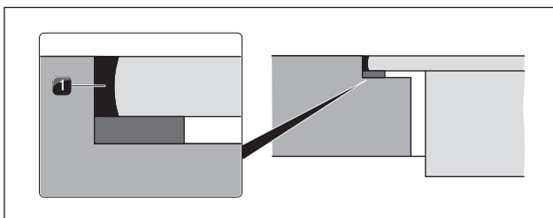
Sl. 8.56 Silikonska tesnilna masa pri montaži v isti ravnini s površino
