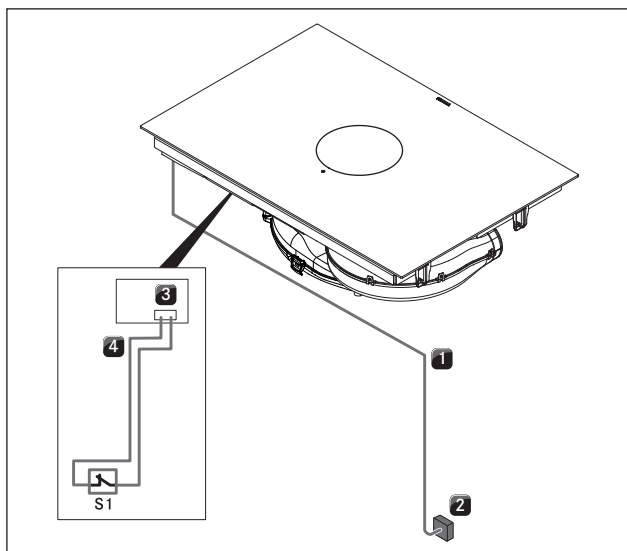
Sl. 8.46 Priključna shema z izbirnim modulom Home-In Modul
