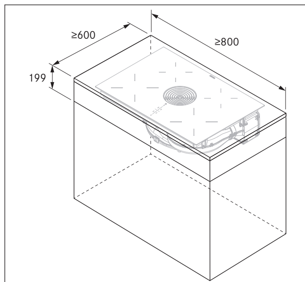
Sl. 8.5 Najmanjše dimenzije pohištva Pure
