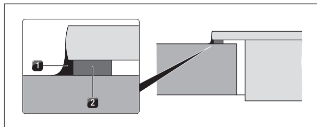
SI. 8.31 Trak za tesnjenje pri nasadni montaži
