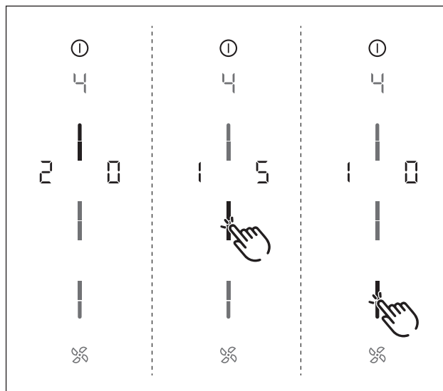
SI. 9.5 Točka menija 4: Trajanje avtomatike za nadaljnje kuhanje
