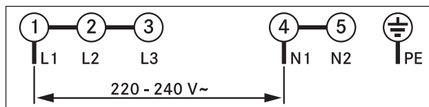
Sl. 8.49 Priključna shema enofaznega priključka
