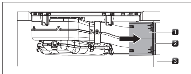
SI. 8.40 Priključek zadnje strani
