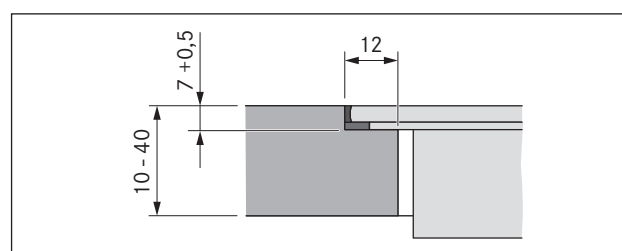
Sl. 8.8 Pregibna mera za montažo v isti ravnini s površino
