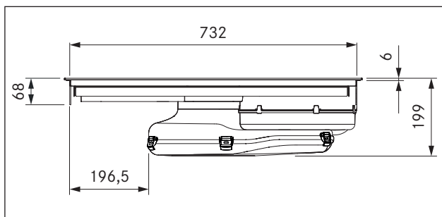
SI. 5.8 Dimenzije naprave PURA, pogled od spredaj
