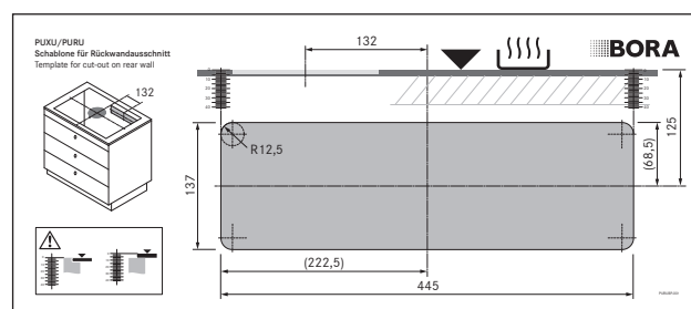
Sl. 8.29 Šablona za izrez zadnje strani
