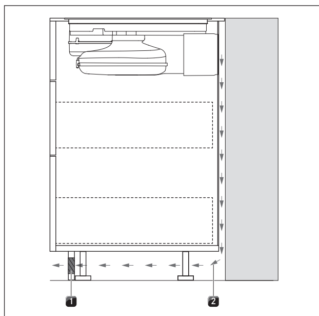
SI. 8.24 Odprtina za povratni tok v območju vtiča
