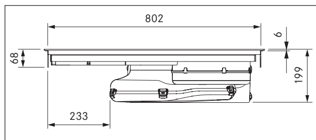
SI. 5.5 Dimenzije naprave PUXU, pogled od spredaj
