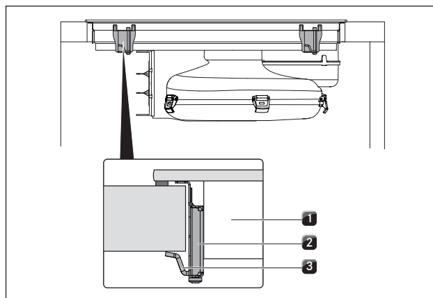
SI. 8.22 Sredinsko pritrdjevanje kuhalne plošče
