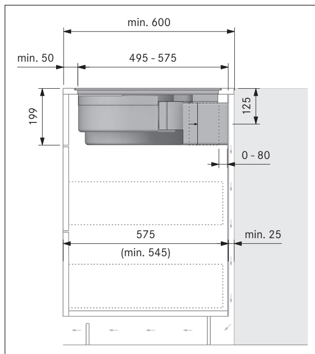
Sl. 8.27 Dimenzije vgradnje pri obtočnem zraku, različica montaže A
