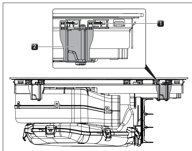
Sl. 8.18 Namestitev montažnih sponk
