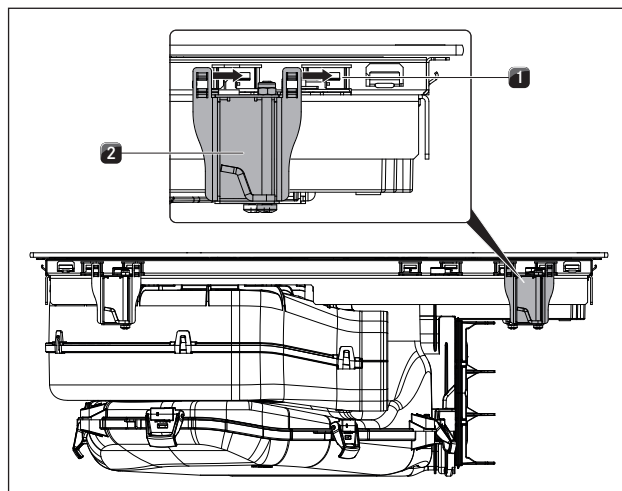
SI. 8.33 Namestitev montažnih sponk
