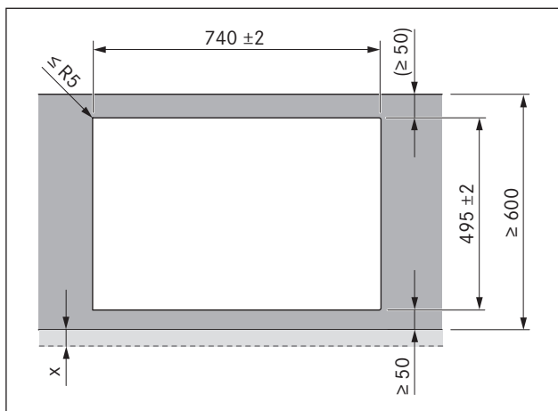
SI. 8.13 Dimenzije izreza za nasadno montažo
