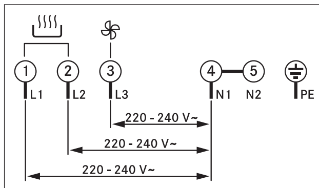
Sl. 8.47 Priključna shema trifaznega priključka
