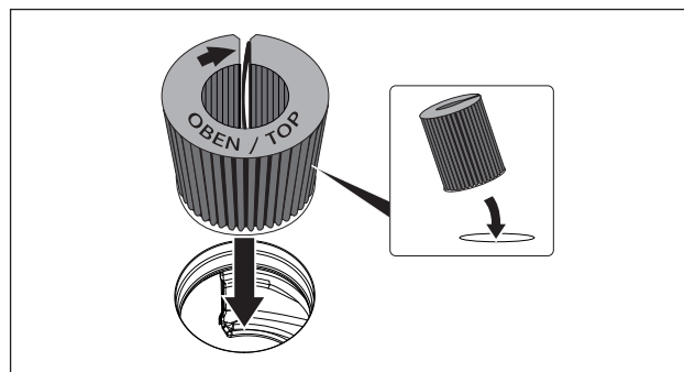
SI. 8.43 Vstavljanje filtra z aktivnim ogljem v odprtino za odvod zraka
