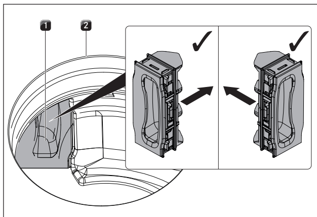
SI. 10.11 Vstavljanje lopute za zamenjavo filtra
