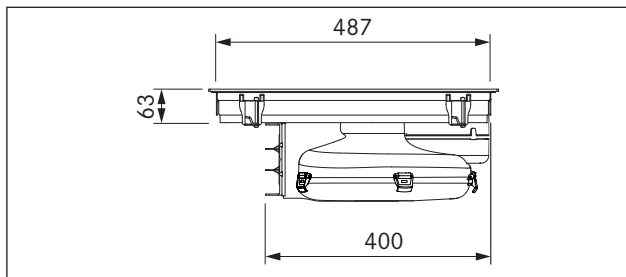
SI. 5.9 Dimenzije naprave PURA, pogled s strani
