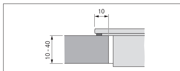
Sl. 8.10 Dimenzije prirobnice za nasadno montažo
