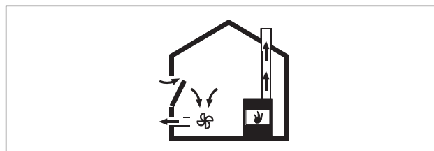
Sl. 8.2 Montaža odvoda zraka – pravilno
