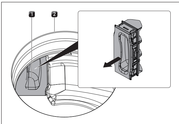
SI. 10.5 Odstranitev lopute za zamenjavo filtra
