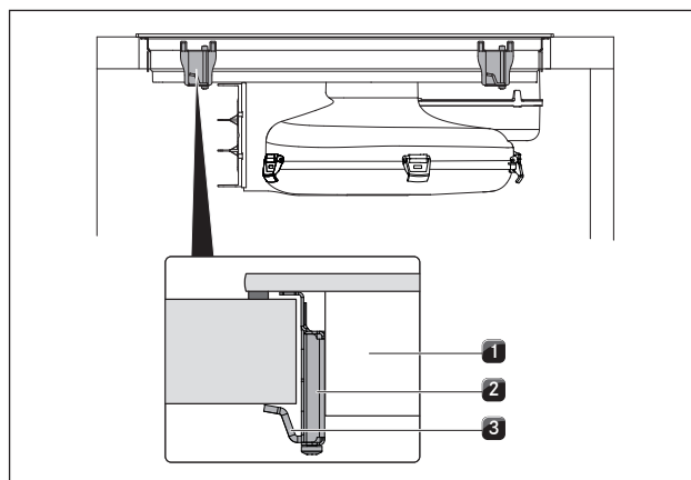
SI. 8.39 Pritrjevanje kuhalne plošče
