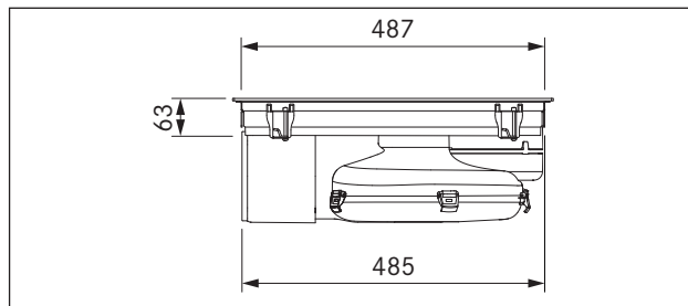
SI. 5.12 Dimenzije naprave PURU, pogled s strani
