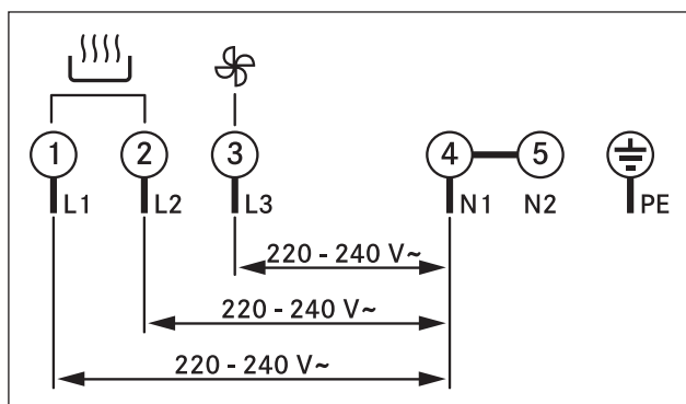
рис. 8.47 Схема подключения к трехфазной сети
