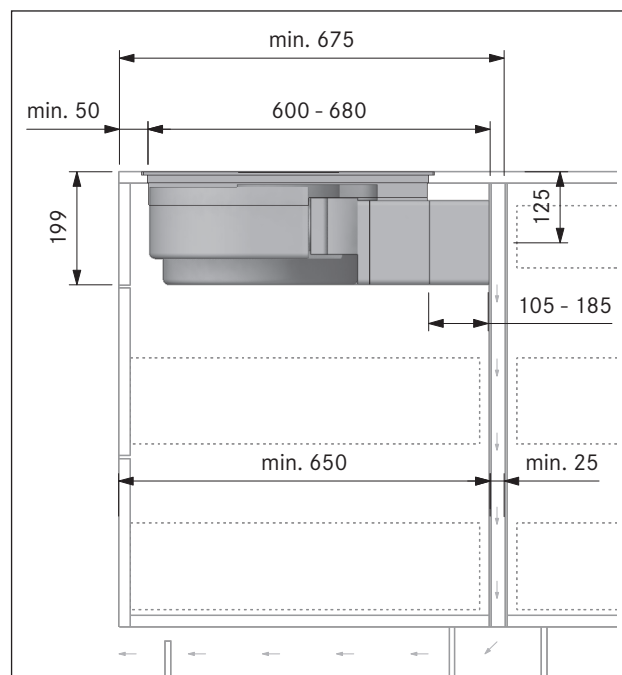
рис. 8.34 Монтажные размеры в варианте с рециркуляцией воздуха, вариант монтажа А, глубина столешницы от 675 мм
