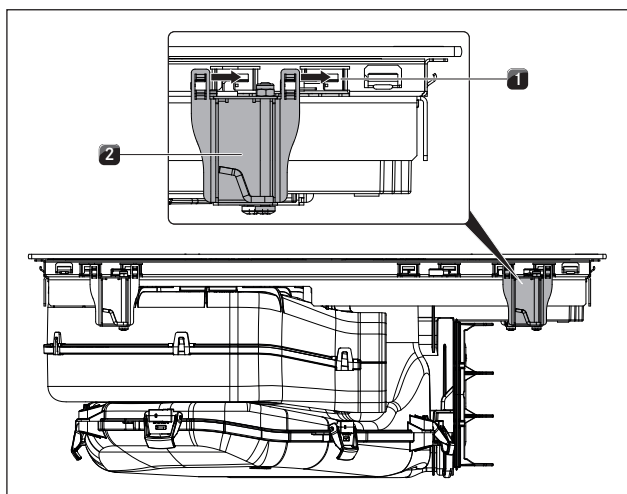
рис. 8.33 Установка монтажных зажимов
