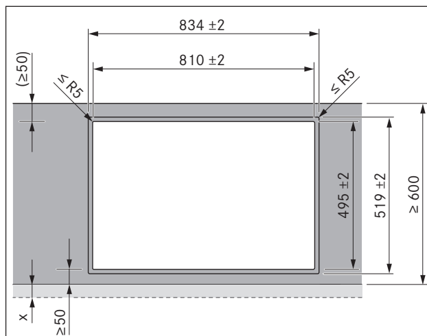
рис. 8.7 Размеры выреза для монтажа заподлицо
