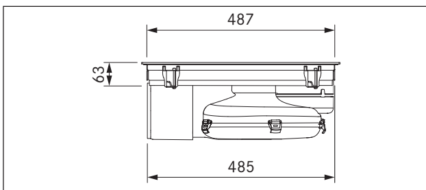
рис. 5.6 Размеры устройства PUXU Вид сбоку
