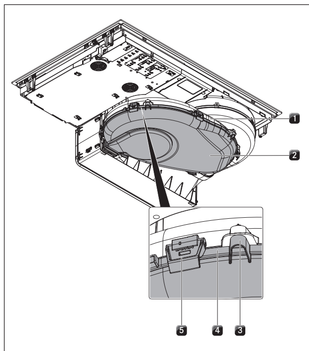
рис. 10.4 Корпус воздушного канала
