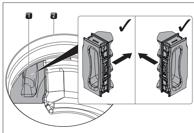
рис. 10.11 Установка откидной крышки фильтра
