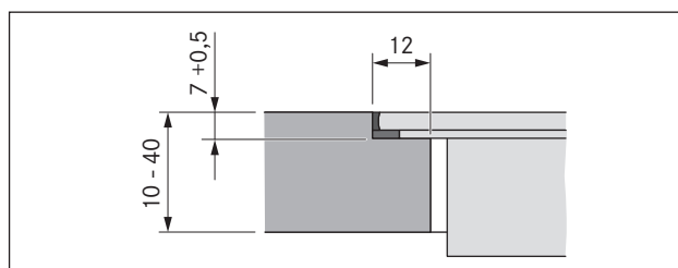
рис. 8.8 Шов для монтажа заподлицо
