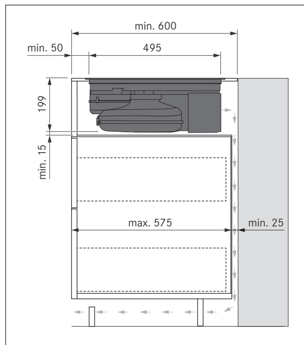
рис. 8.30 Монтажные размеры в варианте с рециркуляцией воздуха, вариант монтажа В, глубина столешницы 600 мм
