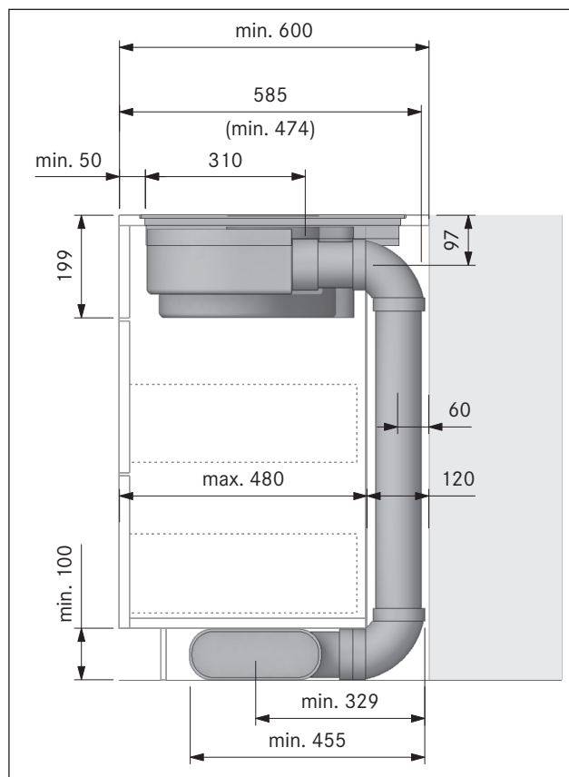
рис. 8.15 Монтажные размеры при установке вытяжной вентиляции, глубина столешницы 600 мм
