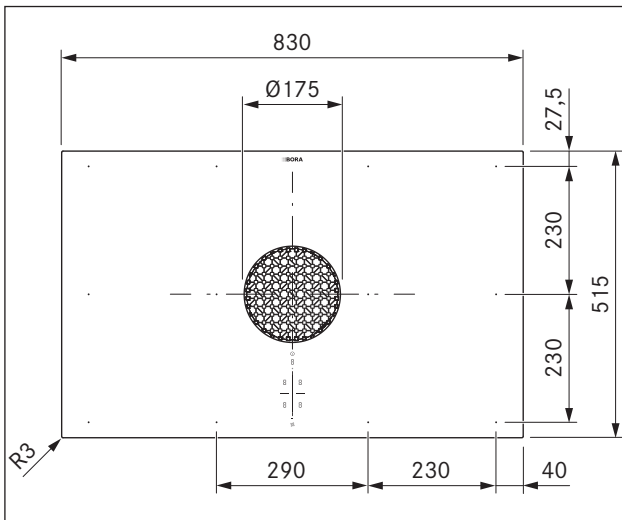
рис. 5.4 Размеры устройства PUXU Вид сверху
