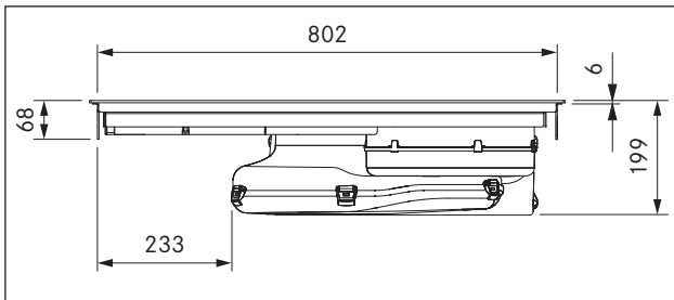
рис. 5.5 Размеры устройства PUXU Вид спереди
