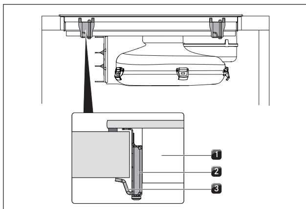
рис. 8.39 Крепление варочной панели
