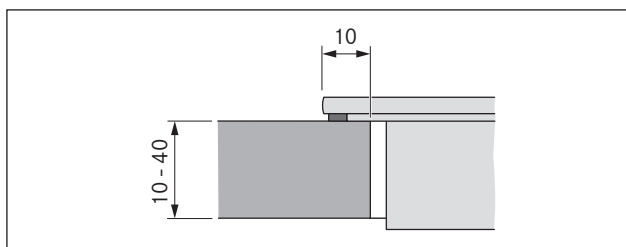
рис. 8.10 Размеры основания для монтажа на поверхности
