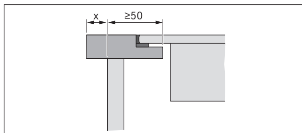
рис. 8.6 Выступ рабочей поверхности
