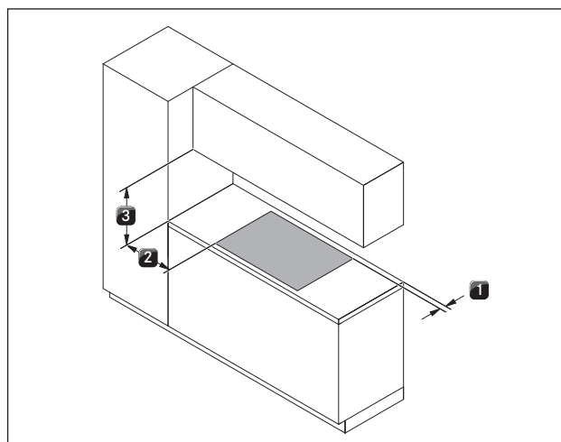
рис. 8.3 обязательные безопасные расстояния
