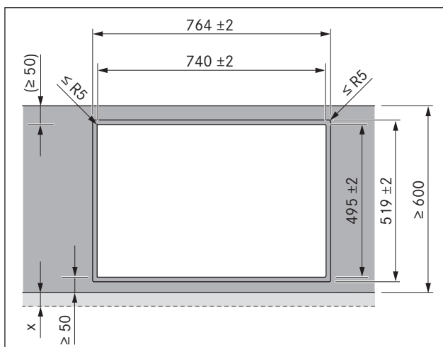
рис. 8.11 Размеры выреза для монтажа заподлицо
