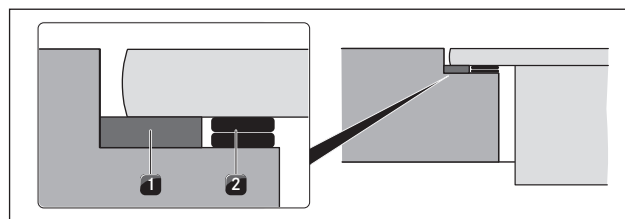
рис. 8.38 Пластины для выравнивания по высоте
