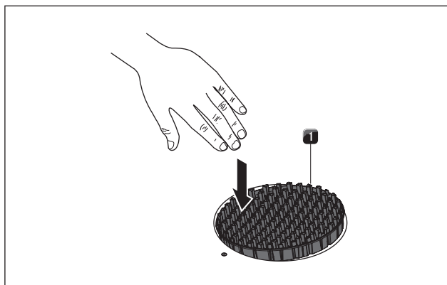
рис. 10.1 Снятие впускного клапана PUXA, PUXU
