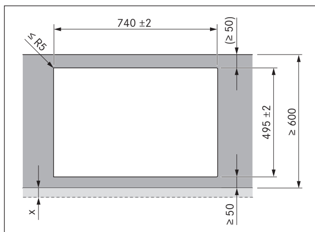
рис. 8.13 Размеры выреза для навесного монтажа
