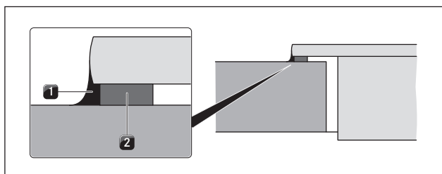
рис. 8.31 Навесной монтаж с использованием уплотнительной ленты
