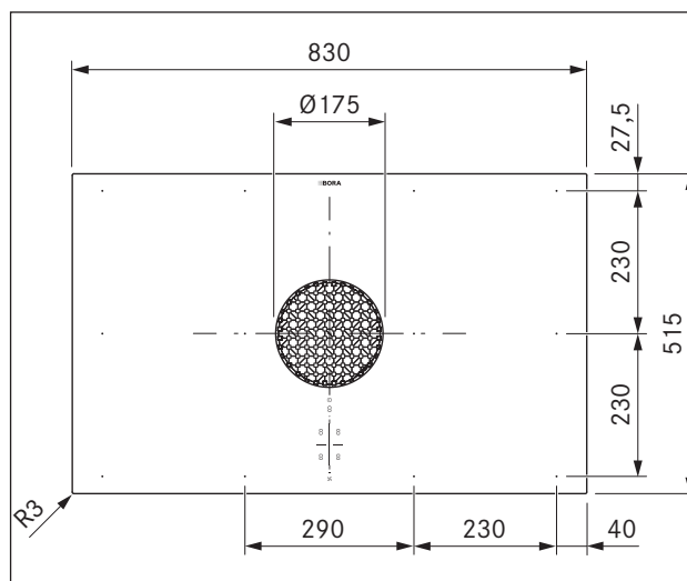
рис. 5.1 Размеры устройства PUXA Вид сверху
