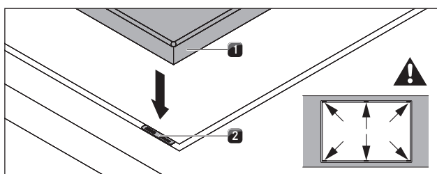
рис. 8.20 Установка пластин для выравнивания по высоте
