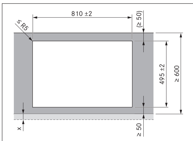
рис. 8.9 Размеры выреза для навесного монтажа
