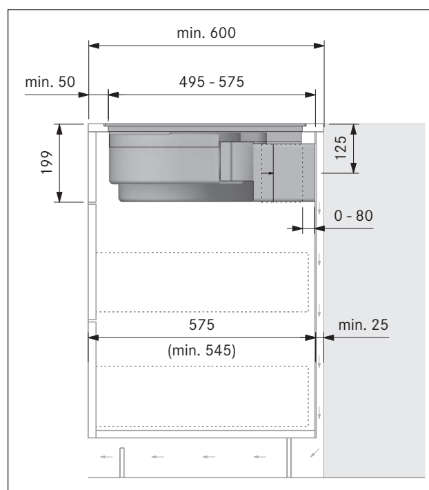
рис. 8.27 Монтажные размеры в варианте с рециркуляцией воздуха, вариант монтажа А
