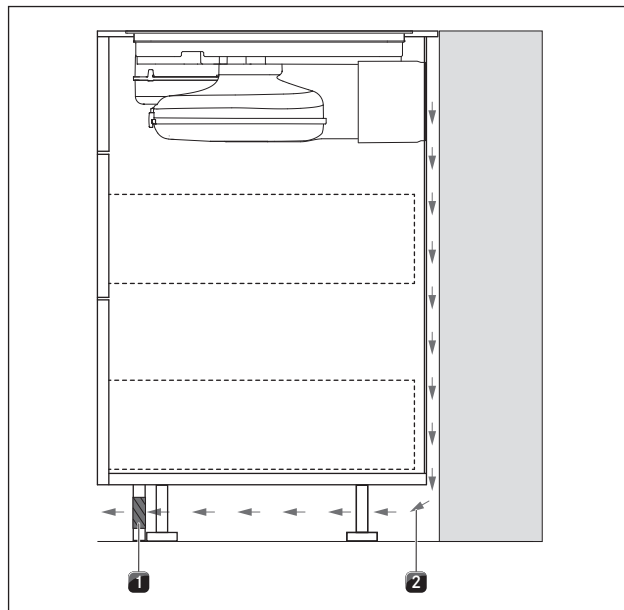
рис. 8.24 Отверстие для обратного потока в цоколе
