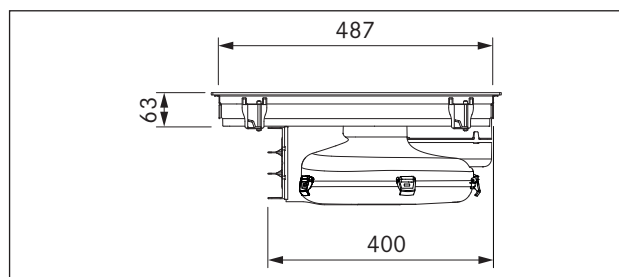
рис. 5.3 Размеры устройства PUXA Вид сбоку
