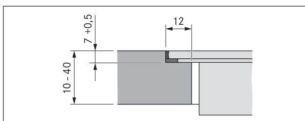
рис. 8.12 Шов для монтажа заподлицо
