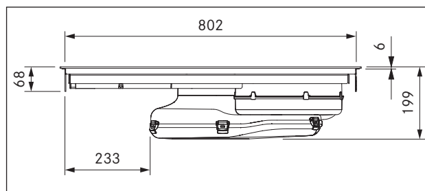
рис. 5.2 Размеры устройства PUXA Вид спереди
