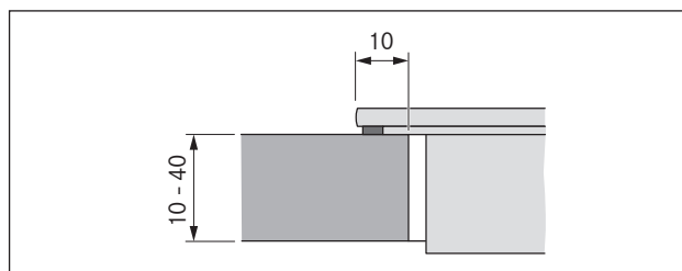
рис. 8.14 Размеры основания для монтажа на поверхности
