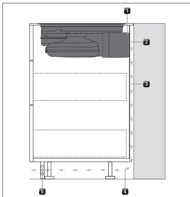
рис. 8.25 Вариант монтажа для сплошной задней стенки
