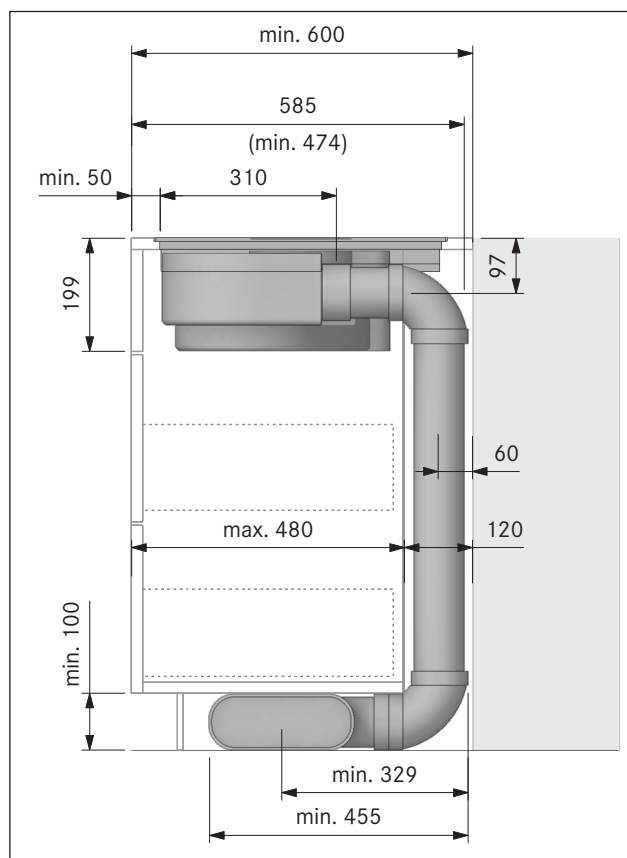
Fig. 6.15 Medidas de montagem para extração de ar, profundidade da bancada de 600 mm
