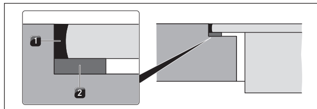
Fig. 6.17 Cinta vedante para montagem à face
