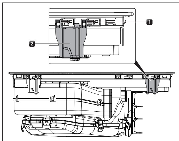
Fig. 6.18 Instalar grampos de montagem
