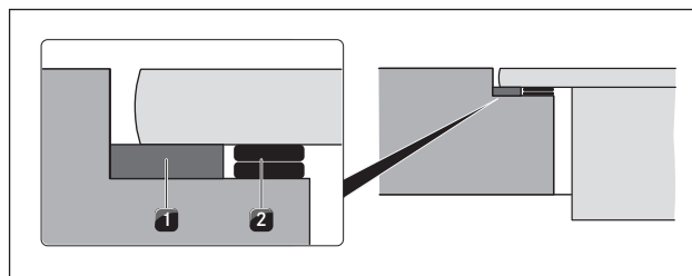
Fig. 6.21 Placas de compensação da altura
