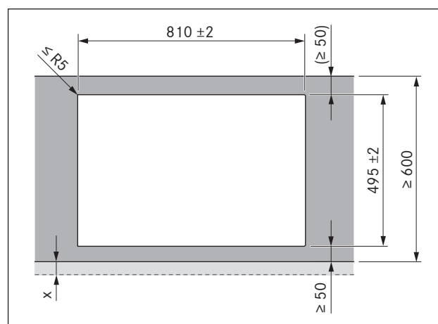
Fig. 6.9 Medidas de recorte para montagem por sobreposição
