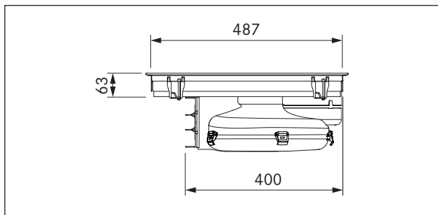
Fig. 3.9 PURA dimensões do aparelho vista lateral
