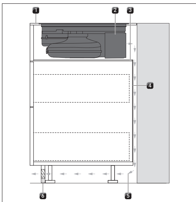
Fig. 6.26 Variante de montagem com fundo falso
