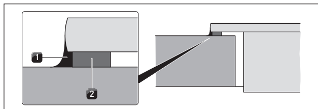
Fig. 6.16 Cinta vedante para montagem por sobreposição
