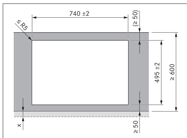
Fig. 6.13 Medidas de recorte para montagem por sobreposição
