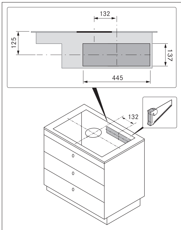
Fig. 6.28 Recorte da abertura de retorno
