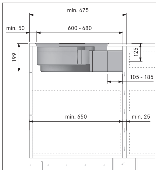
Fig. 6.34 Medidas de montagem para a circulação de ar, variante de montagem A, profundidade da bancada a partir de 675 mm
