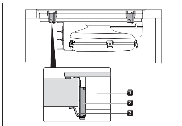
Fig. 6.22 Fixar a placa de cozinhar centrada
