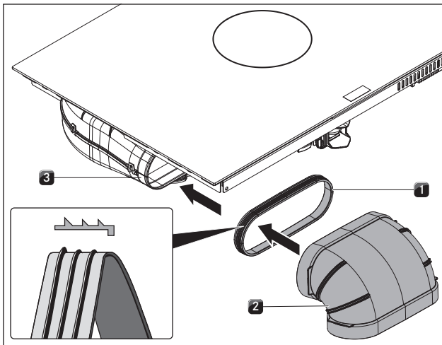
Fig. 6.23 Ligação ao sistema de condutas
