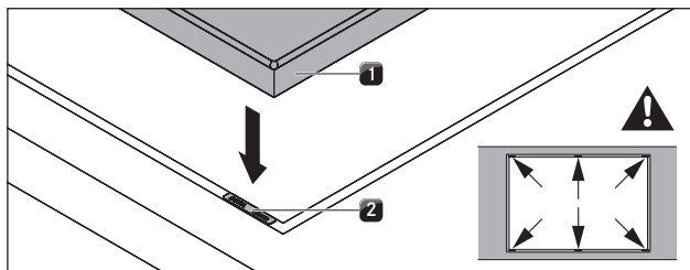
Fig. 6.20 Inserir as placas de compensação de altura
