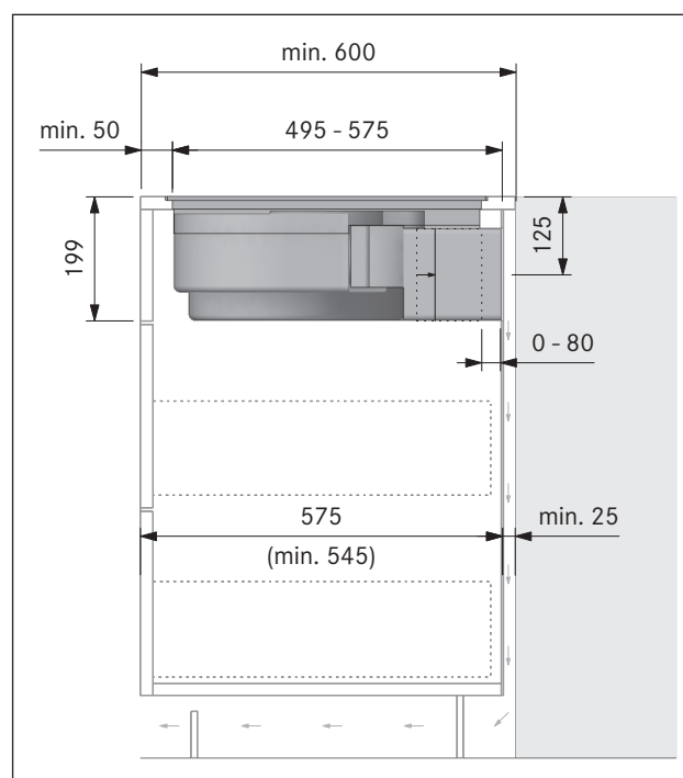
Fig. 6.27 Medidas de montagem para a circulação de ar, variante de montagem A
