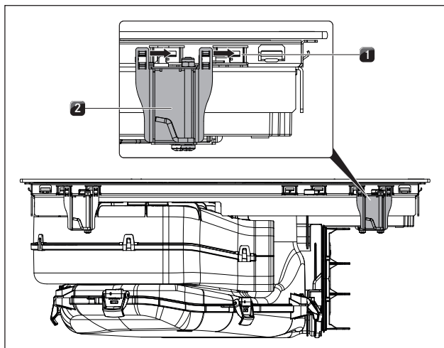
Fig. 6.33 Instalar grampos de montagem
