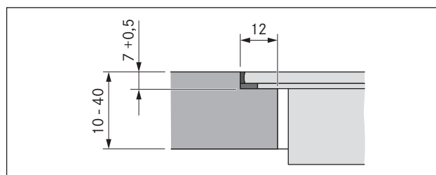
Fig. 6.8 Medida de recesso para montagem à face
