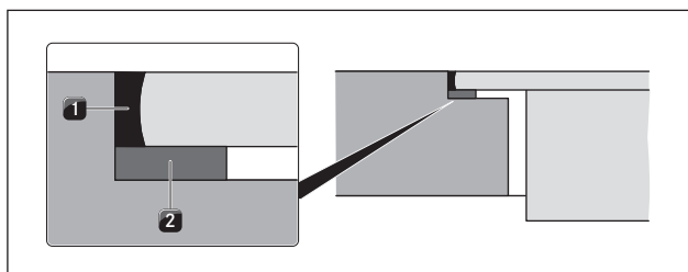
Fig. 6.32 Cinta vedante para montagem à face
