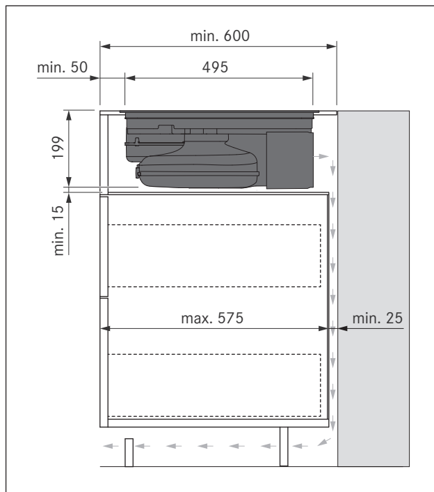
Fig. 6.30 Medidas de montagem para a circulação de ar, variante de montagem B, profundidade da bancada de 600 mm
