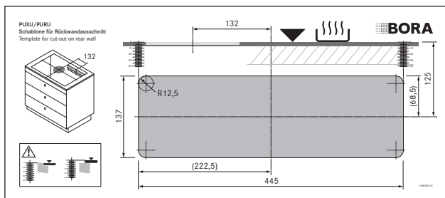
Fig. 6.29 Molde para o recorte do painel traseiro
