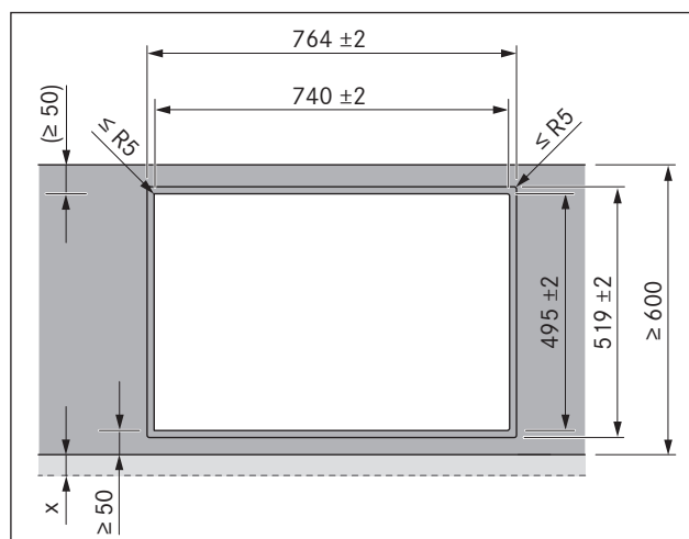
Fig. 6.11 Medidas de recorte para montagem à face
