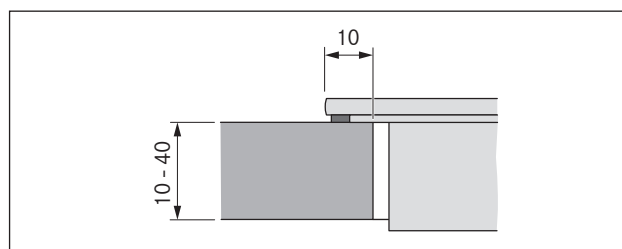
Fig. 6.10 Medida do apoio para montagem por sobreposição
