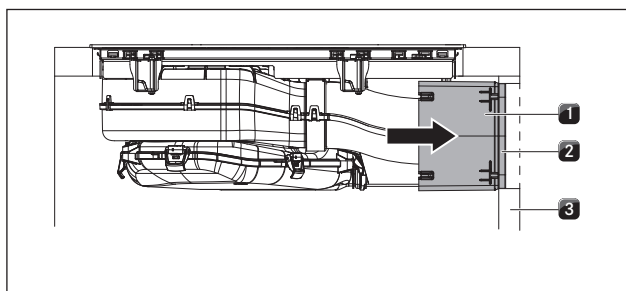
Fig. 6.37 Tilslutning til bagvæggen
