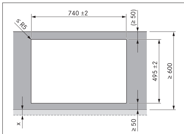
Fig. 6.14 Udskæringsmål til overflademontering
