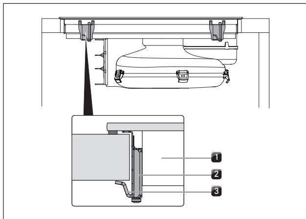
Fig. 6.36 Fastgøring af kogeplade
