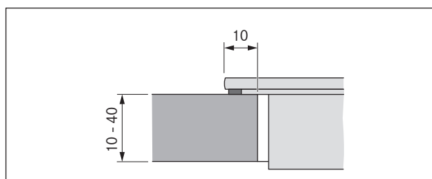
Fig. 6.15 Påsætningsmål til overflademontering
