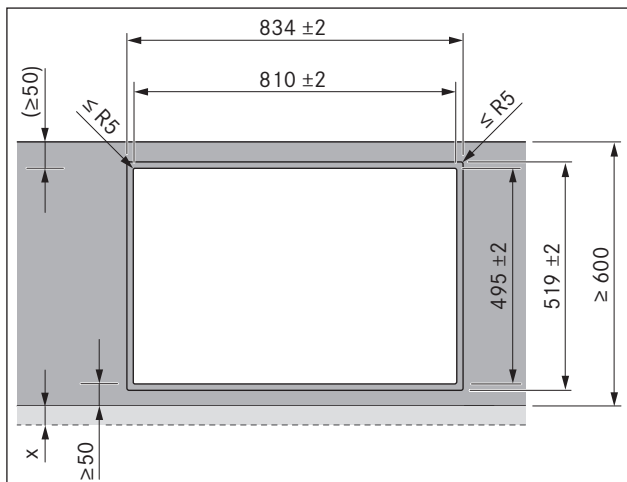
Fig. 6.8 Udskæringsmål til planlimet montering
