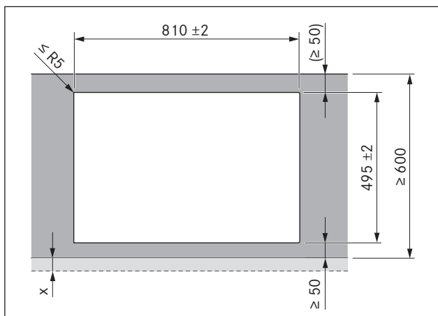
Fig. 6.10 Udskæringsmål til overflademontering
