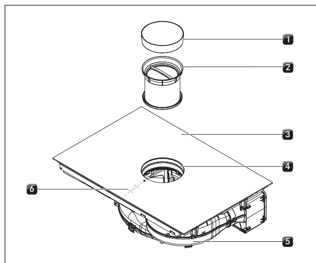
Fig. 5.1 Kogeplade
