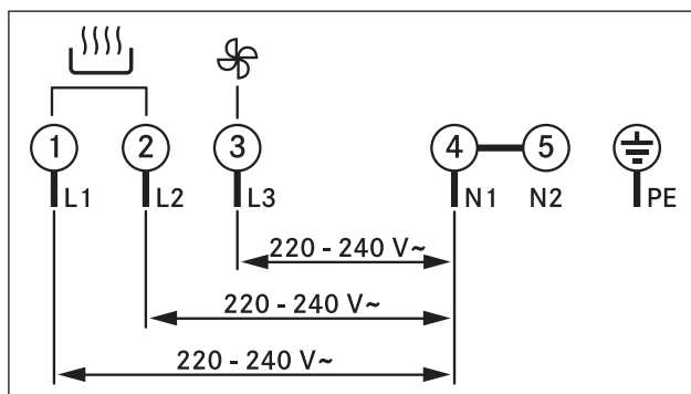
Fig. 6.44 Tilslutningsskema Trefase-tilslutning
