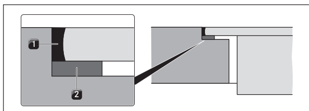
Fig. 6.30 Forseglingsstape ved planlimet montering
