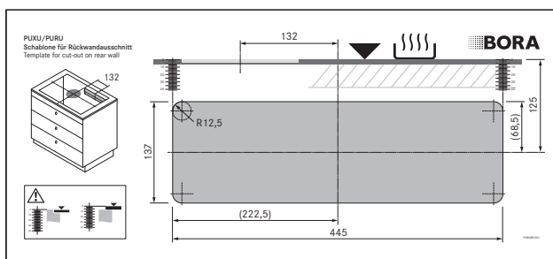
Fig. 6.28 Skabelon til udskæring i bagvæggen
