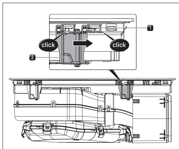
Fig. 6.31 Indsætning af kogepladen
