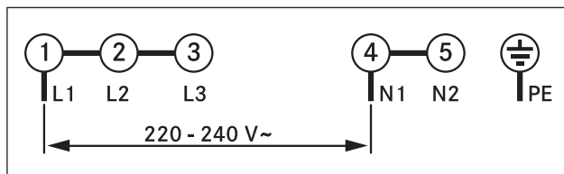
Fig. 6.46 Tilslutningsskema Enfase-tilslutning
