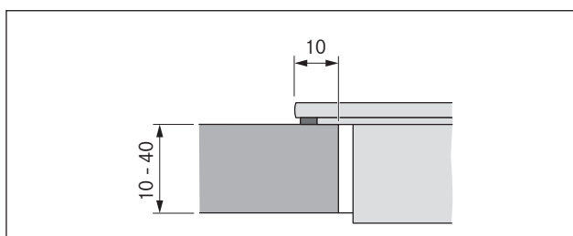
Fig. 6.11 Påsætningsmål til overflademontering
