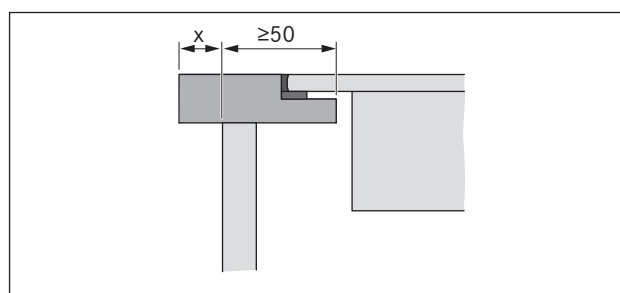
Fig. 6.7 Bordpladefremspring
