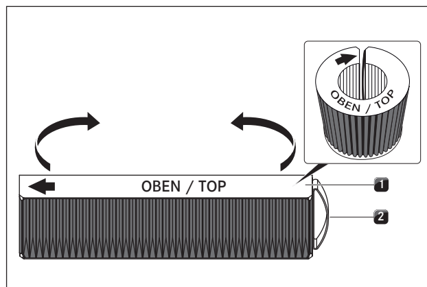
Fig. 6.39 Aktivt-kul-filter
