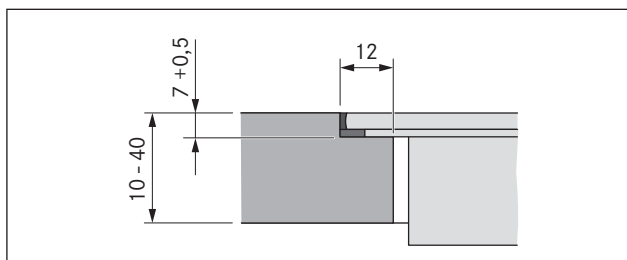
Fig. 6.9 Falsmål til planlimet montering
