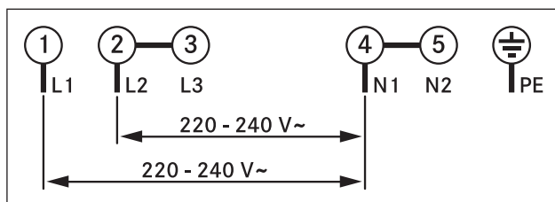
Fig. 6.45 Tilslutningsskema Tofase-tilslutning
