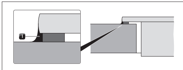
Fig. 6.55 Silicona de sellado para montaje superpuesto
