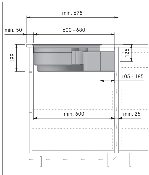
Fig. 6.33 Medidas de montaje para la variante de recirculación A, profundidad de la encimera 675 mm o más
