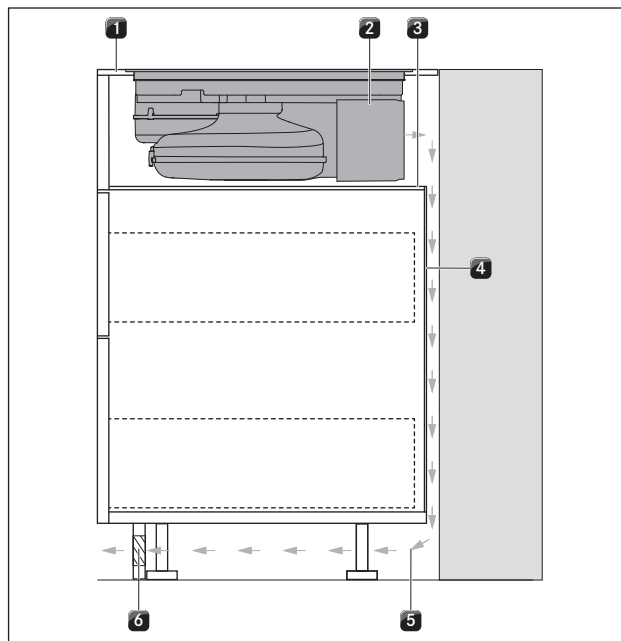
Fig. 6.25 Variante de montaje con base intermedia
