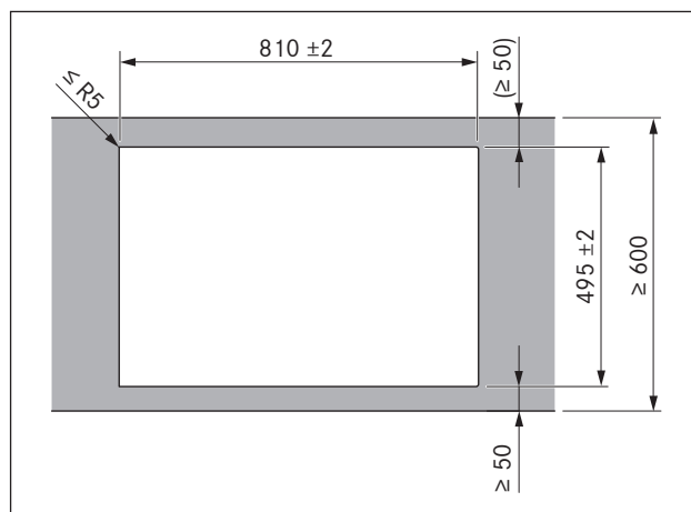
Fig. 6.8 Medidas del recorte para montaje superpuesto
