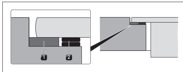
Fig. 6.20 Placas de compensación de altura
