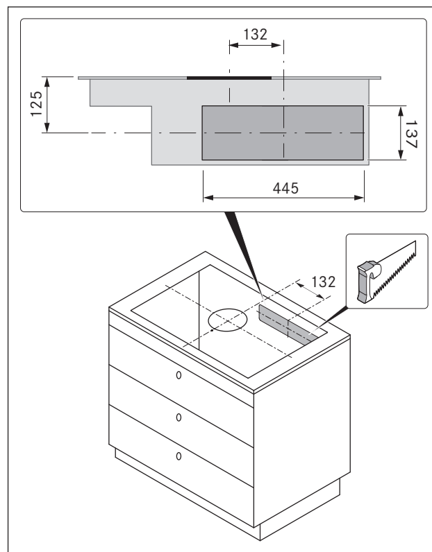
Fig. 6.27 Recorte de la abertura de flujo de retorno
