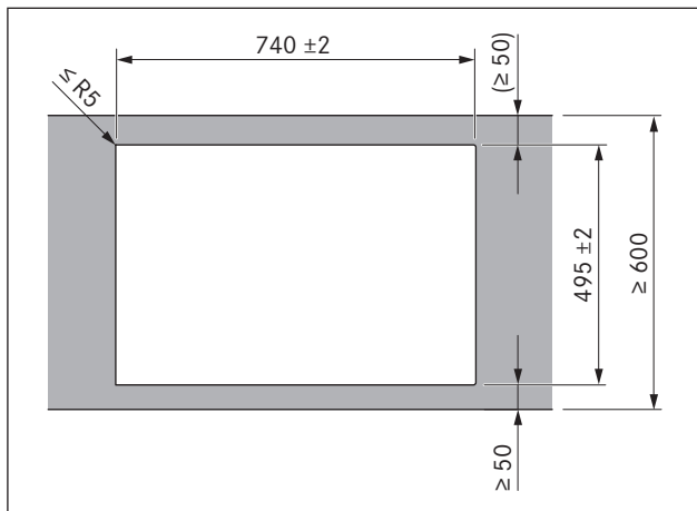
Fig. 6.12 Medidas del recorte para montaje superpuesto
