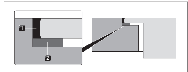
Fig. 6.31 Cinta selladora para montaje enrasado
