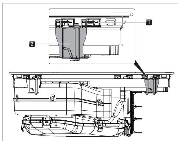
Fig. 6.17 Colocación de las abrazaderas de montaje
