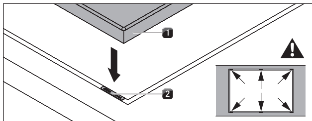
Fig. 6.19 Colocación de placas de compensación de altura
