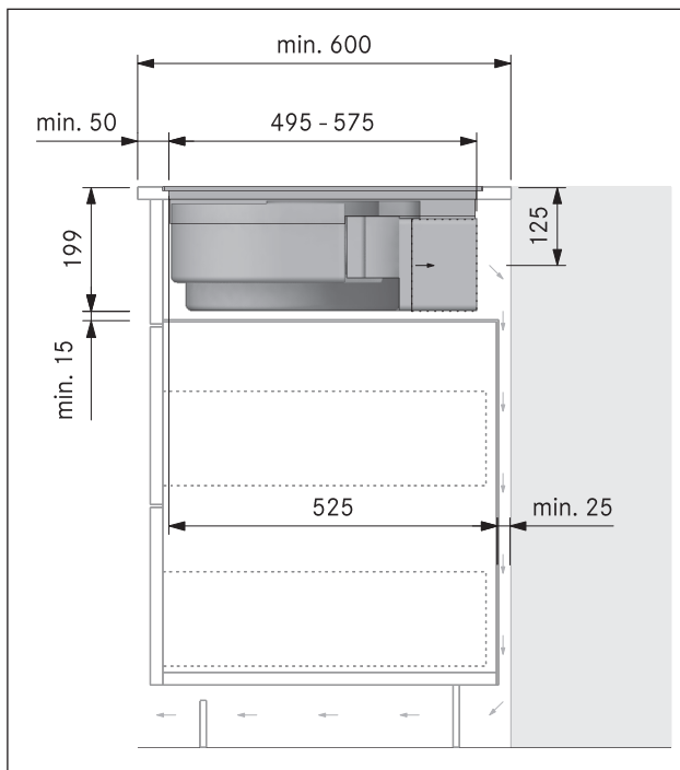
Fig. 6.29 Medidas de montaje para la variante de recirculación B, profundidad de la encimera 600 mm
