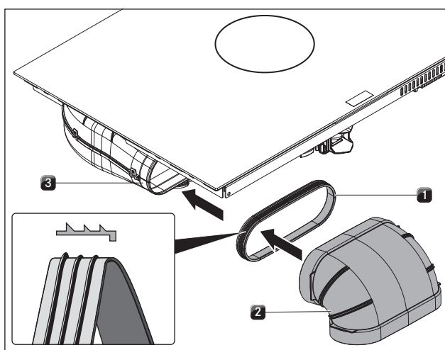
Fig. 6.22 Conexión al sistema de conductos
