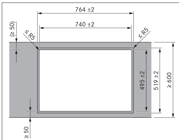
Fig. 6.10 Medidas del recorte para montaje enrasado
