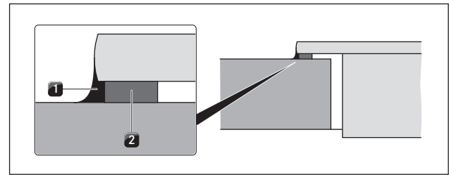
Fig. 6.30 Cinta selladora para superposición
