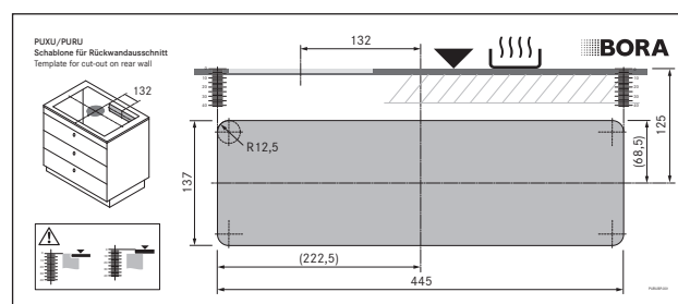
Fig. 6.28 Plantilla para el recorte del panel trasero
