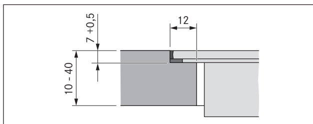
Fig. 6.11 Medida del pliegue para un montaje enrasado
