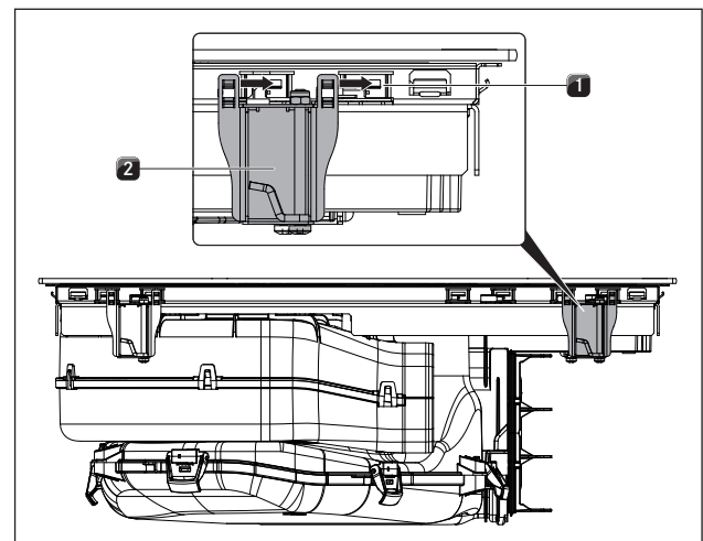
Fig. 6.32 Colocación de las abrazaderas de montaje
