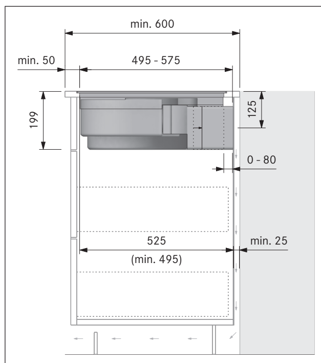
Fig. 6.26 Medidas de montaje con recirculación, variante de montaje A
