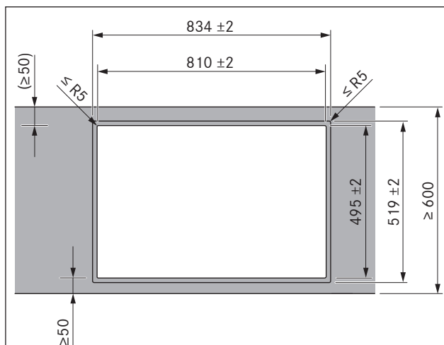
Fig. 6.6 Medidas del recorte para montaje enrasado
