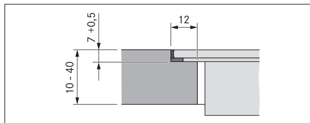
Fig. 6.7 Medida del pliegue para un montaje enrasado
