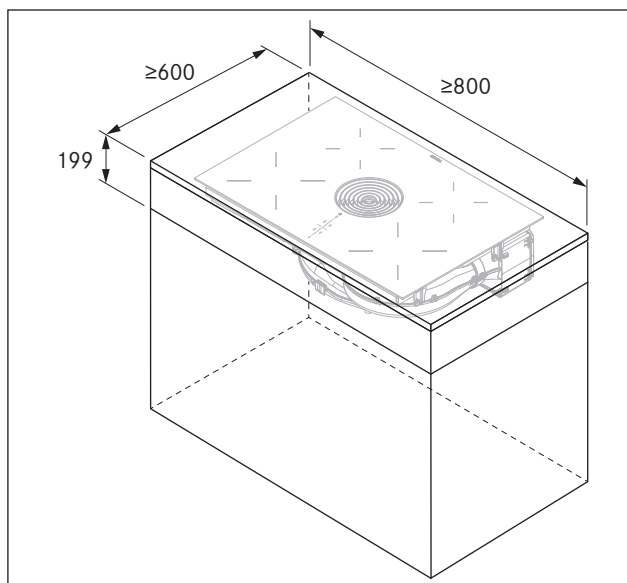
Fig. 6.5 Medidas mínimas de los muebles Pure
