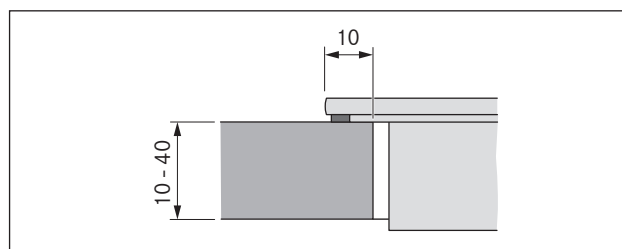
Fig. 6.9 Dimensiones para montaje superpuesto
