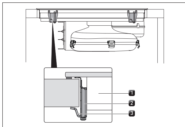
Fig. 6.21 Fijación de la placa de cocción en posición centrada
