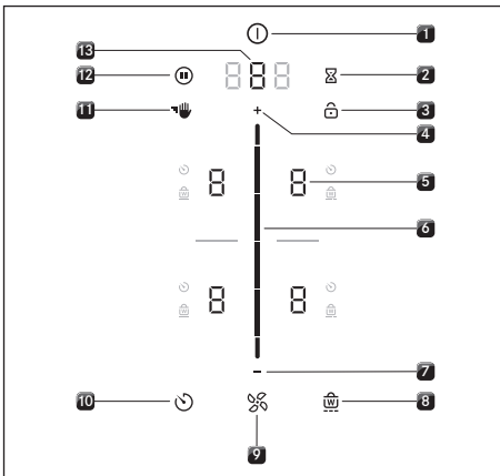
Fig. 5.5 Touch zones/buttons
