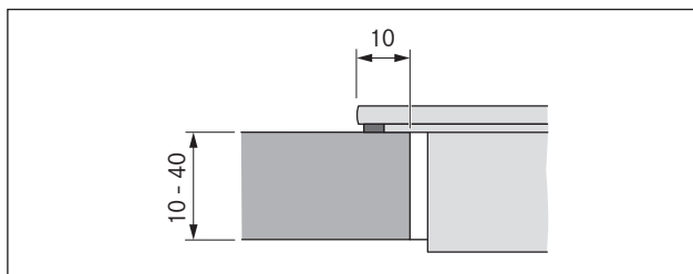
Ilustracja 8.10 Wymiary podparcia dla montażu elementu z uskokiem
