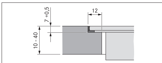
Ilustracja 8.12 Wielkość zakładki przy montażu z zachowaniem równej powierzchni
