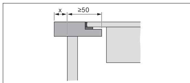
Ilustracja 8.6 Wystający na zewnątrz odcinek blatu
