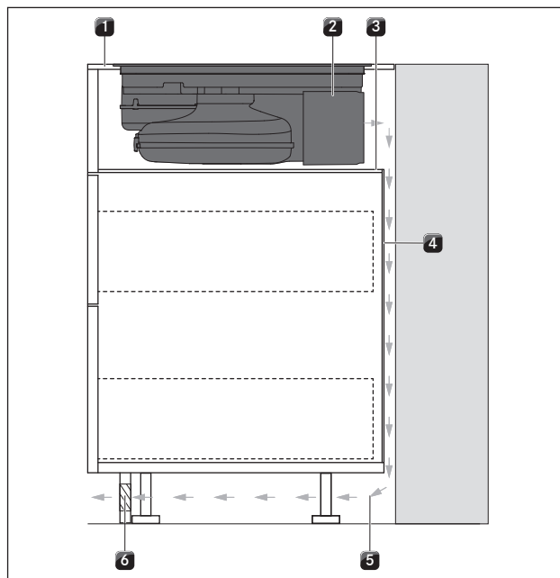
Ilustracja 8.26 Warianty montażowe z płytą pośrednią
