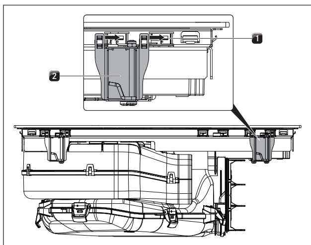
Ilustracja 8.18 Zakładanie zacisków montażowych
