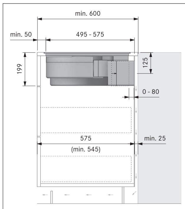
Ilustracja 8.27 Wymiary zabudowy przy pracy w obiegu zamkniętym, wariant montażowy A
