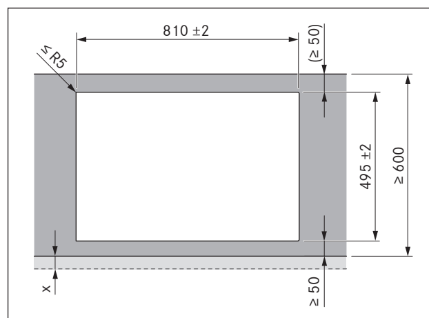
Ilustracja 8.9 Wymiary wycięcia dla montażu elementu z uskokiem
