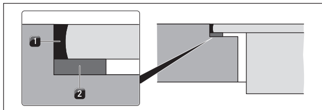
Ilustracja 8.17 Taśma uszczelniająca przy montażu z zachowaniem równej powierzchni
