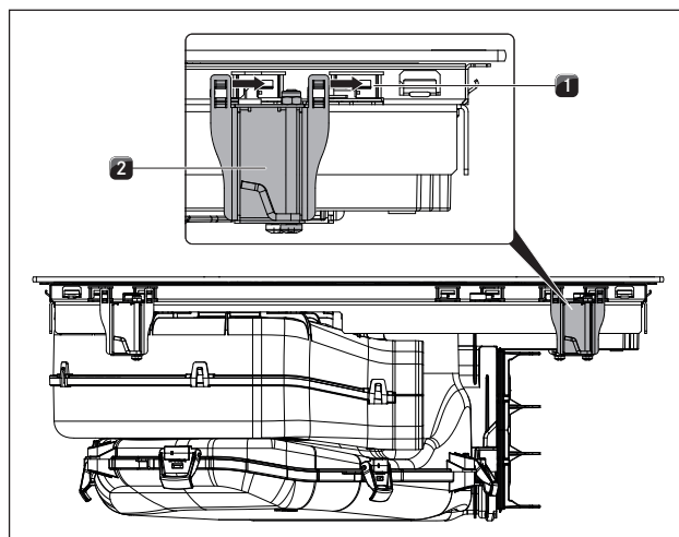
Ilustracja 8.33 Zakładanie zacisków montażowych
