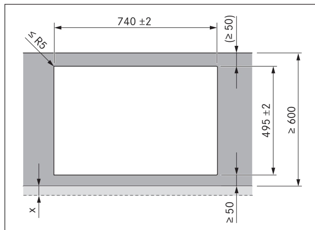
Ilustracja 8.13 Wymiary wycięcia dla montażu elementu z uskokiem
