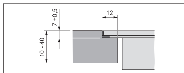
Ilustracja 8.8 Wielkość zakładki przy montażu z zachowaniem równej powierzchni
