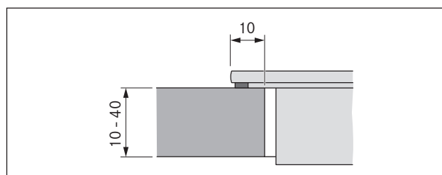
Ilustracja 8.14 Wymiary podparcia dla montażu elementu z uskokiem
