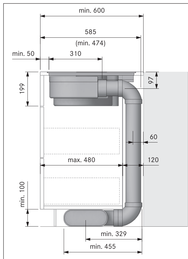
Ilustracja 8.15 Wymiary zabudowy w przypadku trybu pracy z odprowadzaniem powietrza na zewnątrz, głębokość blatu 600 mm
