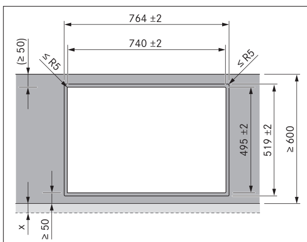
Ilustracja 8.11 Wymiary wycięcia dla montażu z zachowaniem równej powierzchni
