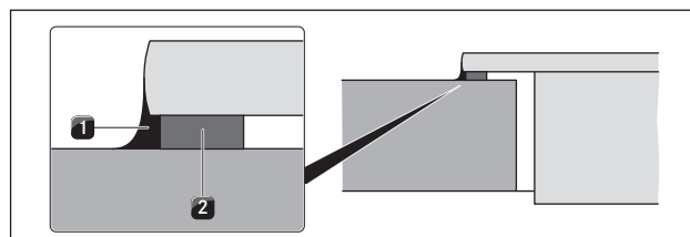
Ilustracja 8.16 Taśma uszczelniająca przy montażu elementu z uskokiem
