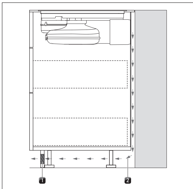
Ilustracja 8.24 Otwór na strumień zwrotny w obszarze cokołu
