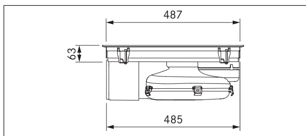
Ilustracja 5.6 PUXU Wymiary urządzenia - widok z boku
