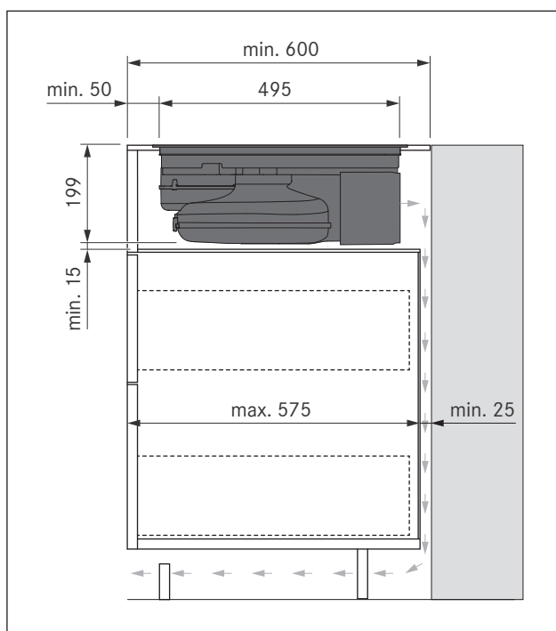
Ilustracja 8.30 Wymiary zabudowy przy pracy w obiegu zamkniętym – wariant montażowy B, głębokość blatu 600 mm
