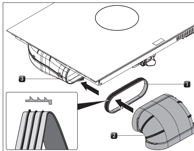
Ilustracja 8.23 Podłączenie do systemu kanałów
