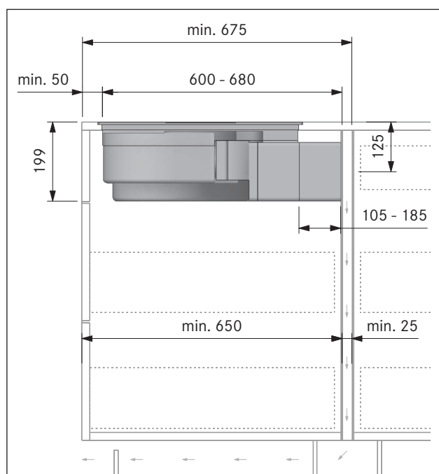
Ilustracja 8.34 Wymiary zabudowy przy pracy w obiegu zamkniętym - wariant montażowy A, głębokość blatu od 675 mm
