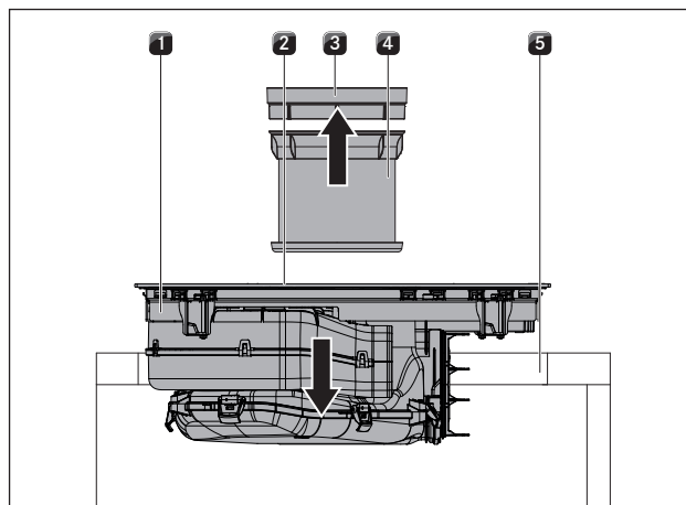
Ilustracja 8.19 Wkładanie płyty grzewczej
