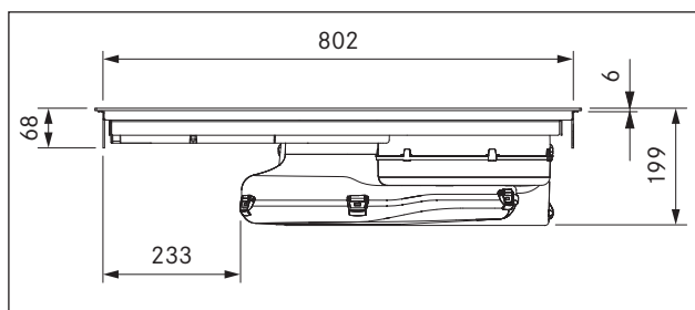
Ilustracja 5.5 PUXU Wymiary urządzenia - widok z przodu
