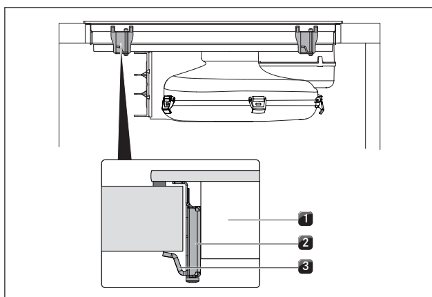
Ilustracja 8.22 Centralne mocowanie płyty grzewczej
