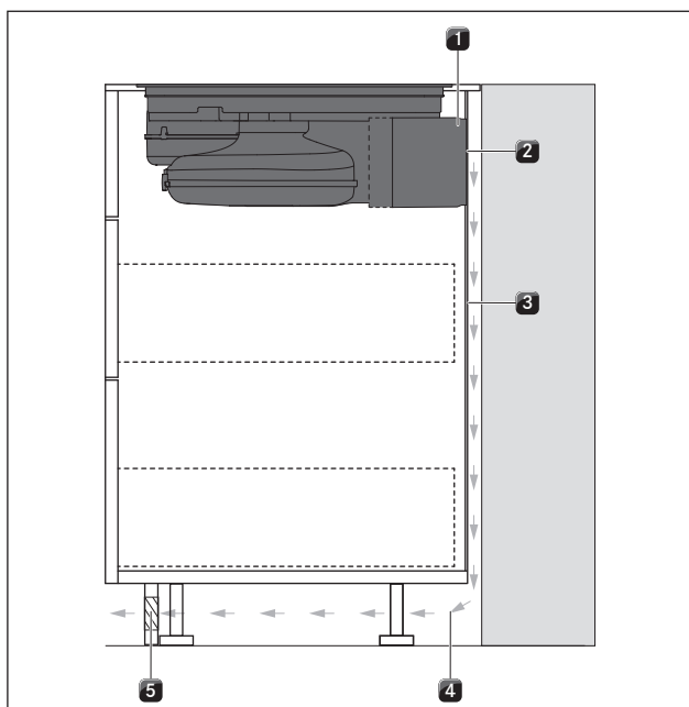
Ilustracja 8.25 Wariant montażowy z ciągłą ścianą tylną
