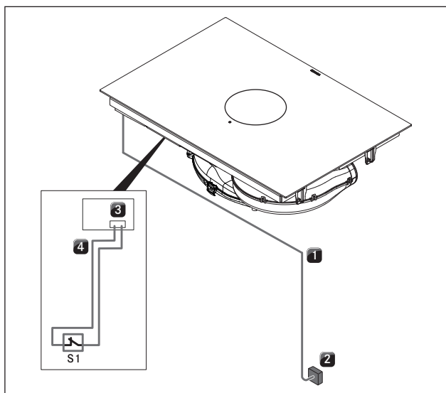
Ilustracja 8.46 Schemat podłączenia z opcjonalnym modułem Home In
