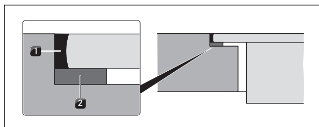
Ilustracja 8.32 Taśma uszczelniająca przy montażu z zachowaniem równej powierzchni
