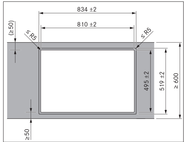
איור 6.6 מידות פתח עבור התקנה שטוחה
