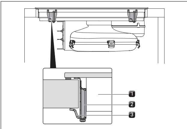
איור 6.38 קיבוע הכיריים
