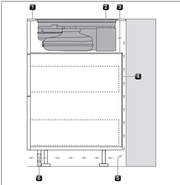
איור 6.25 גרסת התקנה עם משטח הפרדה
