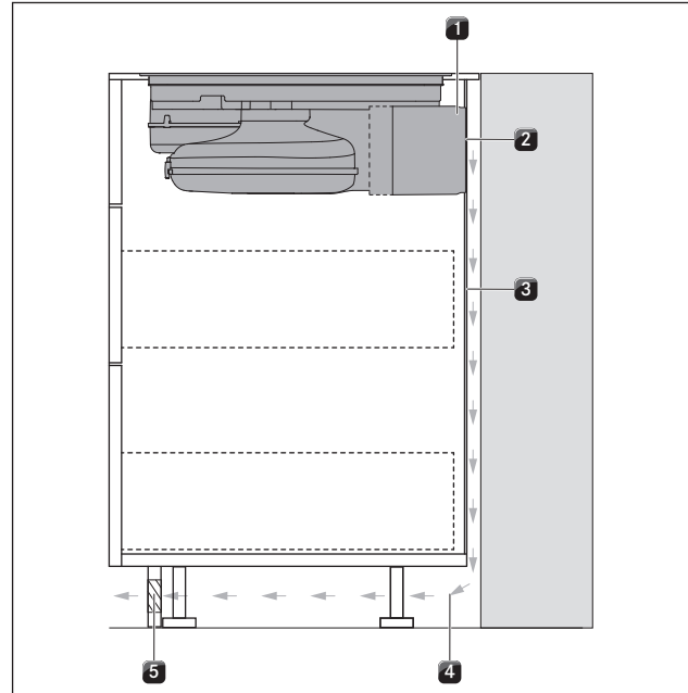
איור 6.24 גרסת התקנה עם דופן מלאה
