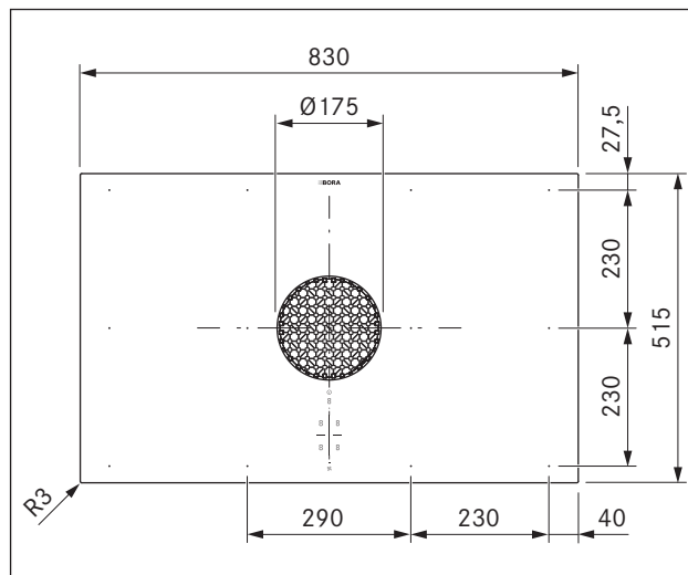
איור 3.4 מידות מכשיר PUXU, מבט מלמעלה
