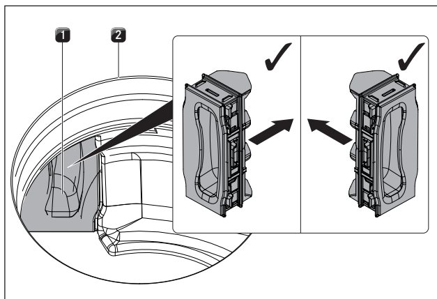
איור 8.11 חיבור מכסה החלפת המסנן
