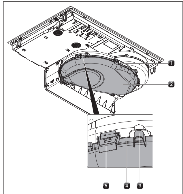
איור 8.4 יחידת ניתוב אוויר
