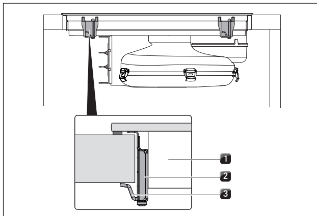
איור 6.21 קיבוע הכיריים במרכז
