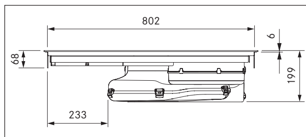
איור 3.5 מידות מכשיר PUXU, מבט מלפנים
