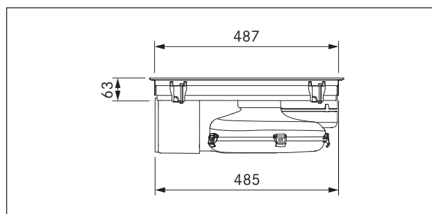
איור 3.6 מידות מכשיר PUXU, מבט מהצד
