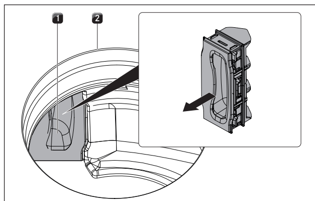
איור 6.40 הסרת מכסה החלפת המסנן
