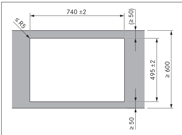
איור 6.12 מידות פתח עבור התקנה עילית
