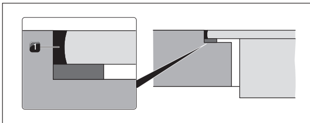
איור 6.55 חומר איטום מסיליקון בהתקנה שטוחה
