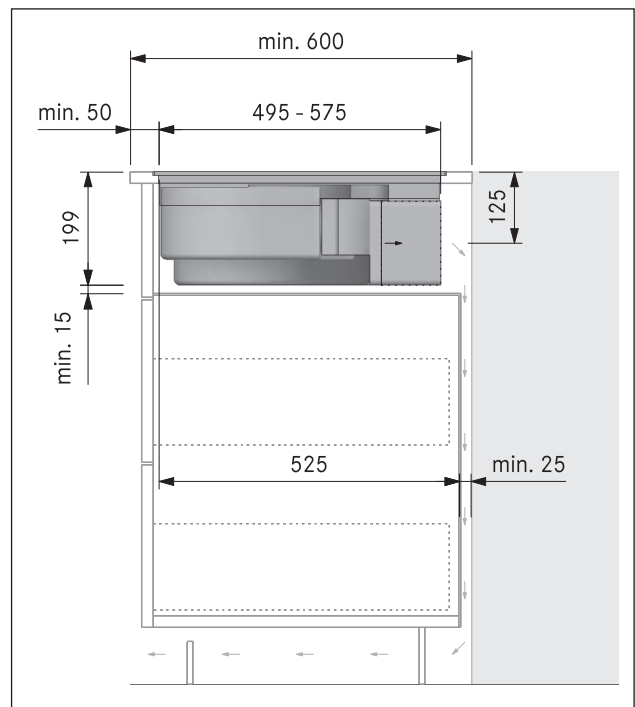
איור 6.29 מידות התקנה בגרסת סחרור אוויר B, עומק משטח עבודה 600 מ"מ
