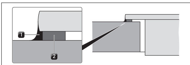
איור 6.15 סרט איטום עבור התקנה עילית
