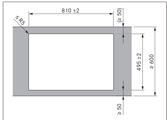
איור 6.8 מידות פתח עבור התקנה עילית
