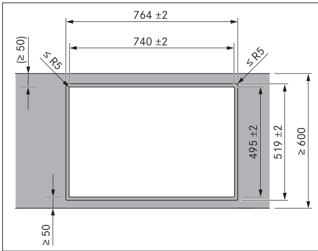
איור 6.10 מידות פתח עבור התקנה שטוחה
