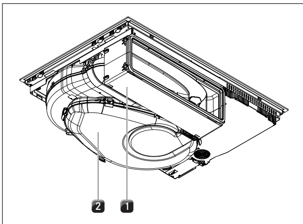
איור 5.3 מבט אחורי PUXU, PURU
