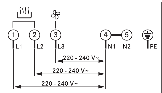
איור 6.46 תרשים חיבורים לחיבור תלת-פאזי
