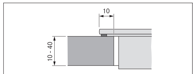
איור 6.9 מידות אוגן עבור התקנה עילית
