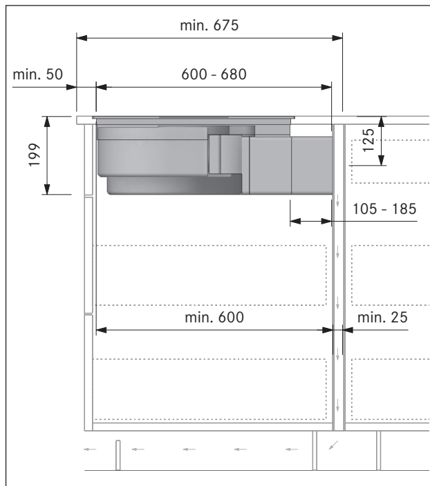
איור 6.33 מידות התקנה בסחרור אוויר, גרסת התקנה A, עומק משטח עבודה החל מ-675 מ"מ
