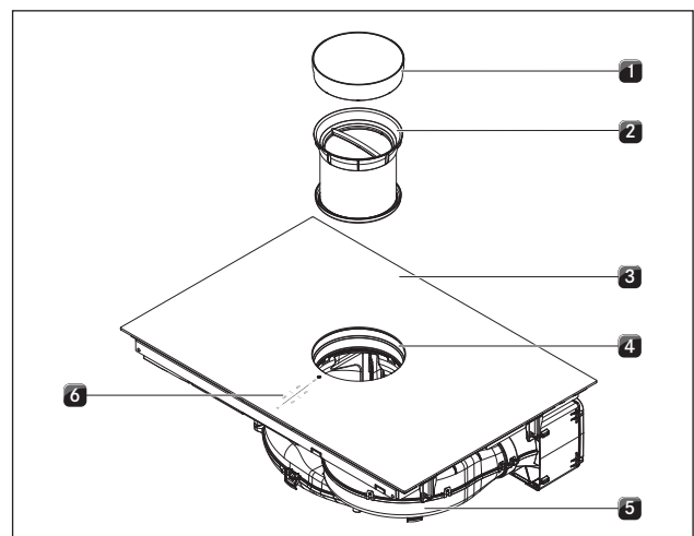
איור 5.1 כיריים
