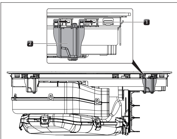
איור 6.32 התקנת ההדקים
