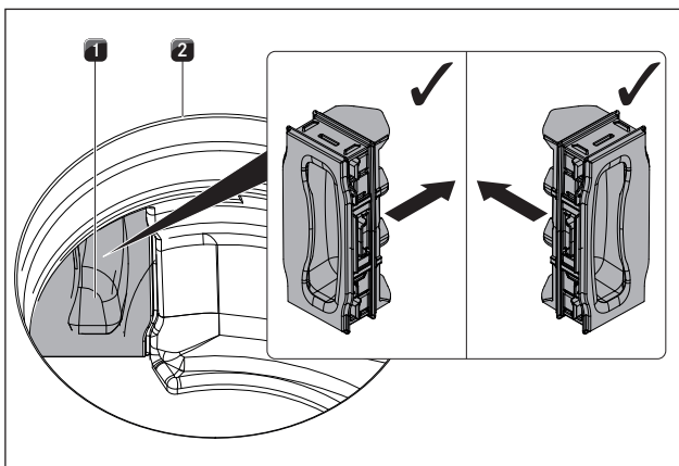
איור 6.44 חיבור מכסה החלפת המסנן
