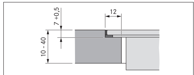
איור 6.7 מידות מדרגה עבור התקנה שטוחה
