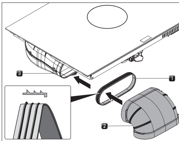
איור 6.22 חיבור למערכת התעלות
