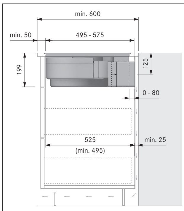
איור 6.26 מידות התקנה בסחרור אוויר, גרסת התקנה A
