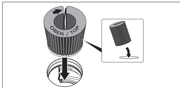
איור 6.42 הכנסת מסנן הפחם הפעיל לפתח השאיבה
