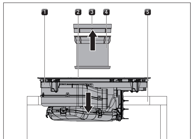
איור 6.18 התקנת הכיריים
