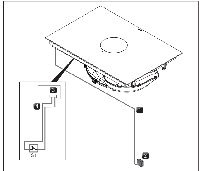
איור 6.45 תרשים חיבורים עם מודול Home-In אופציונלי
