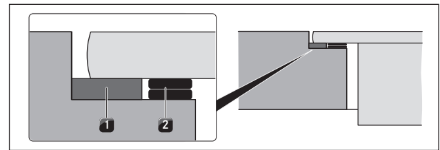
איור 6.37 לוחות איזון גובה
