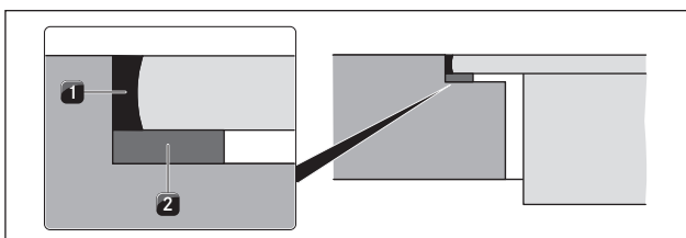
איור 6.16 סרט איטום עבור התקנה שטוחה
