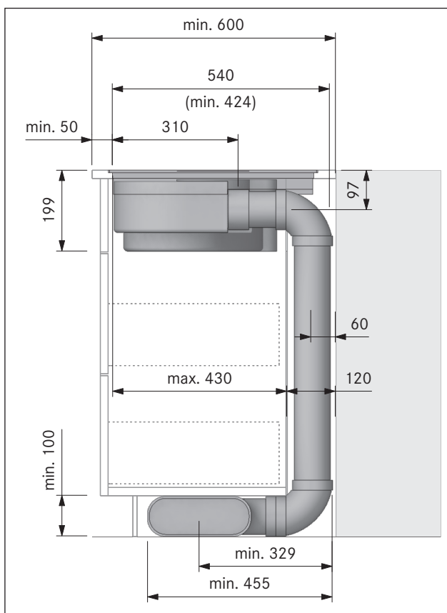
איור 6.14 מידות התקנה עבור יציאת אוויר, עומק משטח עבודה 600 מ"מ
