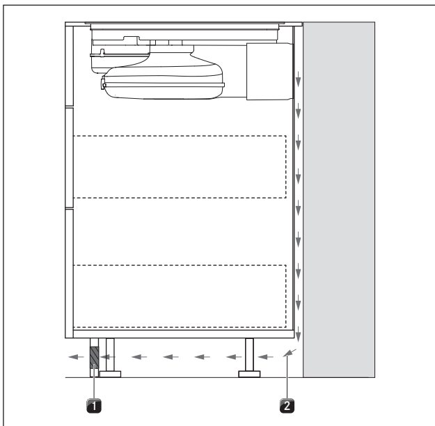
איור 6.23 פתח זרימה חוזרת בבסיס הארון
