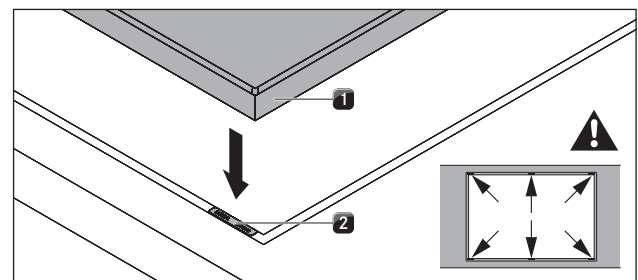
איור 6.36 לוחות איזון גובה
