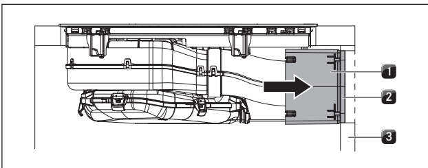
איור 6.39 חיבור לדופן האחורית
