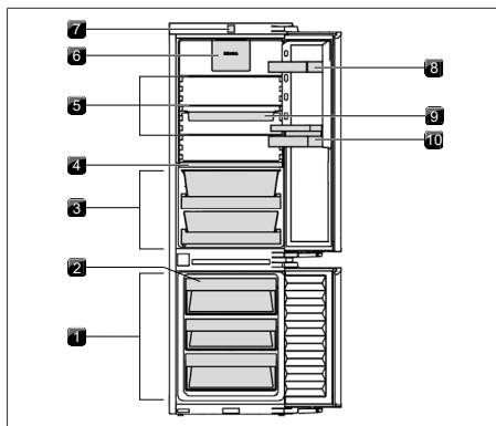
Fig. 5.4 Design C178KGW
