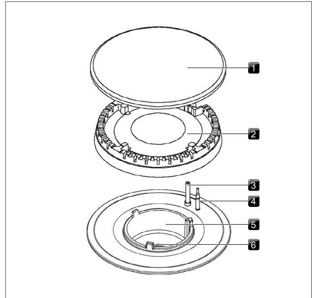
Fig. 7.7 Struttura bruciatore a gas
