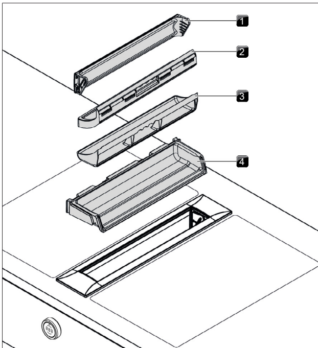
Fig. 3.7 Componenti filtro
