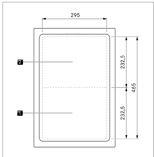
Fig. 3.14 Montaggio griglia Teppanyaki in acciaio inox PKT3 e dimensioni delle zone cottura
