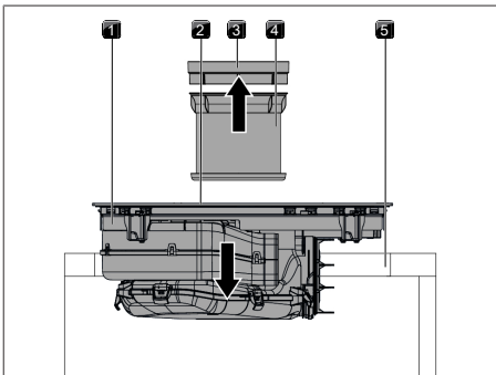
Bild 9.13 Placera spishällen centrerat
