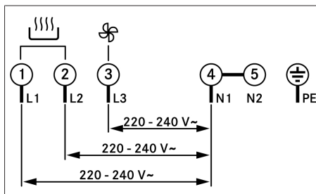
Bild 9.34 Anslutningsschema 3-fas anslutning
