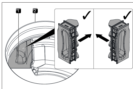
Bild 7.10 Sätta in filterbytesklaffen
