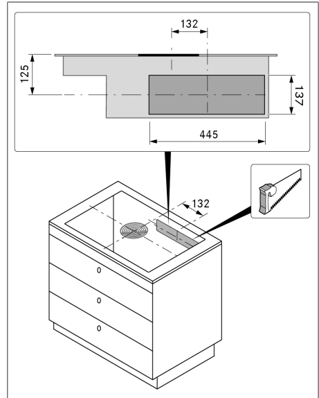
Bild 9.19 Utskärning i den bakre väggen
