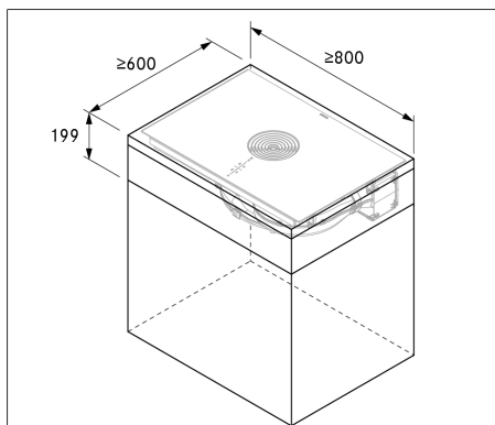
Bild 9.4 Möbels minimimått M Pure
