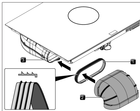
Bild 9.17 Anslutning till kanalsystemet
