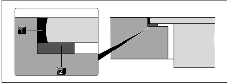
Bild 9.24 Tätningband vid planmontering
