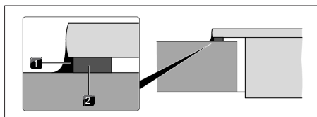
Bild 9.10 Tätningsband vid ytmontering
