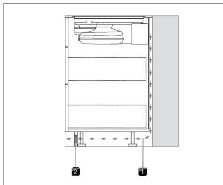
Bild 9.18 Återströmningsöppning i sockelområdet
