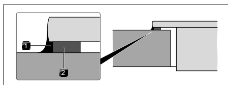
Bild 9.23 Tätningsband vid ytmontering
