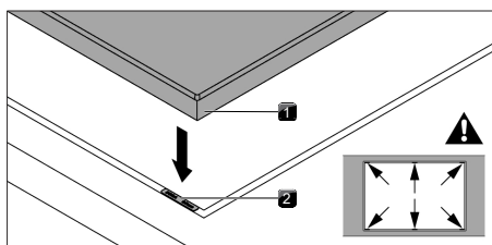
Bild 9.29 Höjdtjämningsplattornas positionering
