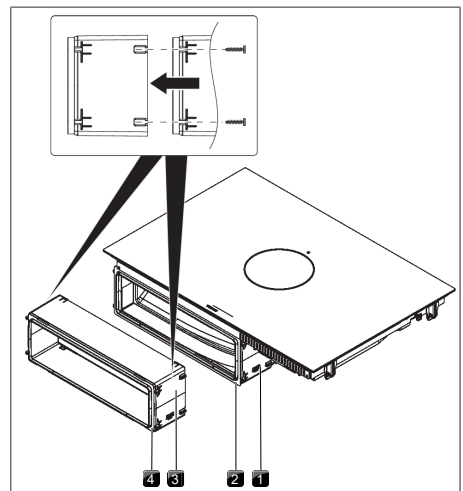
Bild 9.27 Förlängning av teleskoputdraget
