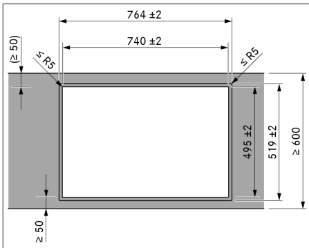
Bild 9.5 Utskärningsmått för planmontering
