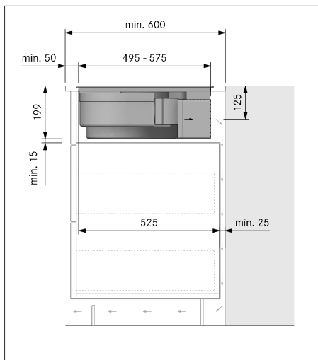
Bild 9.22 Inbyggnadsmått vid luftcirkulation monteringsvariant B, bänkskivans djup 600 mm
