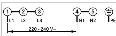
Bild 9.35 Anslutningsschema 1-fas anslutning
