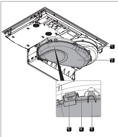
Bild 7.3 Luftledningskåpa
