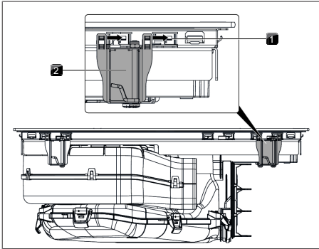
Bild 9.12 Sätta på monteringsklämmorna
