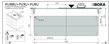
Bild 9.20 Schablon för öppningen i den bakre väggen
