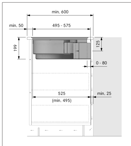
Bild 9.21 Inbyggnadsmått vid luftcirkulation, monteringsvariant A
