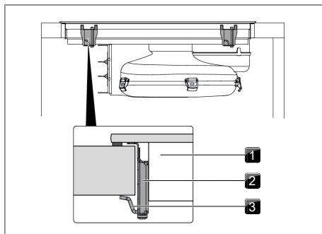
Bild 9.16 Fästa spishällen centrerat
