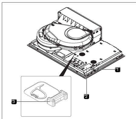
Bild 9.37 Spishällens elektriska anslutningar
