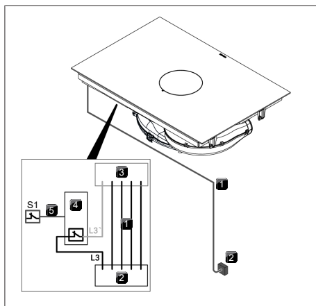
Bild 9.33 Anslutningsschema med extern kontakt
