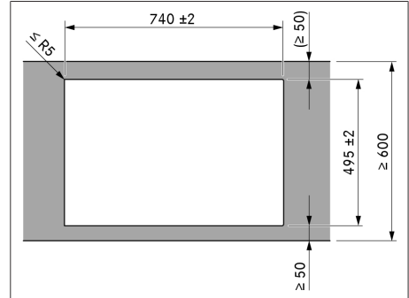
Bild 9.7 Utskärningsmått för ytmonteringen
