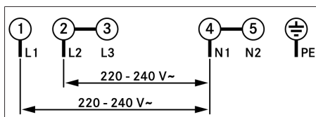
Bild 9.36 Anslutningsschema 2-fas anslutning
