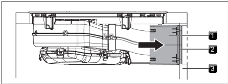
Bild 9.32 Anslutning på bakväggen
