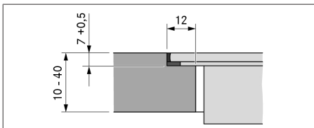
Bild 9.6 Falsmått för planmontering
