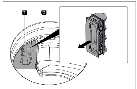
Bild 7.4 Avlägsna filterbytesklaffen
