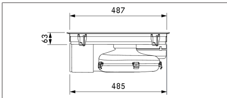
Bild 3.6 PURMU apparatmått bild från sidan
