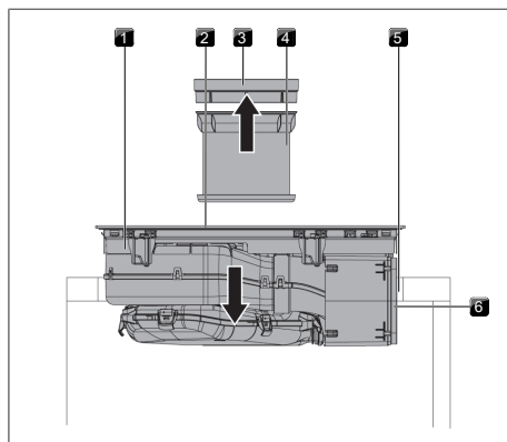
Bild 9.28 Placera spishällen centrerat
