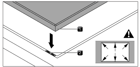
Bild 9.14 Höjdtjämningsplattornas positionering
