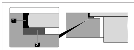
Bild 9.11 Tätningsband vid planmontering
