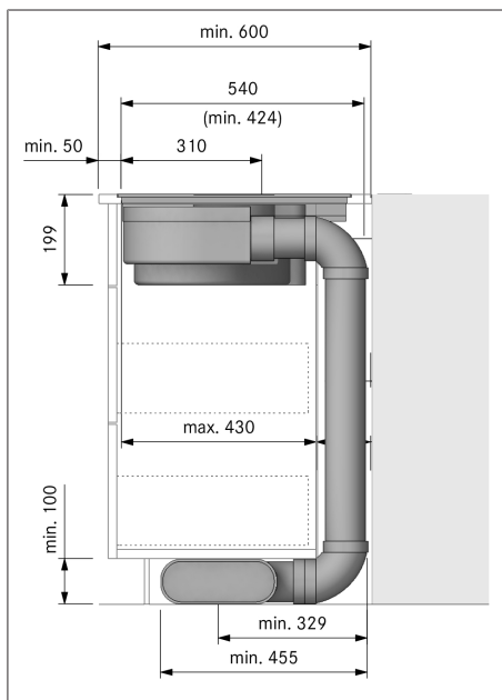
Bild 9.9 Inbyggnadsmått frånluft, bänkskivans djup 600 mm
