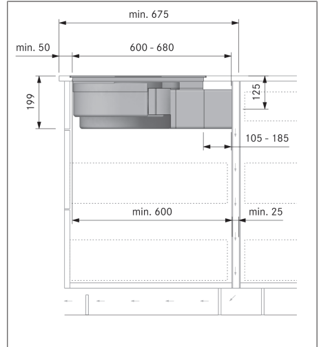
Bild 9.26 Inbyggnadsmått vid luftcirkulation monteringsvariant A, bänkskivans djup från 675 mm
