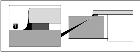
Bild 9.42 Silikontätningssmassa vid ytmontering
